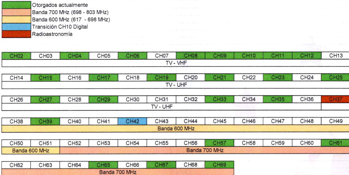
Figura No. 02 – Distribución actual de Canales de Televisión
