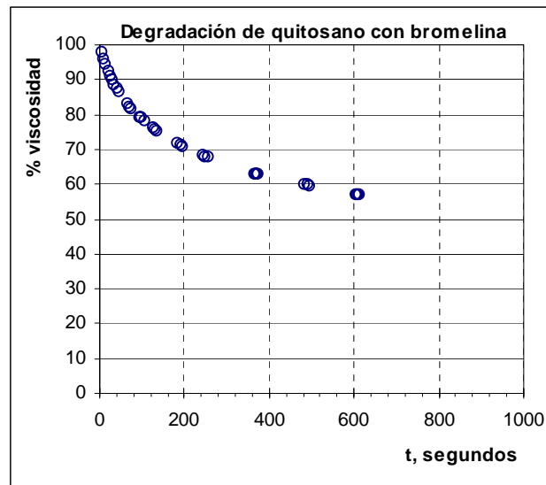
Fig. 5.- Resultados de los estudios preliminares en la depolimerización del quitosano con bromelina en soluciones acuosas a 25 °C.
