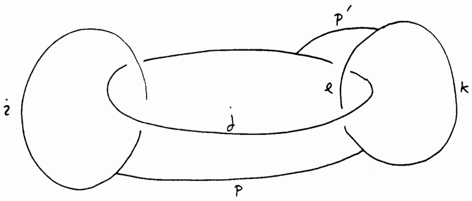
Graph used to prove Sa = bS
