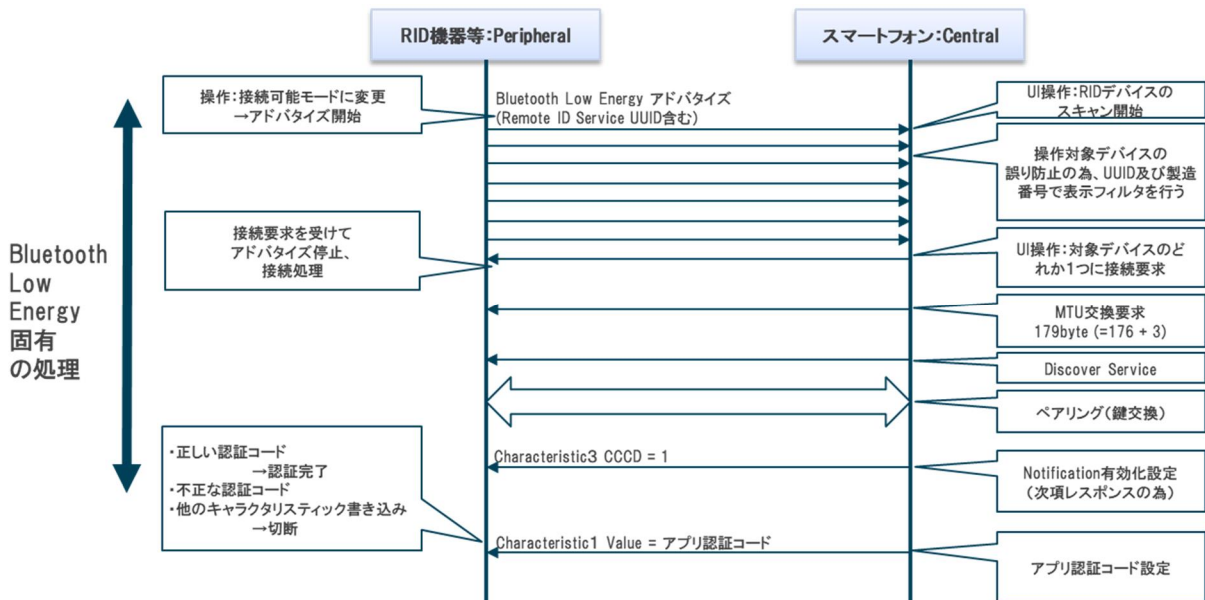
図 1 RID 機器等への接続処理シーケンス
