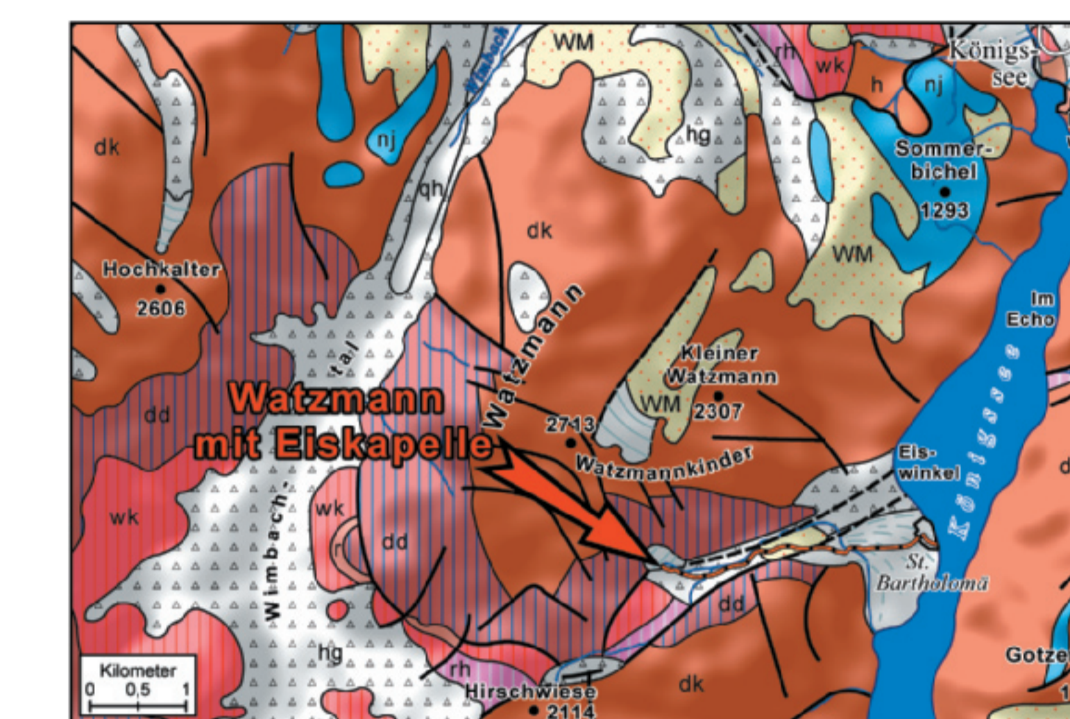
Geologische Karte der Umgebung des Watzmanns
