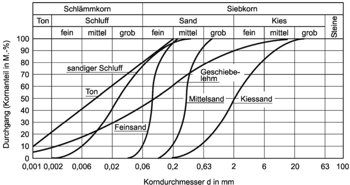
6-31 Kornverteilungslinien
