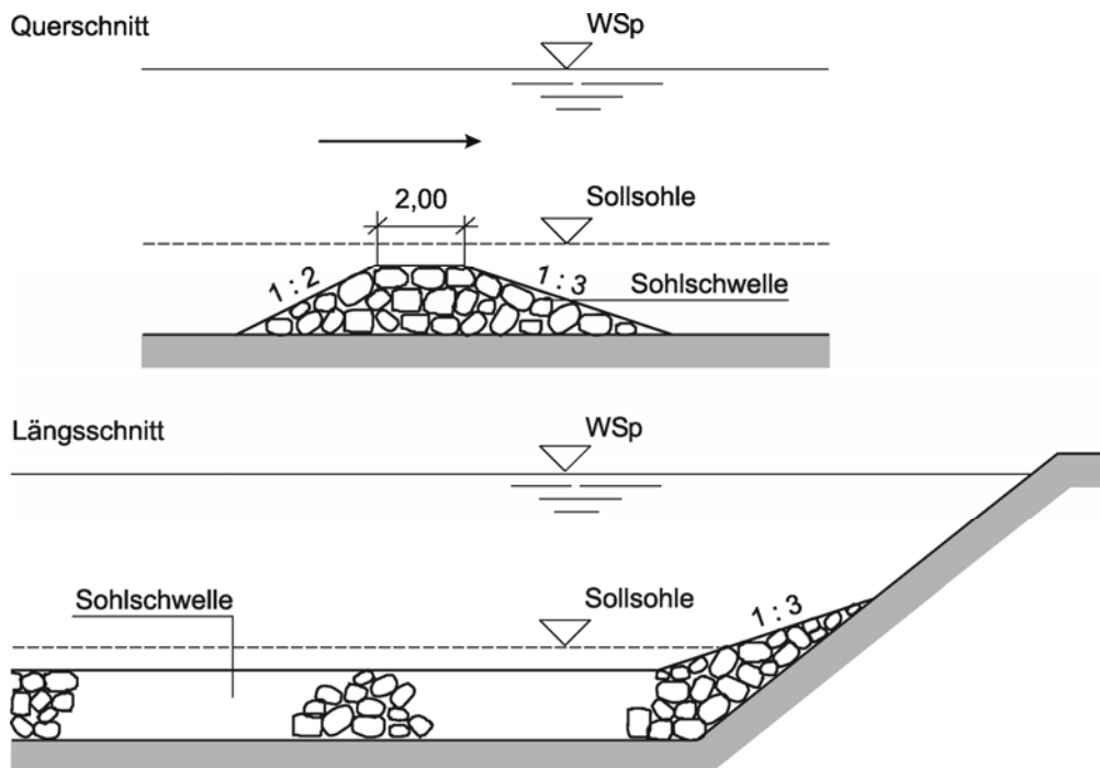
12-14 Sohlschwelle
