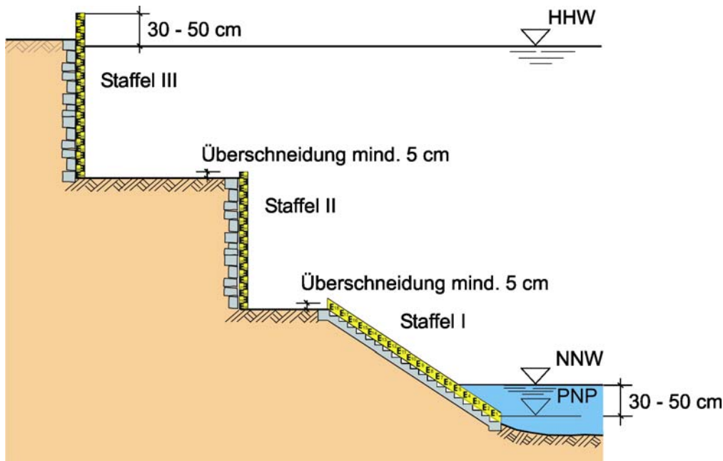
10-8 Pegelstaffel
