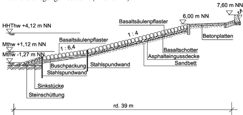
19-11 Schrägdeckwerk auf Norderney (nach Unterlagen des Niedersächsischen Landesbetriebes für Wasserwirtschaft, Küsten- und Naturschutz (NLWKN))
