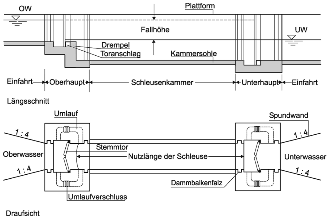
16-11 Längsschnitt und Draufsicht einer Schleuse
