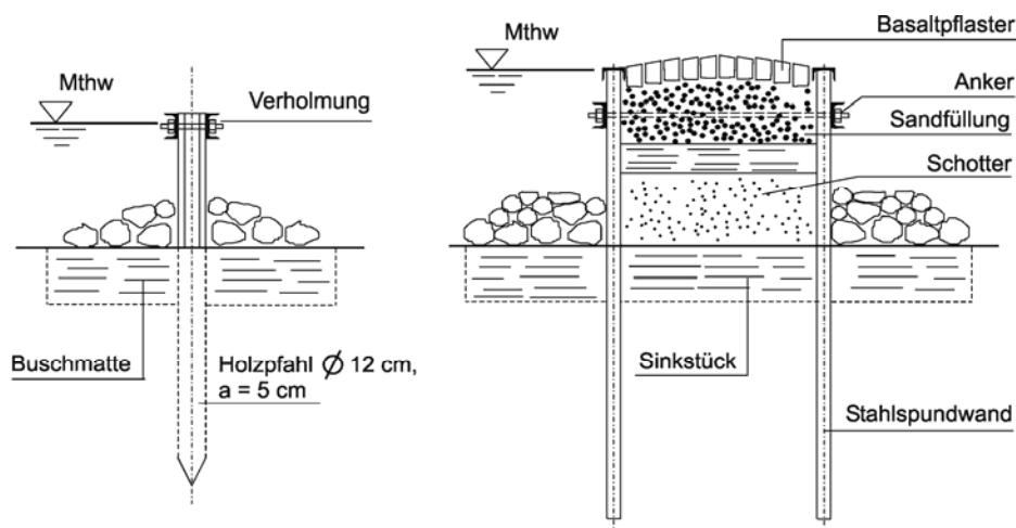
19-13 Einreihige Pfahlbuhne (Querschnitt)
