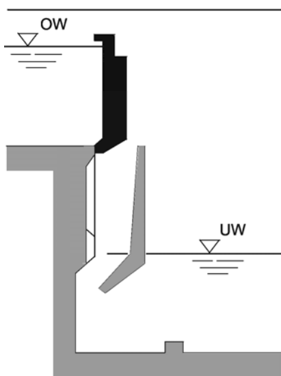
Senktor
