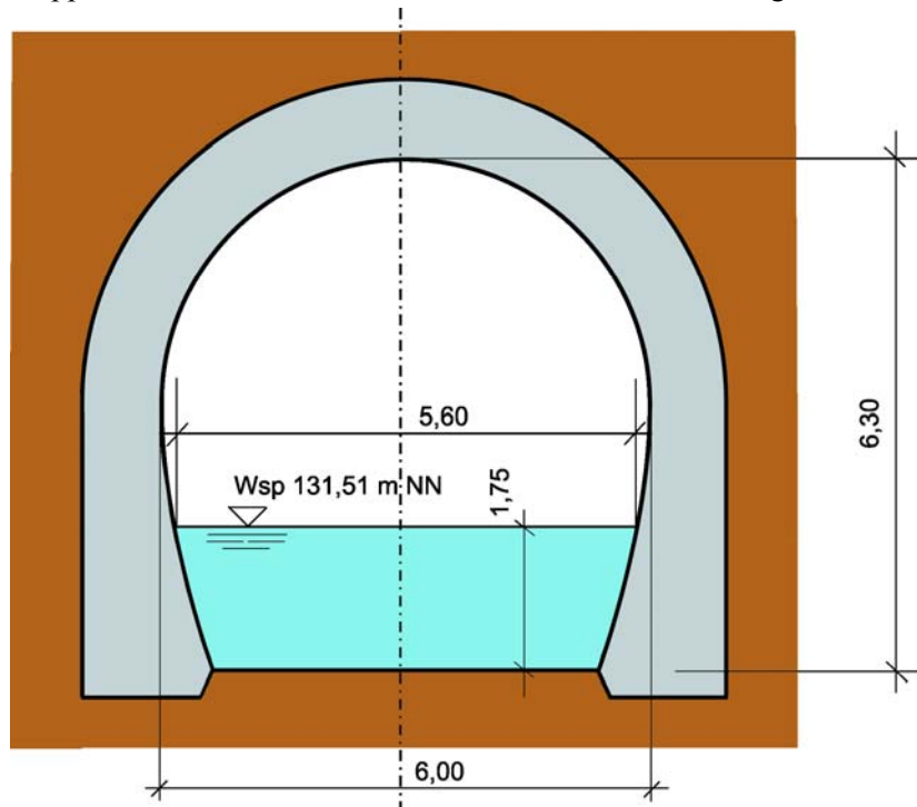
16-25 Schiffahrtstunnel bei Weilburg/Lahn
