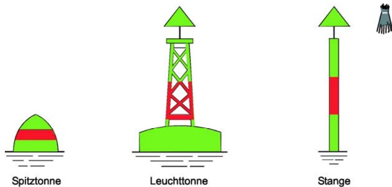
Steuerbordseite des durchgehenden Fahrwassers/Backbordseite des abzweigenden oder einmündenden Fahrwassers
