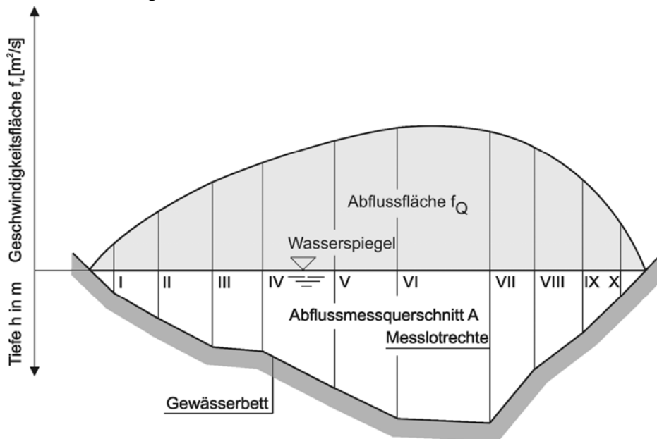
10-19 Ermittlung des Abflusses
