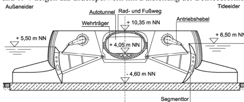
19-6 Eidersperrwerk (Querschnitt)
