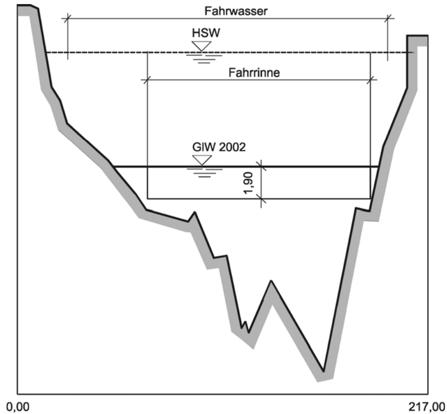
13-2 Fahrrinne und Fahrwasser (Querprofil bei Rhein-km 553,400 (Überhöhte Darstellung))
