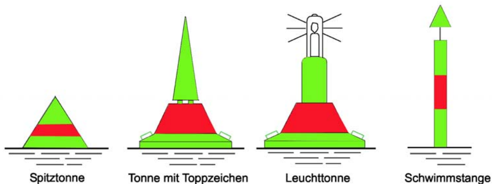
Linke Seite der durchgehenden Fahrrinne/rechte Seite der abzweigenden oder einmündenden Fahrrinne
