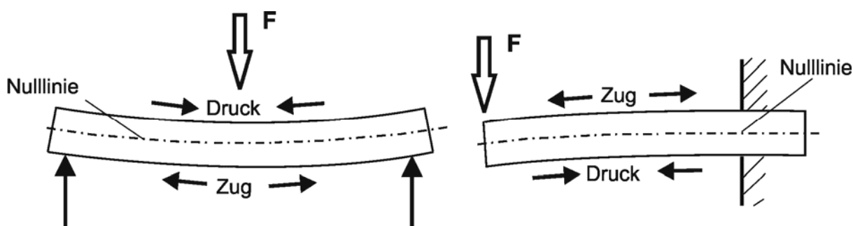
6-22 Balken auf zwei Stützen
