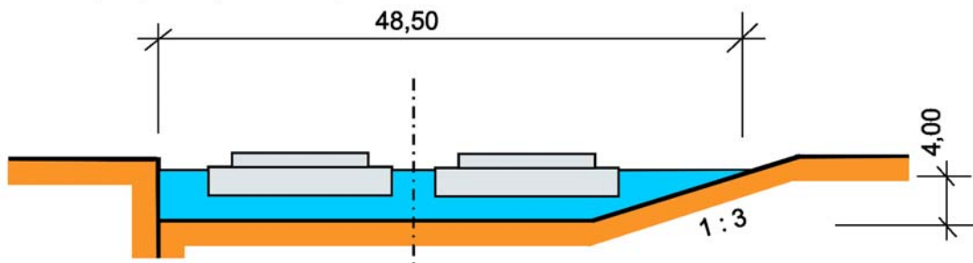
Rechtecktrapezprofil (RT-Profil)
