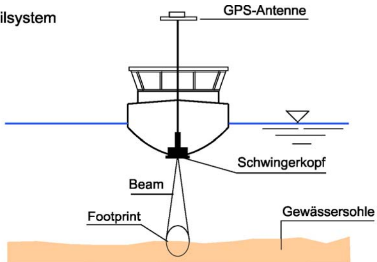
Auslegersystem
