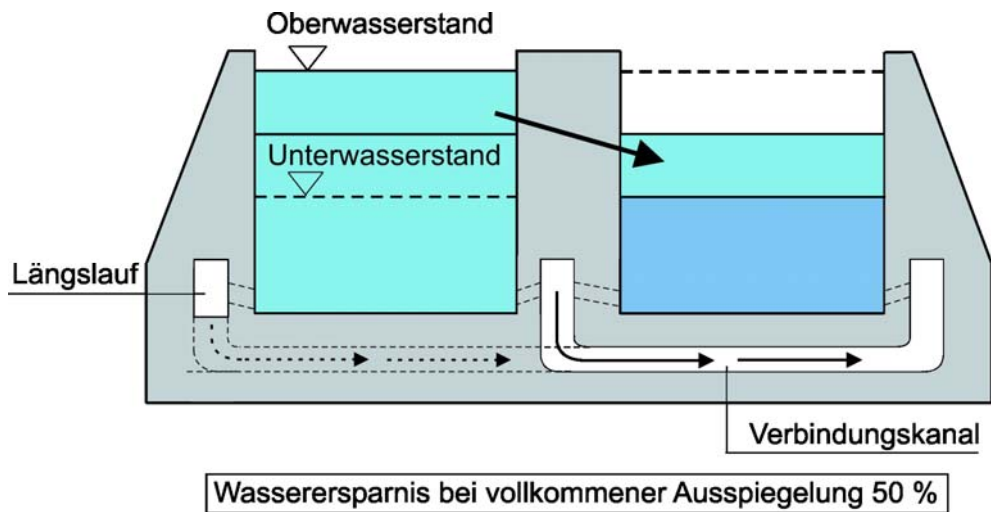
16-13 Zwillingschleuse
