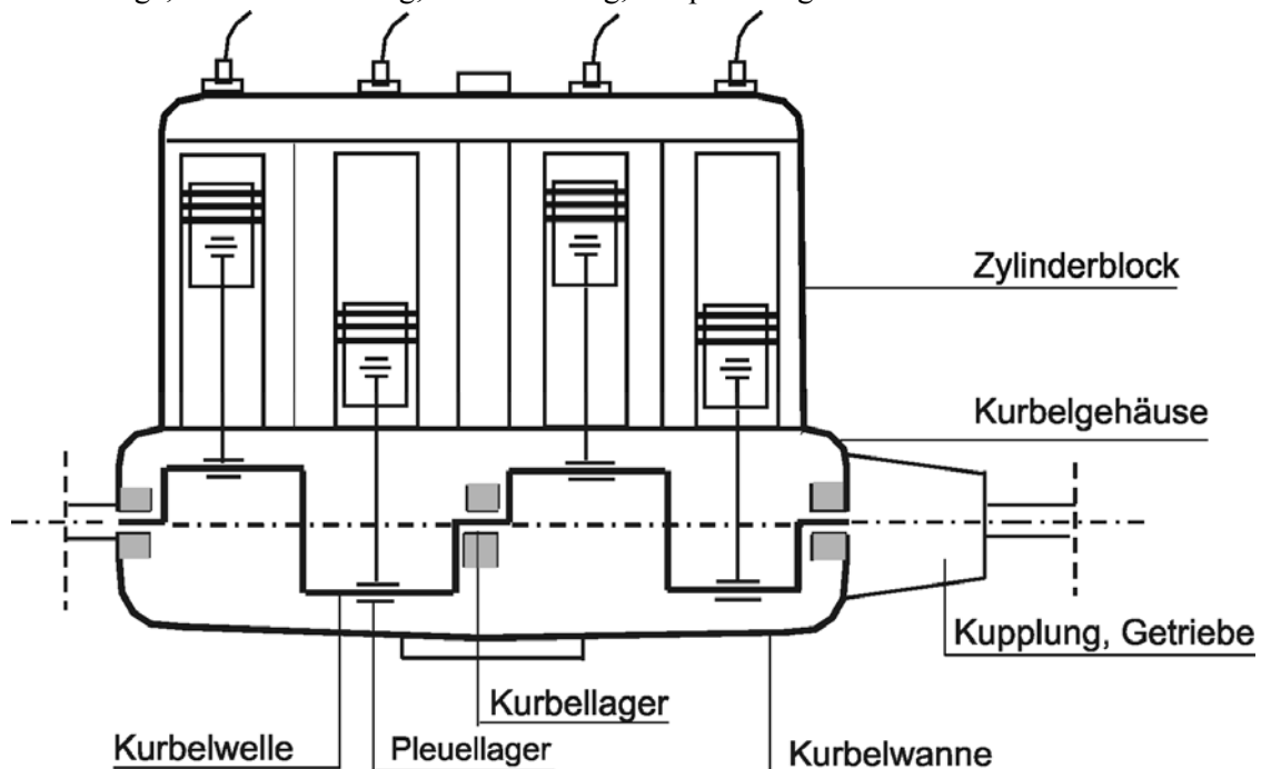
7-2 Otto-Viertaktmotor
