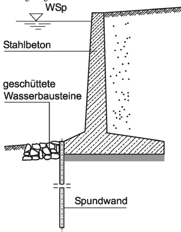
15-37 Winkelstützmauer
