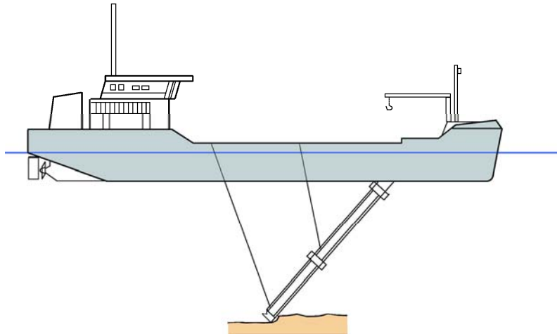
14-5 Hopperbagger (Laderaumsaugbagger)
