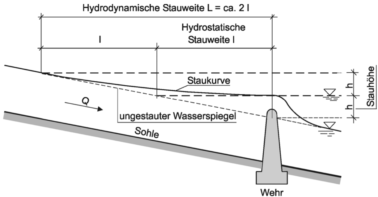
12-16 Staubereich einer Stauhaltung
