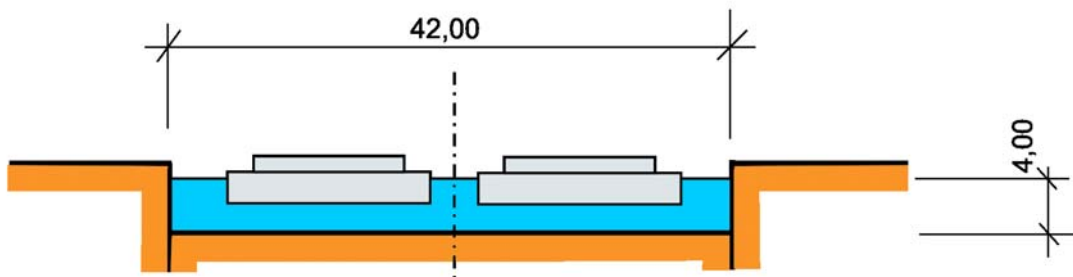
Rechteckprofil (R-Profil)
