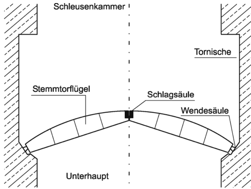
16-16 Stemmtor (Draufsicht)
