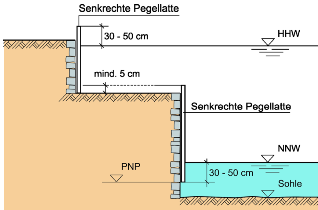
10-3 Lage des Pegelnullpunktes
