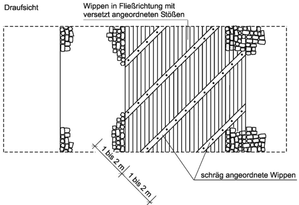
15-15 Faschinenmatte
