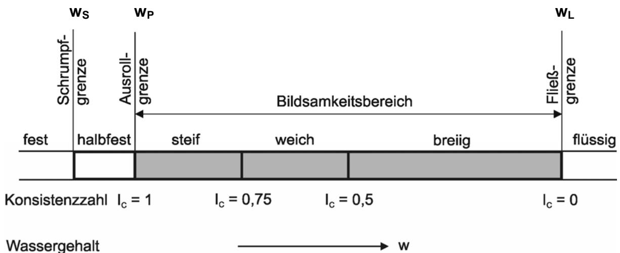
6-32 Konsistenzbalken nach Atterberg
