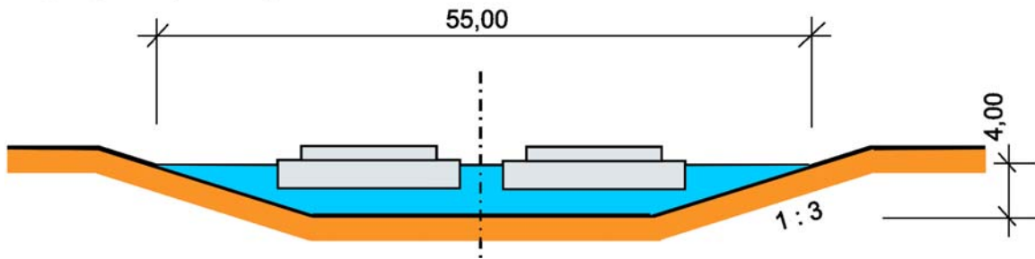
Trapezprofil (T-Profil)
