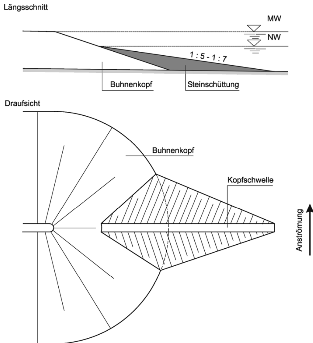
12-12 Kopfschwelle
