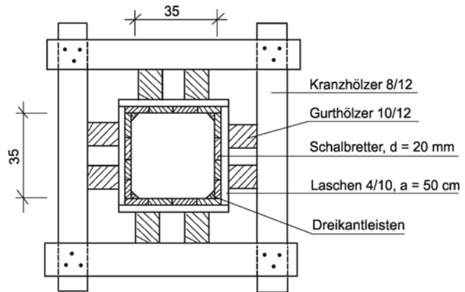
6-20 Schalung für eine Stahlbetonstütze (Querschnitt)
