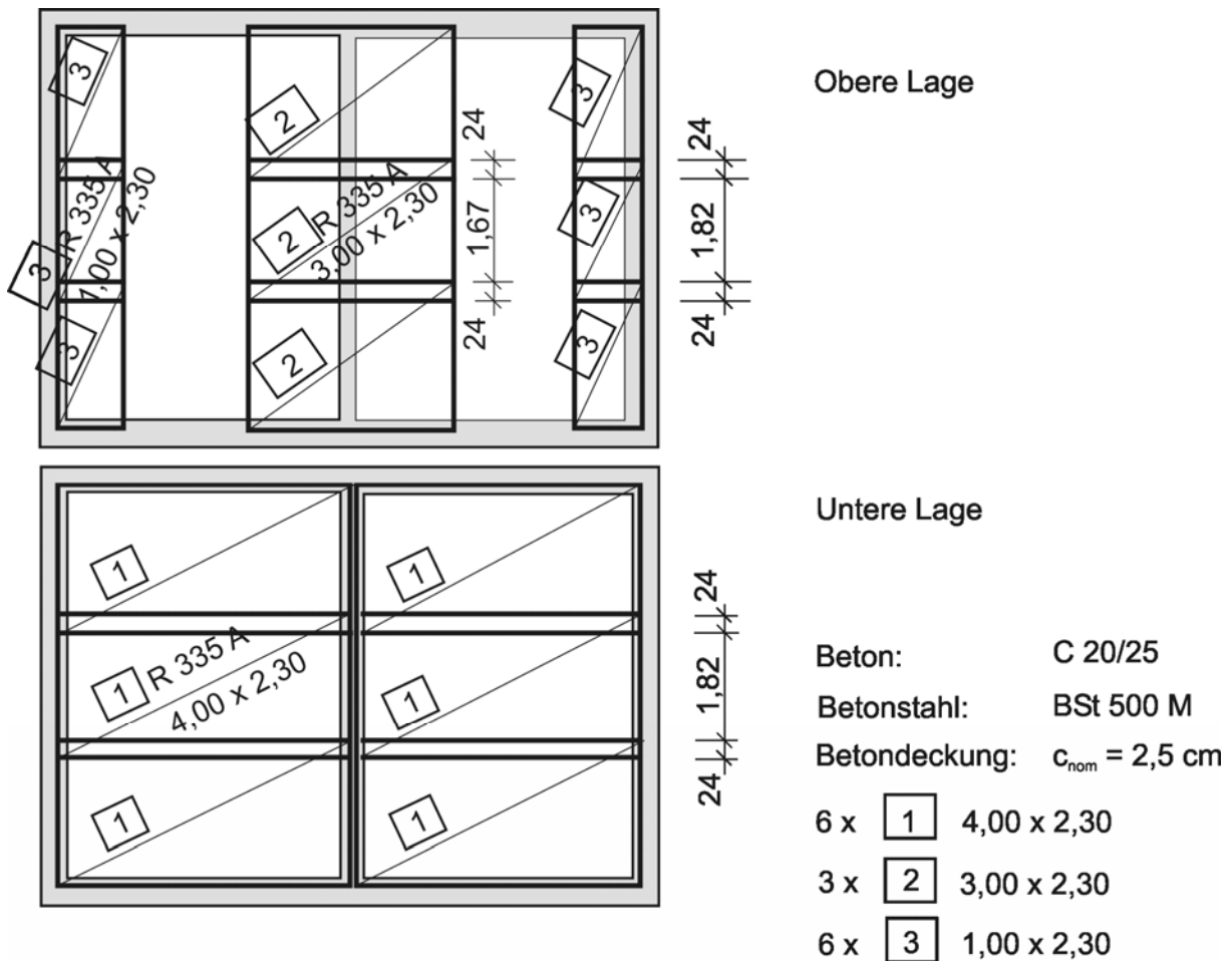
6-27 Deckenbewehrung
