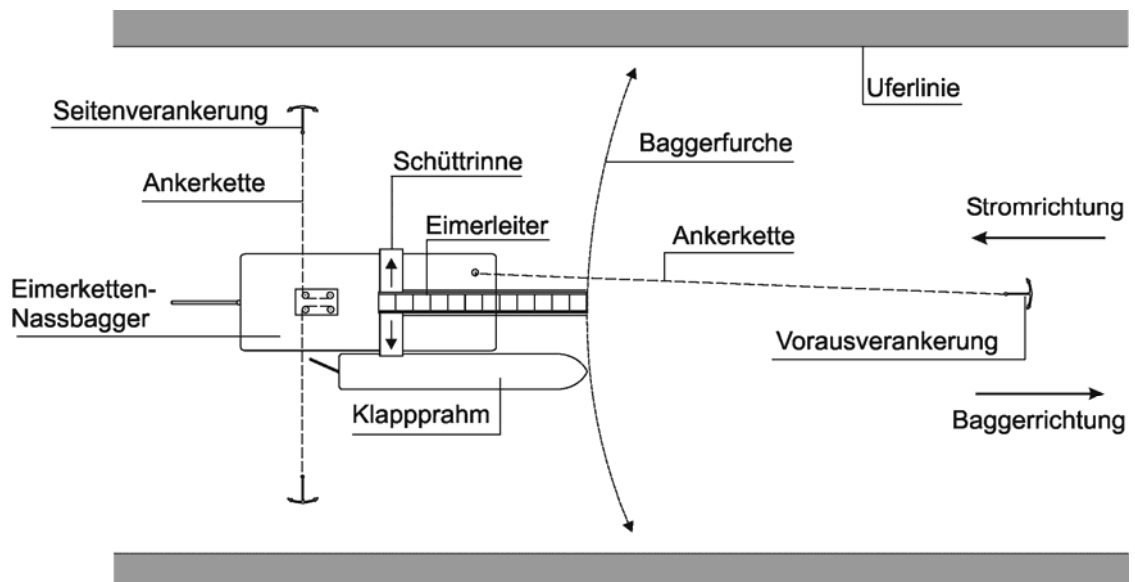
14-4 Arbeitsweise des Eimerketten-Nassbaggers
