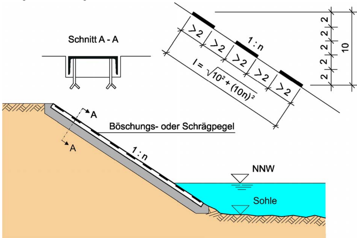
10-6 Böschungs- oder Schrägpegel
