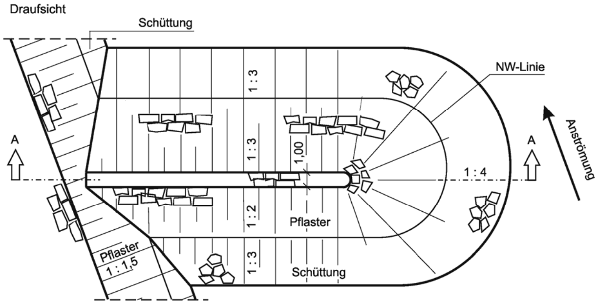
12-6 inklinante Steinbühne
