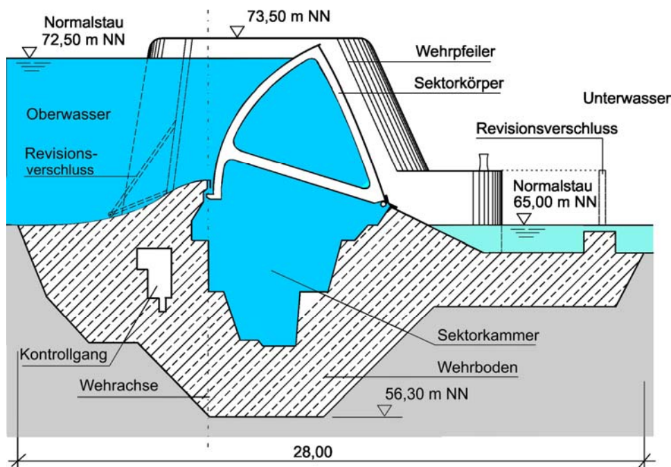
16-5 Sektorwehr Lehmen/Mosel (Inbetriebnahme 1965)
