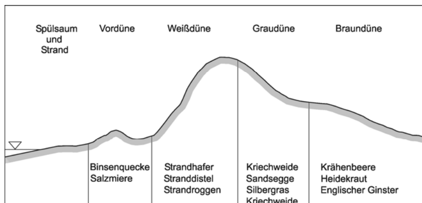
19-10 Schematischer Querschnitt der Dünen der Nordsee und ihr Pflanzenbewuchs (LKN-SH)
