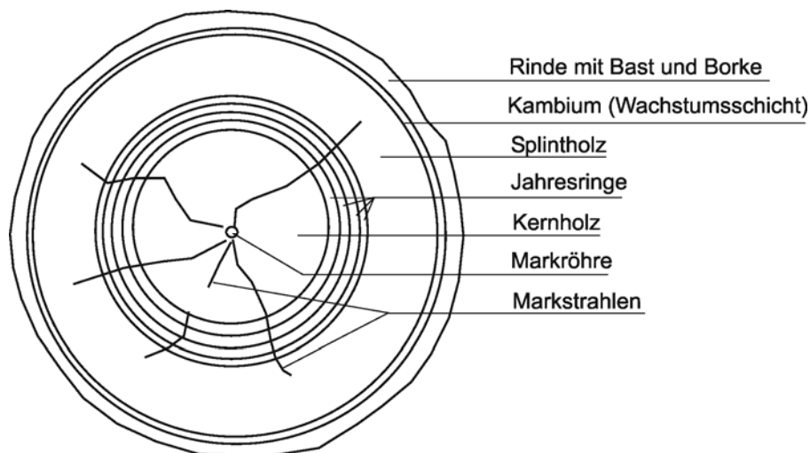
6-33 Aufbau des Holzes (Querschnitt)
