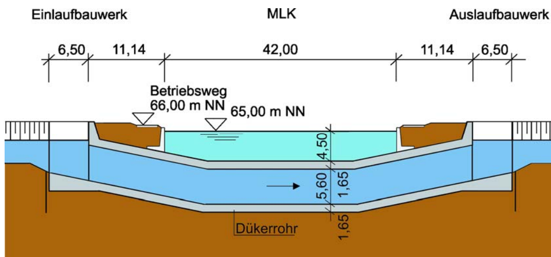
16-29 Längsschnitt eines Dükers unter dem Mittellandkanal
