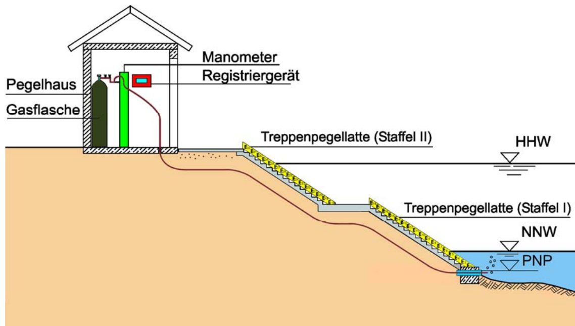
10-10 Druckluftpegel (Einperlmethode)
