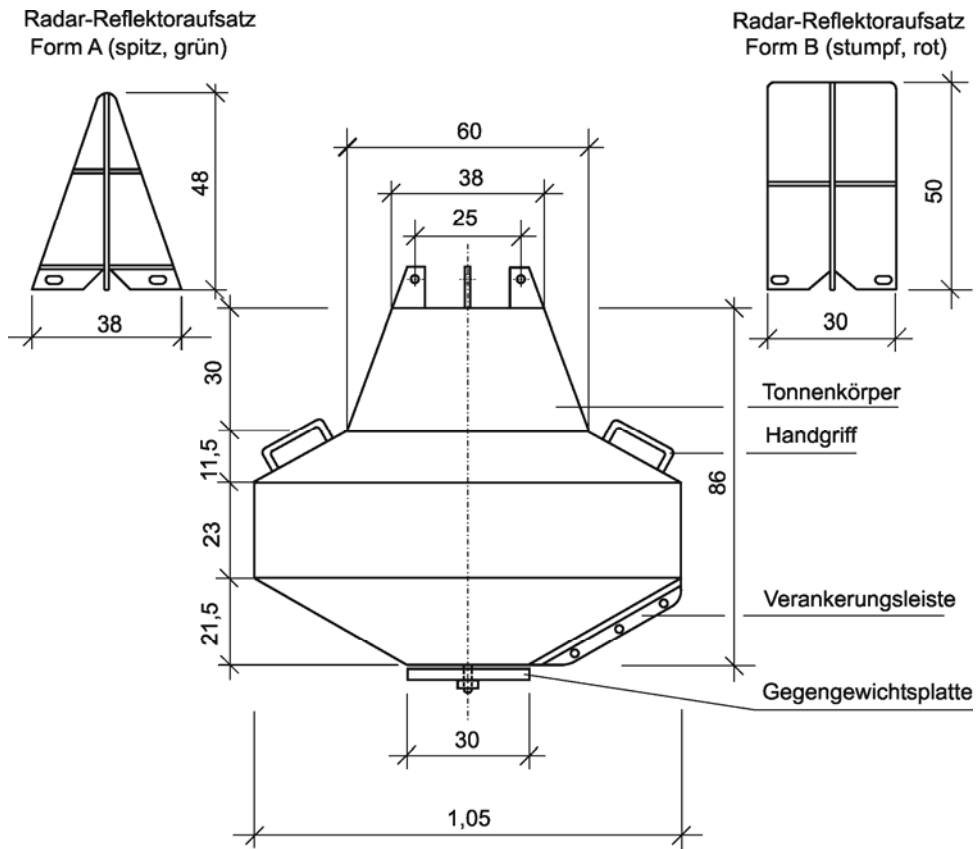
13-4 Einheitstonne
