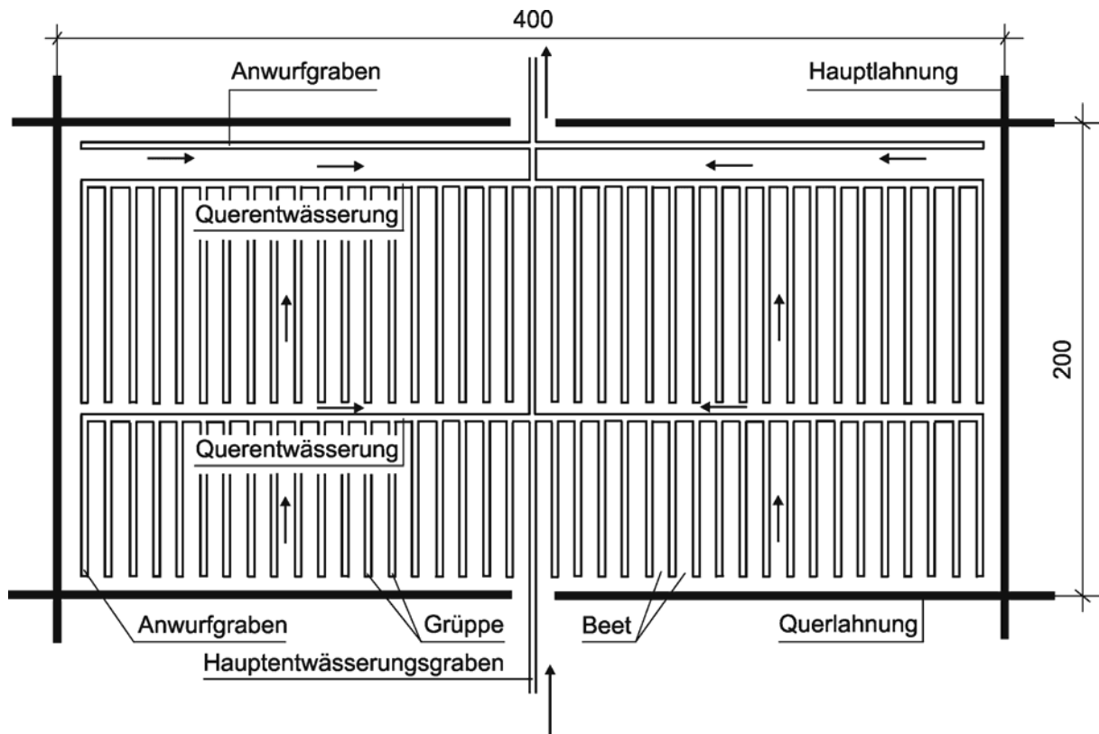
19-17 Lahnungsfeld
