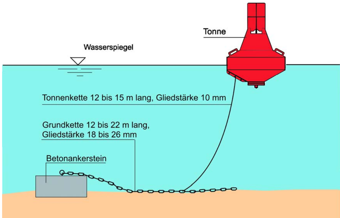
13-5 Tonnenverankerung auf kiesiger Flusssohle in schnell strömenden Gewässern
