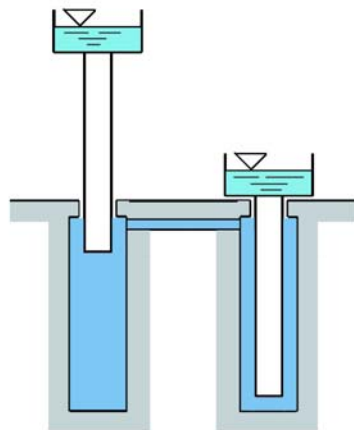
Presskolbenhebwerk
