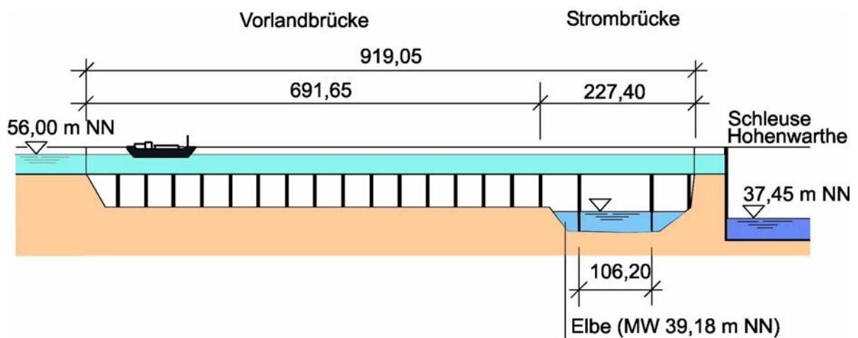
16-23 Längsschnitt der Kanalbrücke Magdeburg (überhöhte Darstellung)
