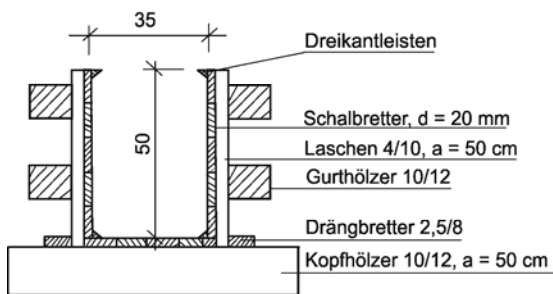
6-19 Schalung für einen Stahlbetonbalken (Querschnitt)
