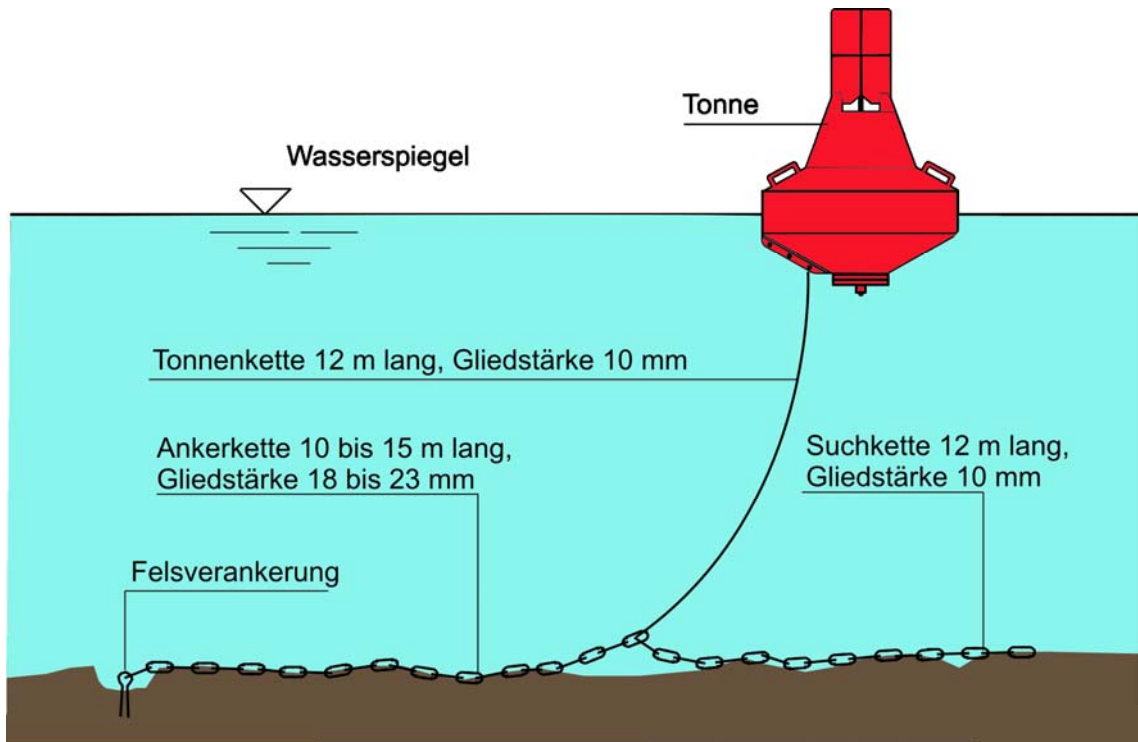
13-6 Tonnenverankerung auf felsiger Flusssohle
