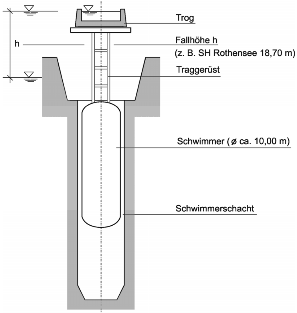
16-20 Schwimmerhebewerk (Querschnitt) - Schraubenspindeln zum Antrieb nicht dargestellt -
