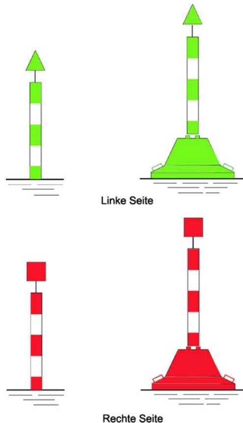
13-10 Schwimmende Zeichen zur Bezeichnung von Hindernissen
