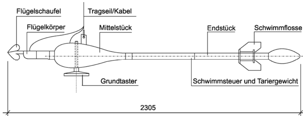
10-16 Messflügel in Schwimmflügelausrüstung (Ott-Schwimmflügel mit 100 kg-Mittelstück)
