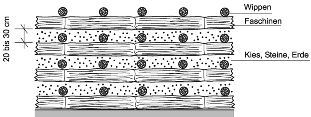
15-16 Packfaschinat
