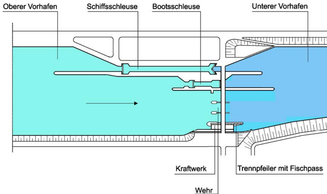
12-17 Bauwerke einer Staustufe
