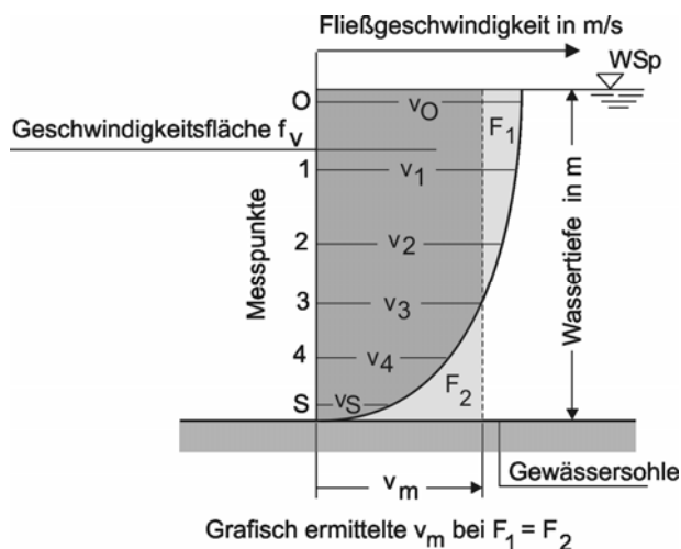
10-17 Geschwindigkeitsverteilung in einer Messlotrechten
