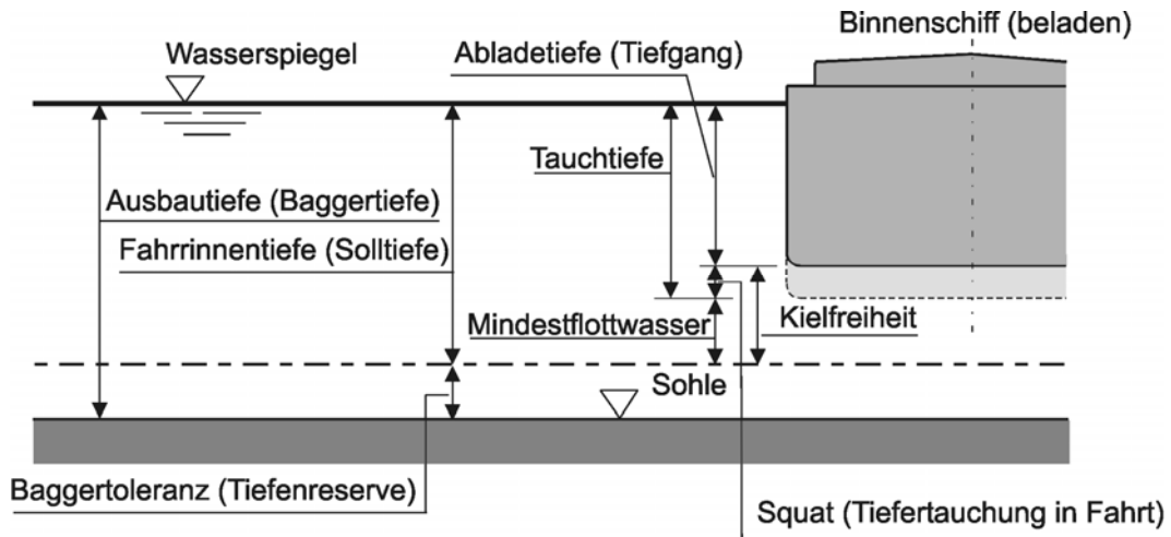
13-1 Schiff und Fahrrinne
