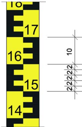
10-4 Maßeinteilung einer senkrechten Pegellatte
