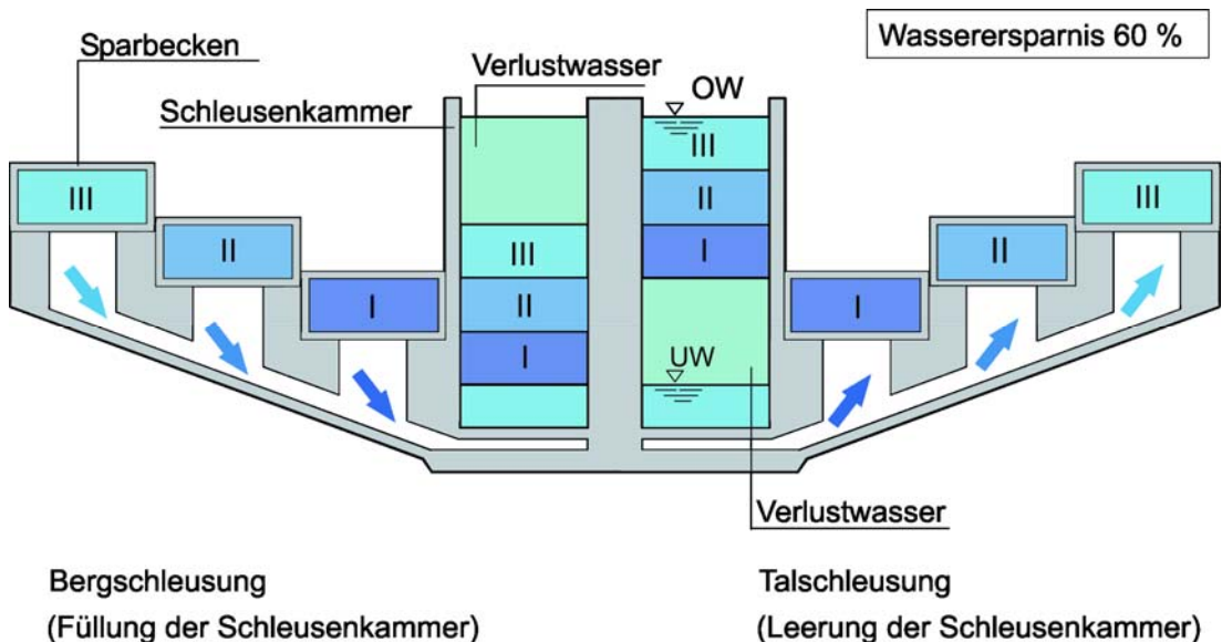
16-14 Schematischer Querschnitt einer Doppelschleuse mit Sparbecken
