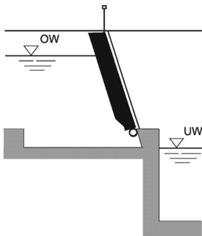
Klapptor
