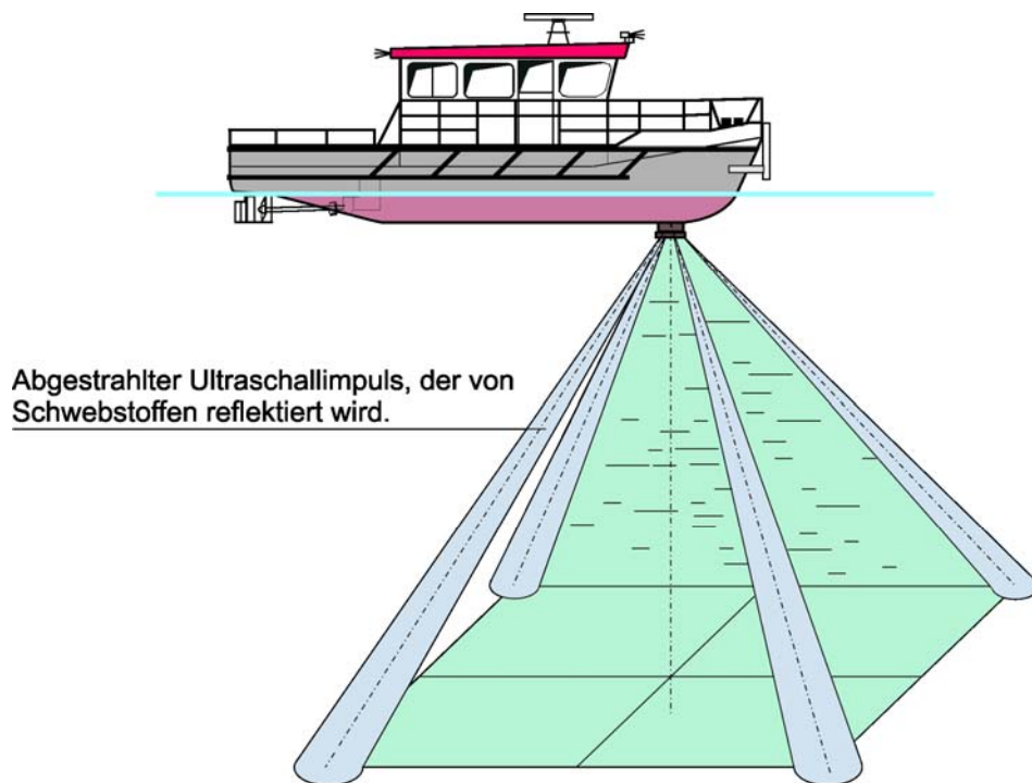
10-21 ADCP-Messprinzip
