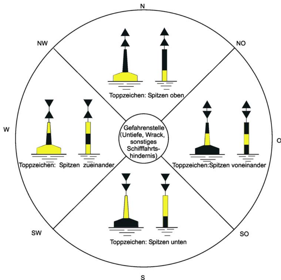
13-11 Kardinalzeichen
