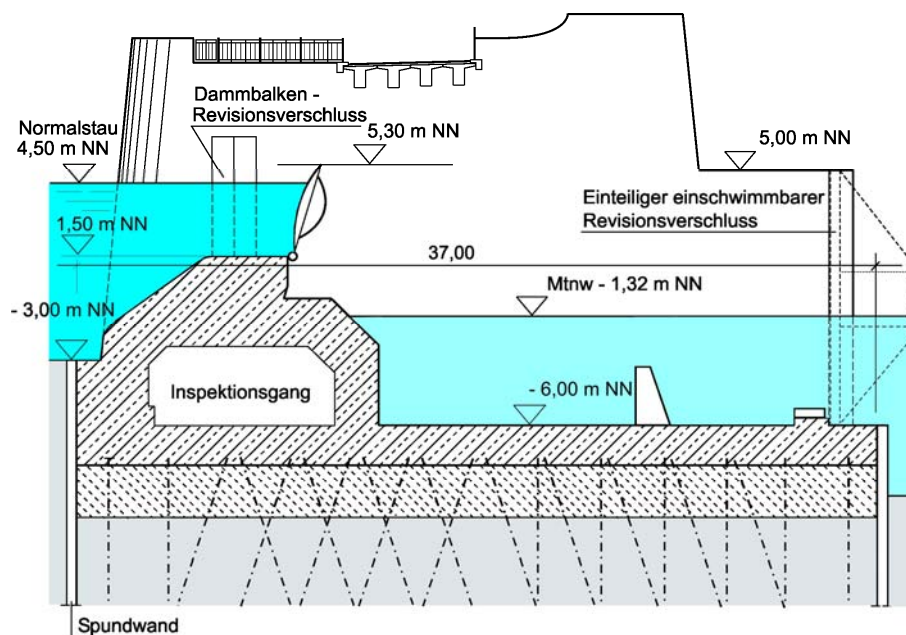
16-4 Klappenwehr in Bremen/Weser (Inbetriebnahme 1993)
