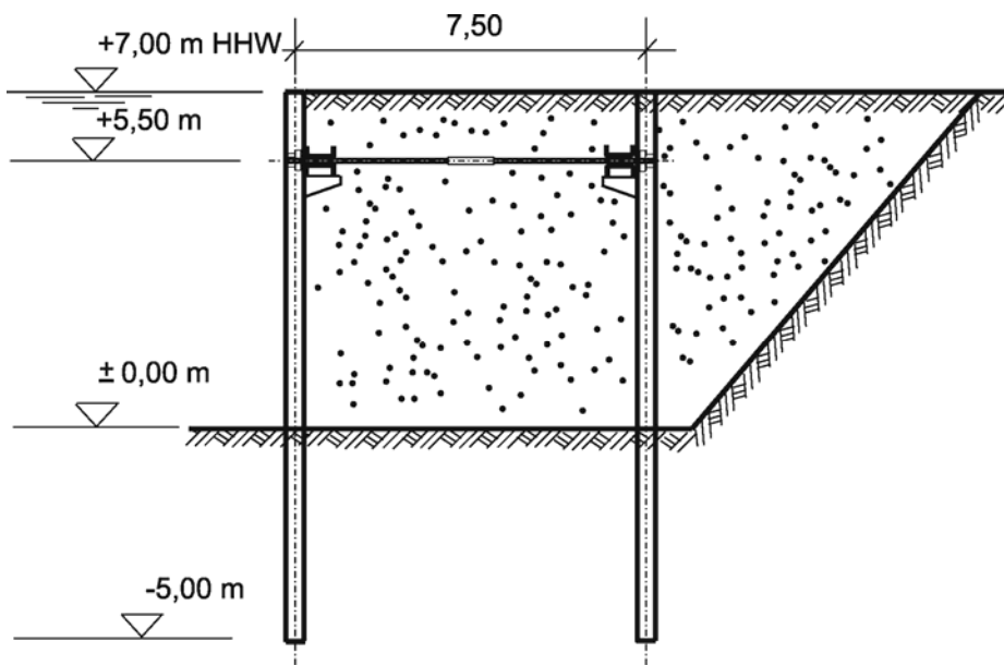
15-35 Querschnitt eines Kastenfangedammes
