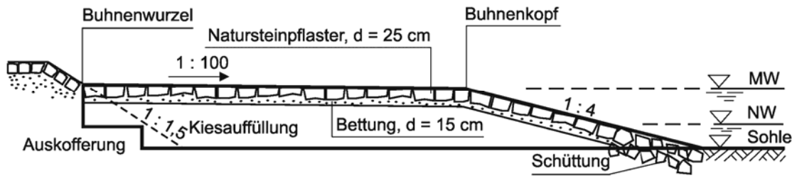
Längsschnitt A - A
