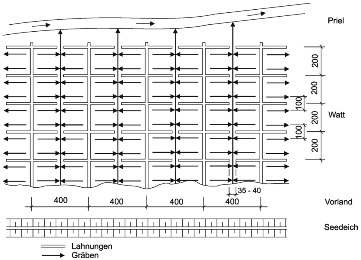
19-16 Lahnungssystem
