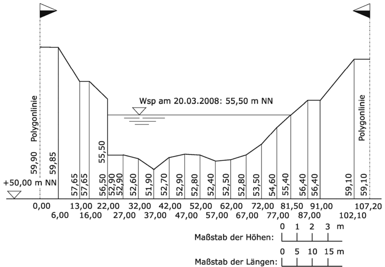
9-3 Querprofil bei Fluss-km 65,4
