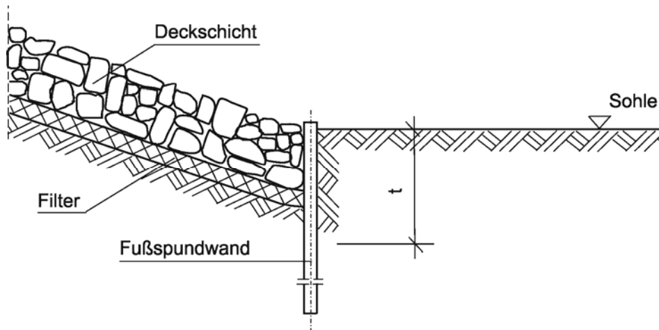
15-30 Fußspundwand
