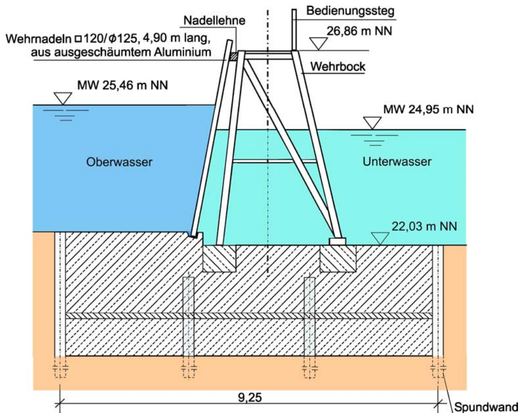
16-9 Nadelwehr Grütz/Untere Havel-Wasserstraße (Inbetriebnahme 2003; Ersatz eines Nadelwehres, Baujahr 1910)
