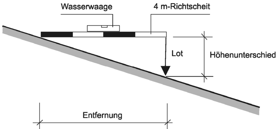
8-6 Staffelmessung
