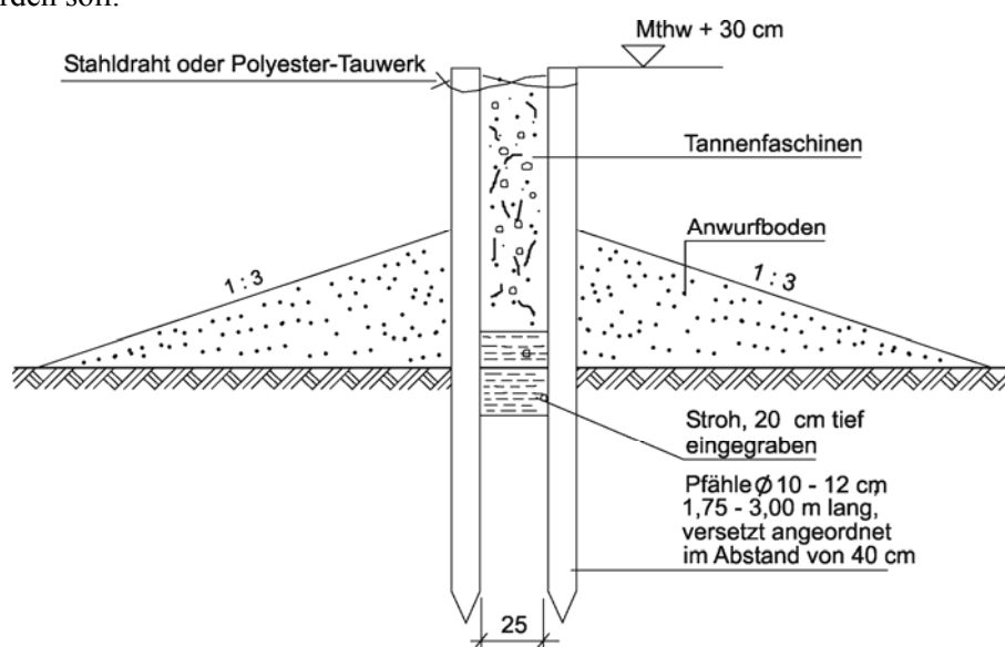
19-15 Lahnung (Querschnitt)
