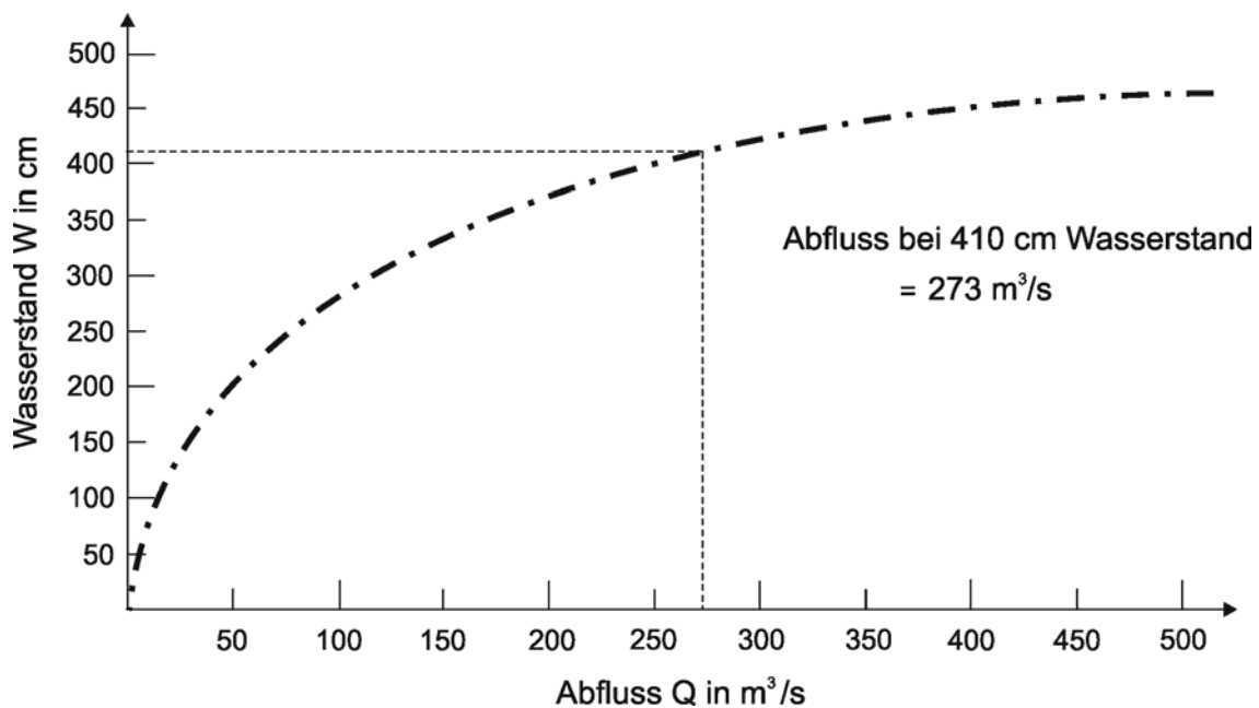
10-15 Abflusskurve
