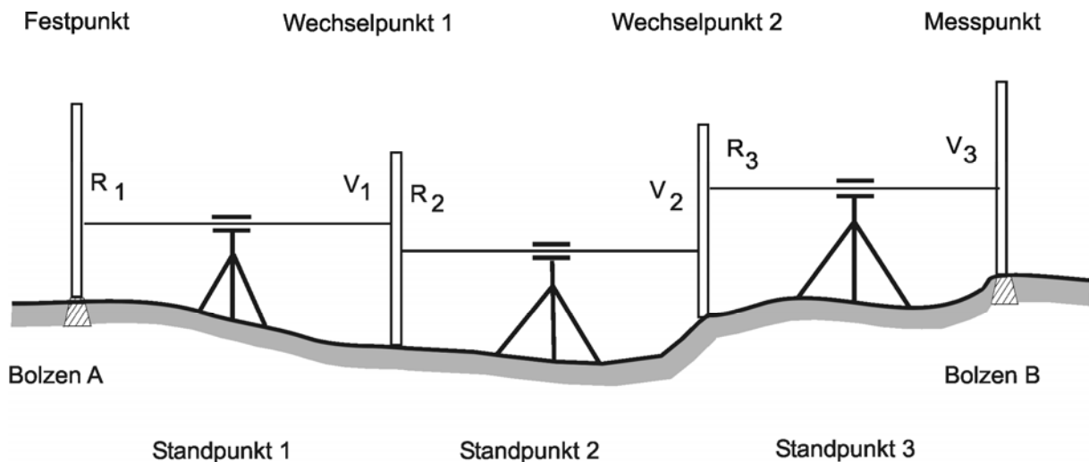
8-8 Liniennivellement
