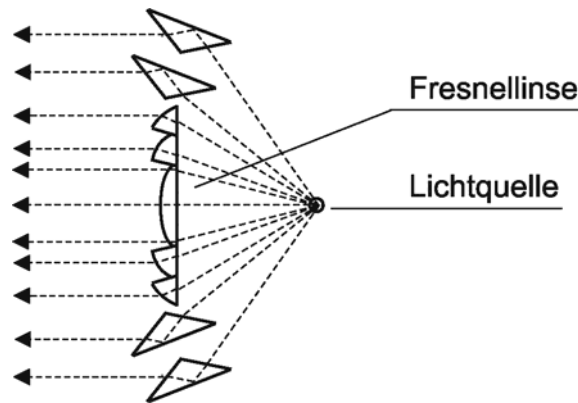
13-23 Fresnel-Linsensystem
