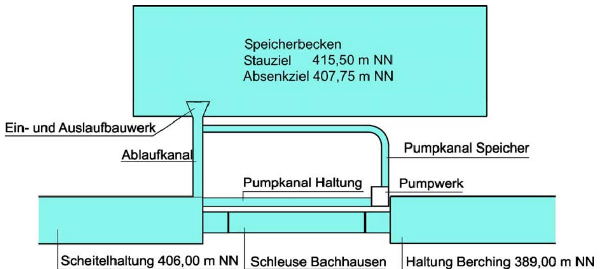
17-2 Draufsicht des Dürrlohspeichers am Main-Donau-Kanal (Schematische Darstellung)
