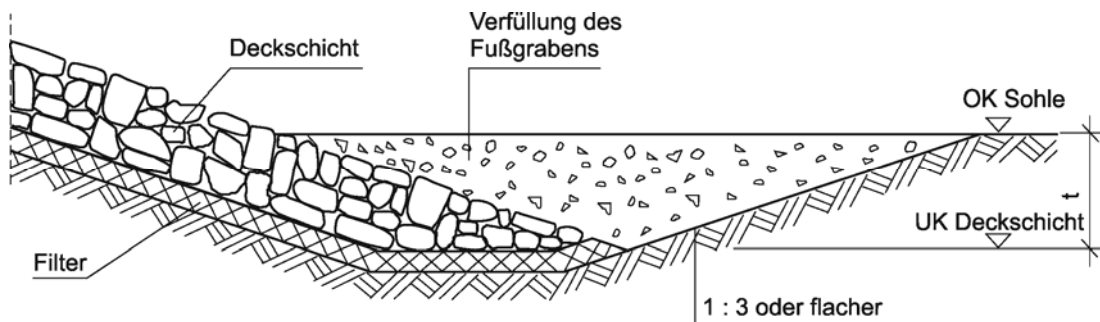
15-28 Fußeinbindung (Fußverlängerung)
