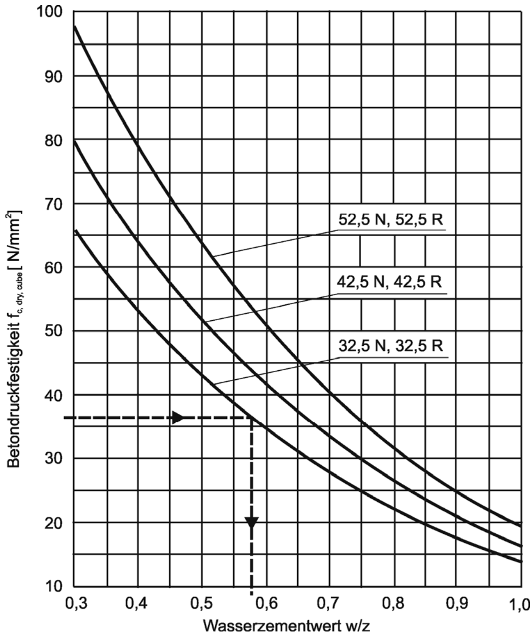
6-12 Zusammenhang zwischen Betondruckfestigkeit, Festigkeitsklasse des Zements und Wasserzementwert (Walz-Diagramm) Erläuterung zum Diagramm: Die Betondruckfestigkeitswerte beziehen sich auf trocken gelagerte Probewürfel.
