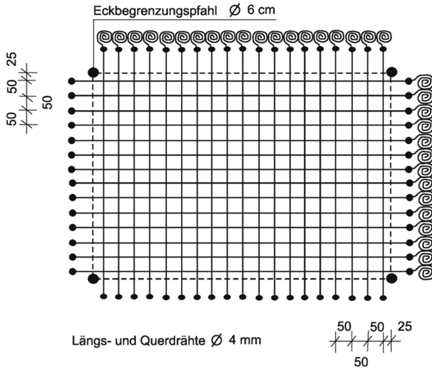
15-14 Herstellung der Buschmatte (Draufsicht auf den Drahtrost)
