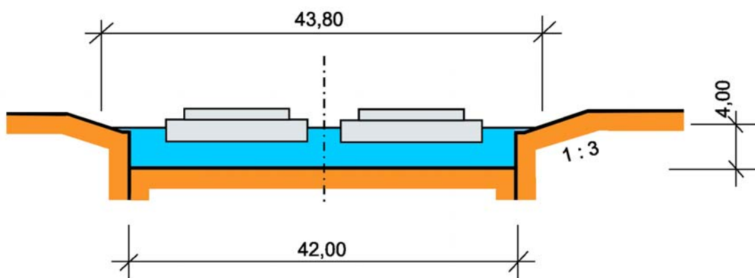
Kombiniertes Rechtecktrapezprofil (KRT-Profil)
