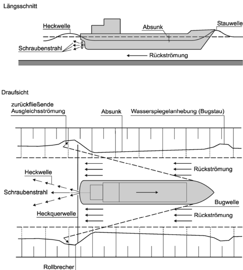
13-2 Hydraulische Belastung einer Böschung durch das fahrende Schiff
