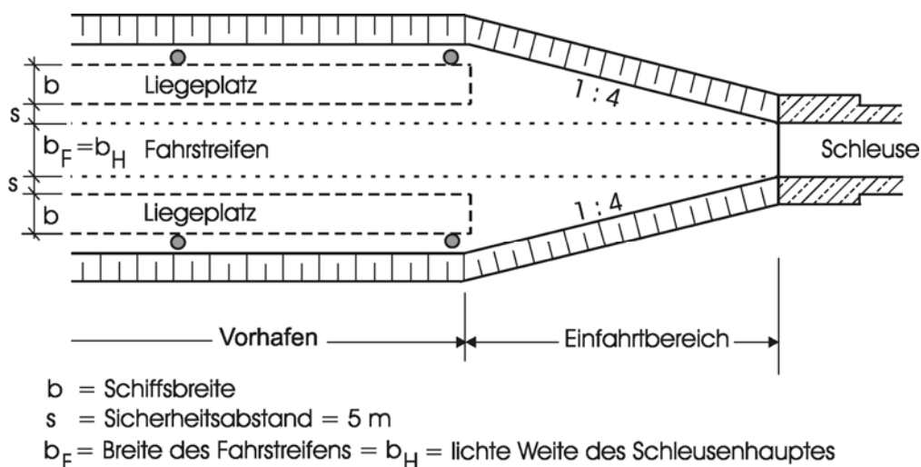
16-18 Schleusenvorhafen
