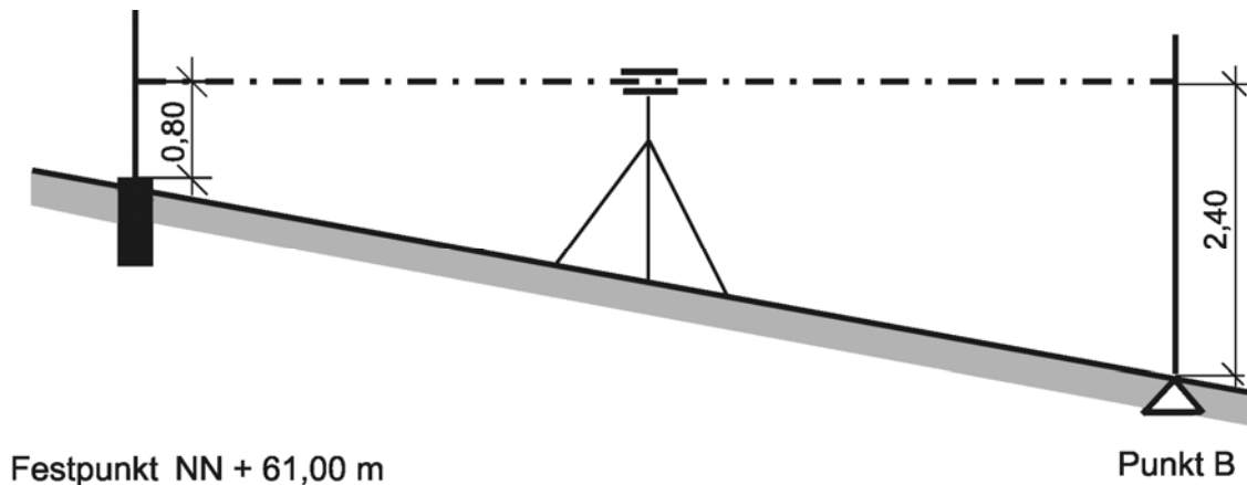
8-4 Messung des Höhenunterschieds zwischen zwei Punkten
