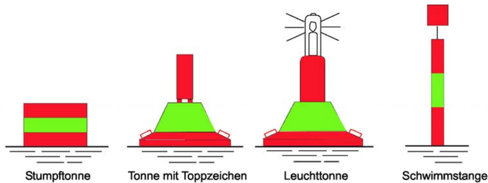
Rechte Seite der durchgehenden Fahrrinne/linke Seite der abzweigenden oder einmündenden Fahrrinne
