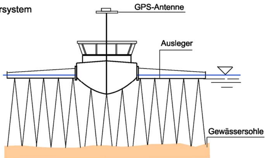
Fächerecholot
