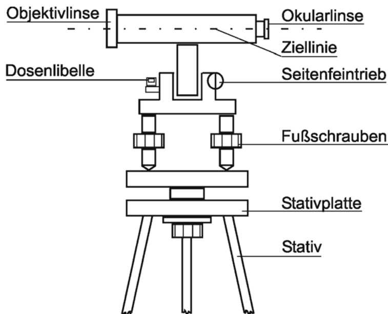
8-1 Automatisches Nivelliergerät
