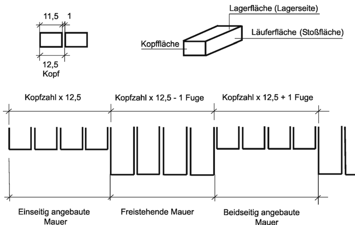
6-7 Schema für die Berechnung der Mauerlängen
