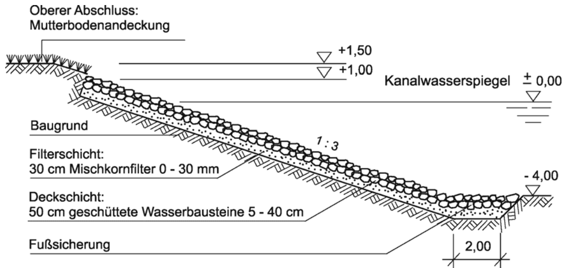
15-20 Durchlässiges Uferdeckwerk
