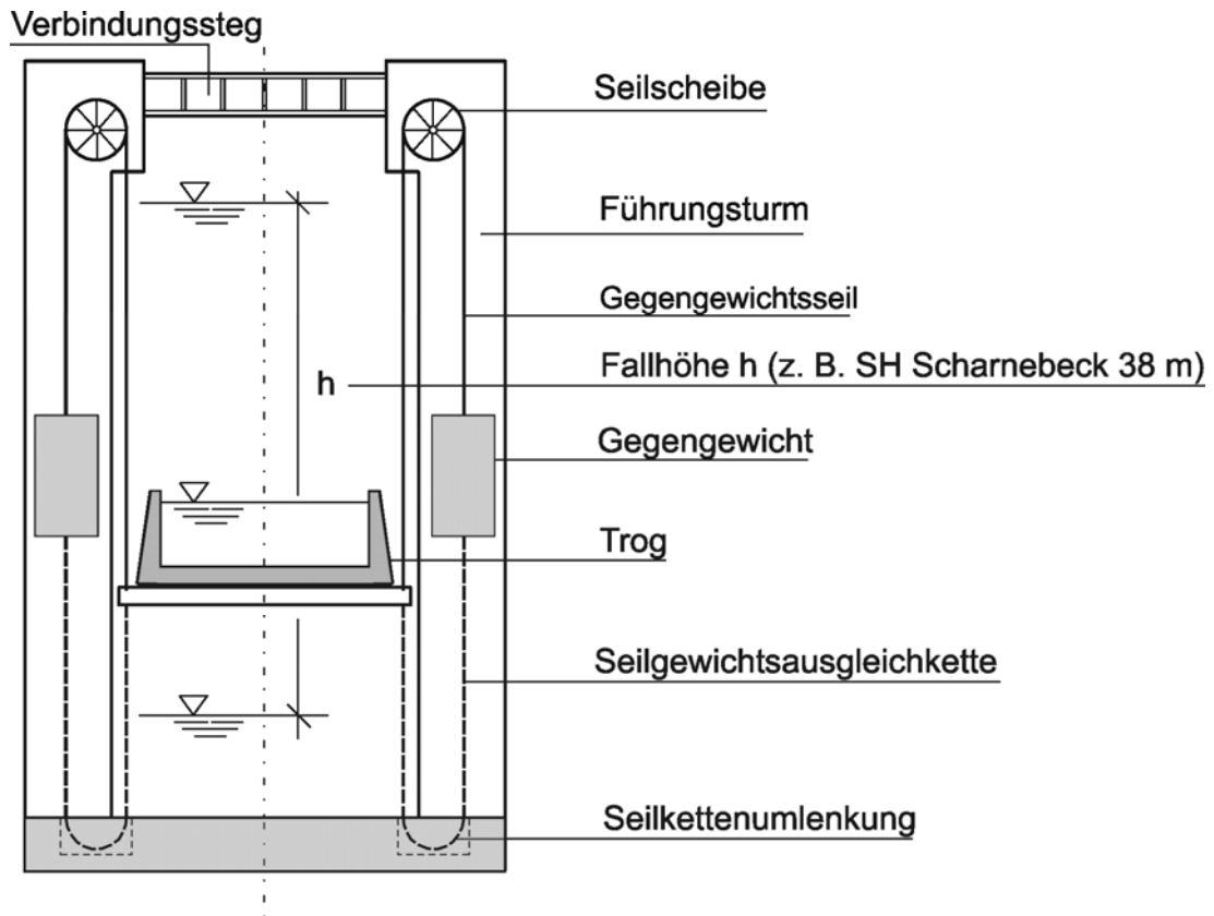
16-21 Gegengewichtshebewerk (Querschnitt) - Antriebs-elemente (Spindeln, Zahnstangen) nicht dargestellt -
