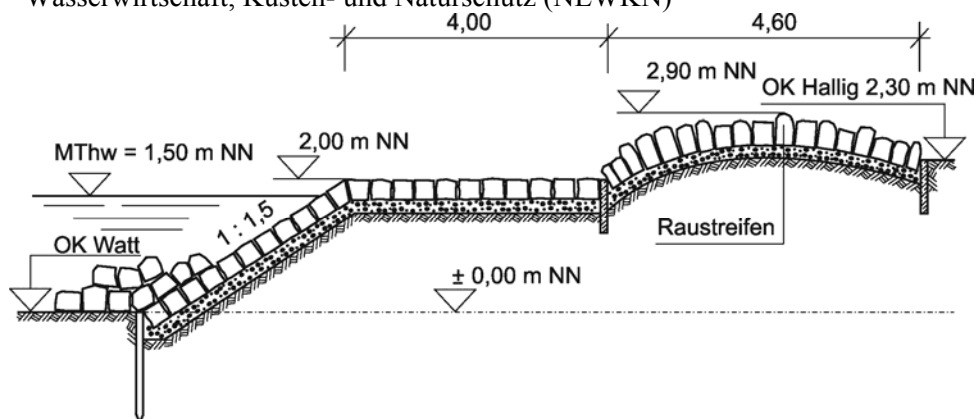
19-12 Deckwerk einer Hallig mit Raustreifen (Igel)
