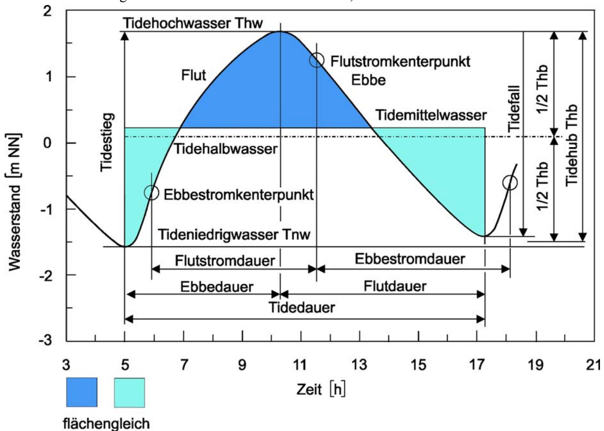
19-1 Tidekurve der deutschen Nordsee nach DIN 4049 Teil 3
