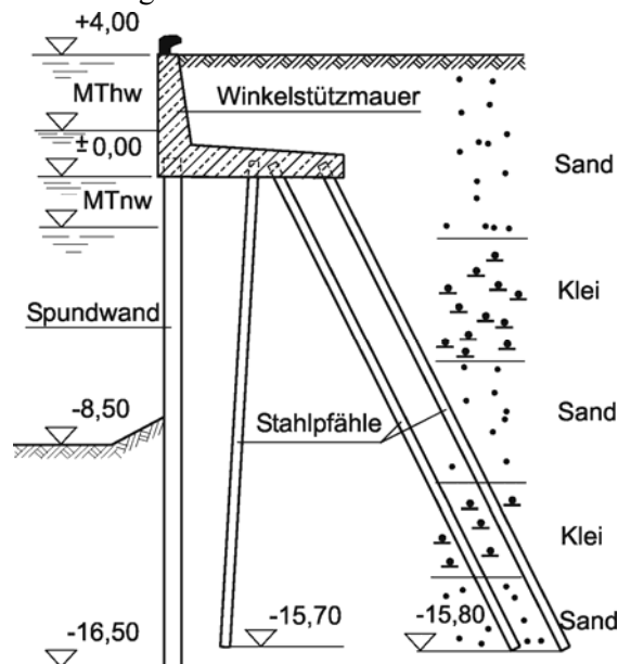
15-40 Pfahlrostbauwerk
