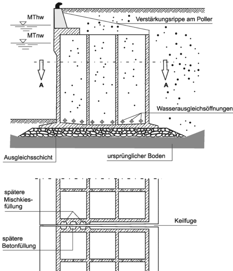
Schnitt A - A (nach dem Absetzen)
