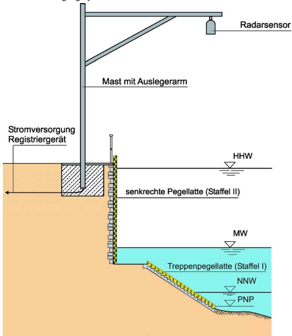
10-11 Radarpegel
