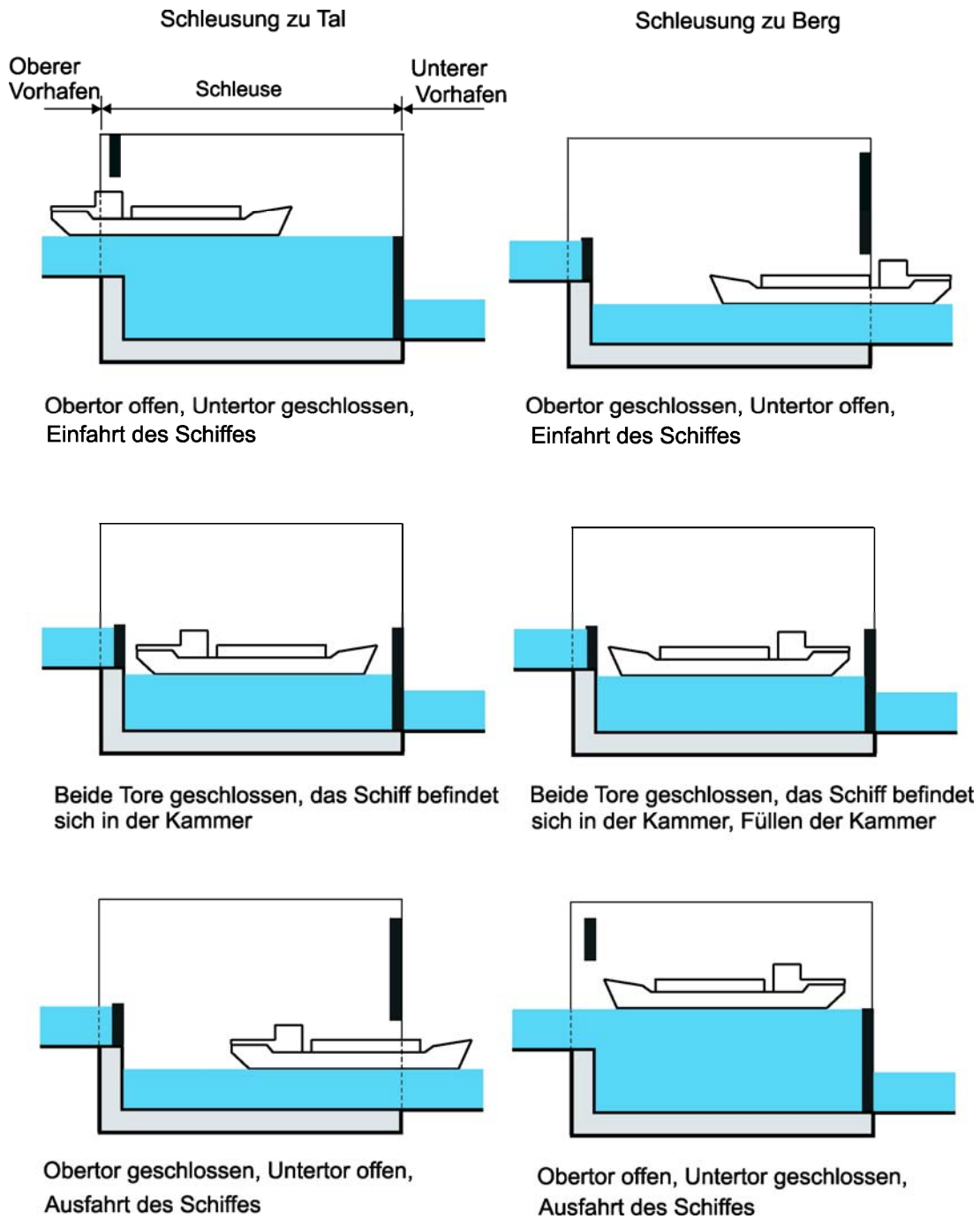
16-10 Schleusungsvorgang
