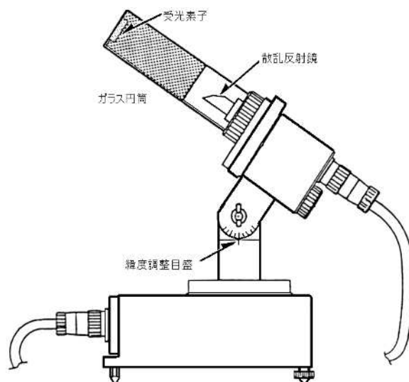
図 8-1 回転式日照計
