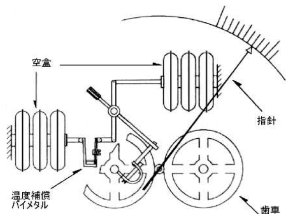
図 6-3 高精度のアネロイド型気圧計の構造
