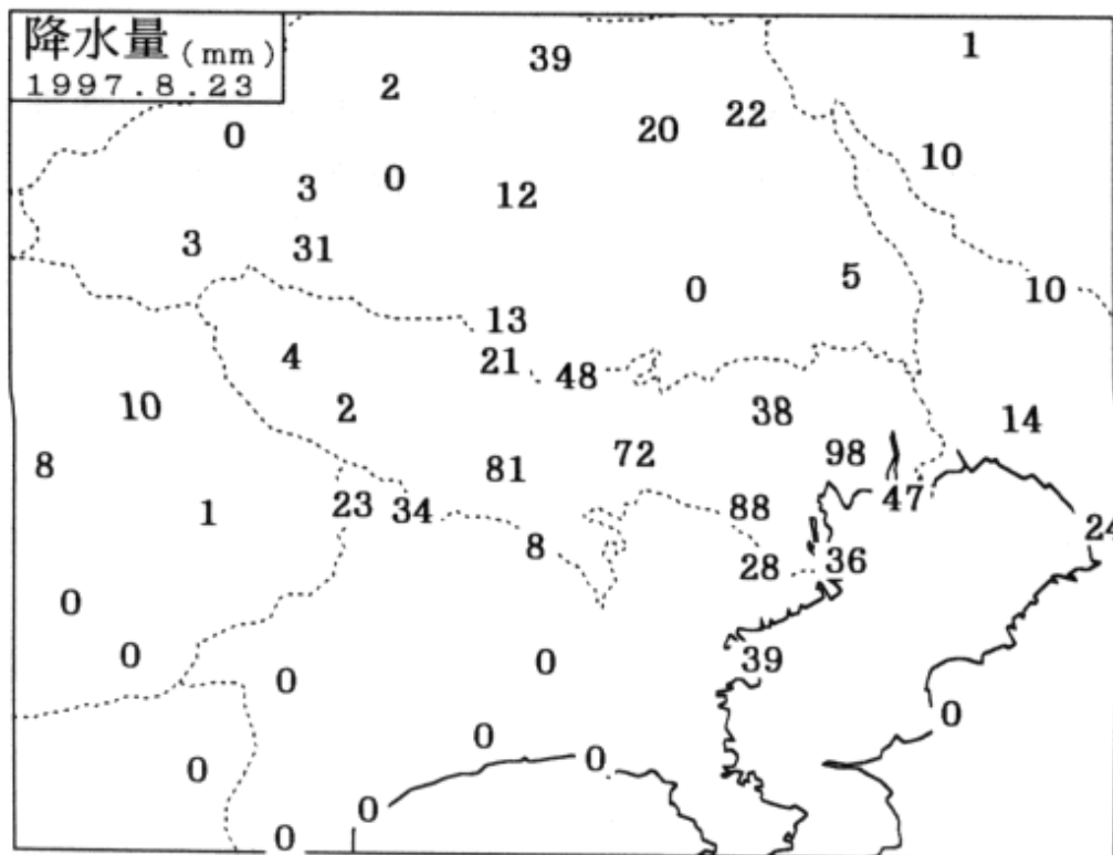
図13-6 雷雨による降水量の分布
