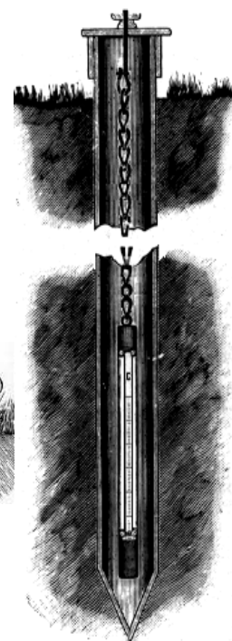
図3-5 鉄管地中温度計
