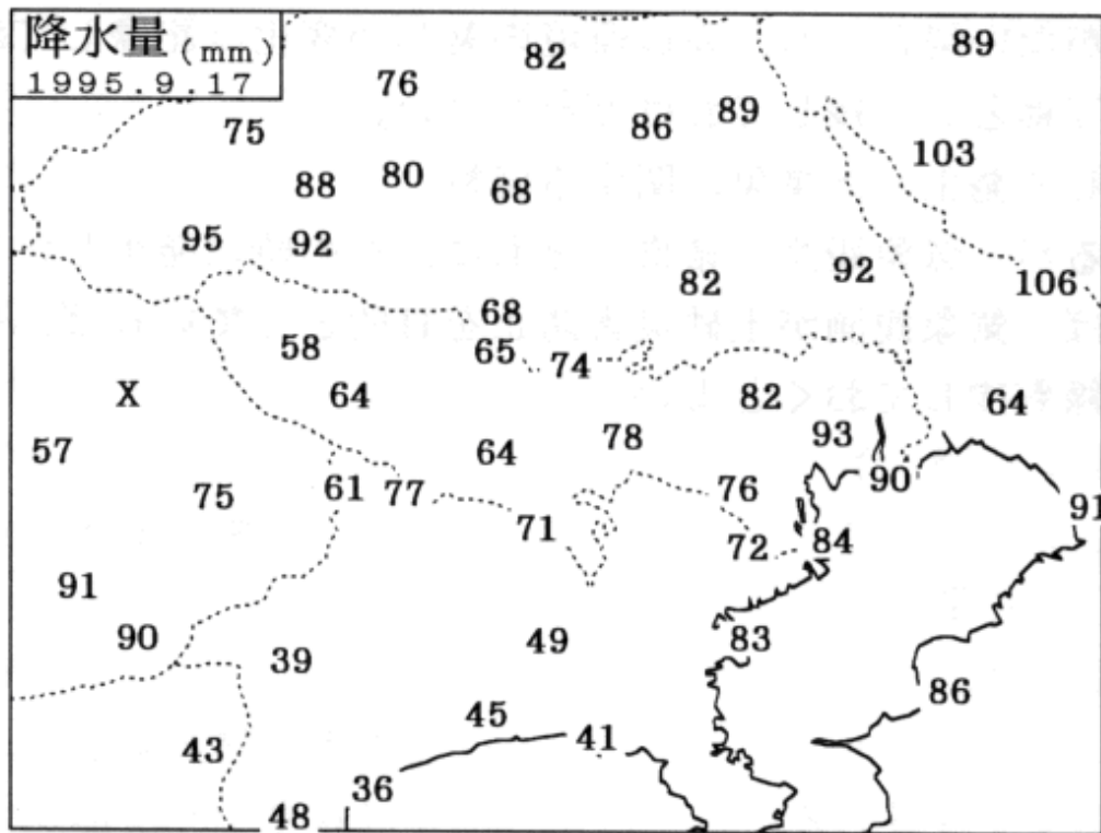
図13-5 前線と台風による降水量の分布
