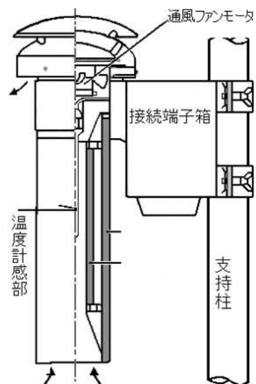
図3-3 温度計通風筒
