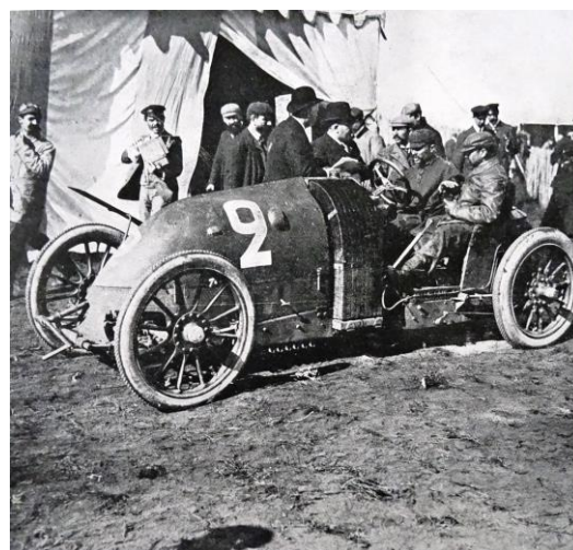
Renault de Sisz, grand prix de l'ACF 1905. (LFA).
