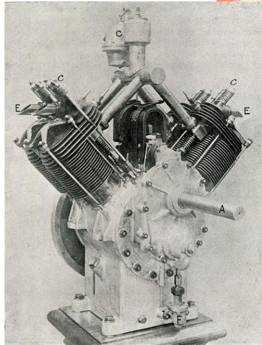
Moteur d'aviation Renault 4 B (1909) formé d'un demi V8. (L'Aérophile).
