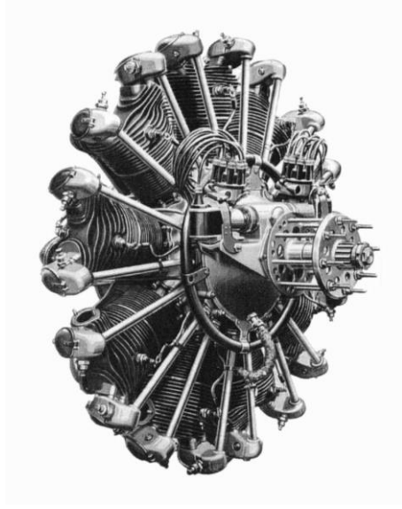
Moteur Renault 9A de 250 ch (1929).
