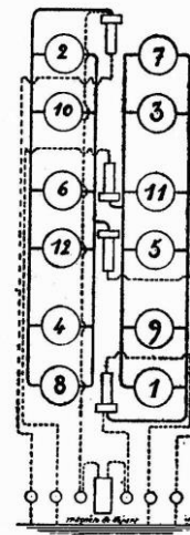
Moteur Renault 220 ch (type 12 E /F), ordre d'allumage des cylindres.
