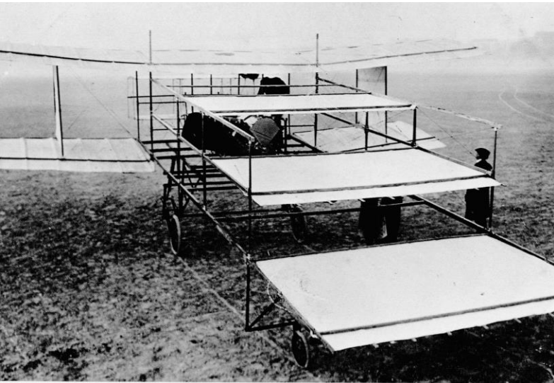
Biplan Witzig-Lioré-Dutilleul avec moteur Renault 50 ch photographié à Issy-les-Moulineaux en janvier 1909. (Musée de l'Air).
