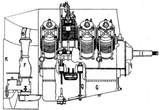
Moteur Renault V8 de 50-60 ch vu en coupe longitudinale. (L'Aérophile janvier 1911).
