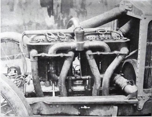
Moteur de course Renault de 100 ch du Grand Prix de l'ACF 1906. (LFA).
