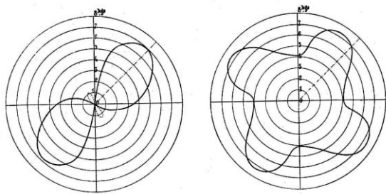
Fig. 14. — Variations du couple moteur dans le cas d'un 4 et d'un 8 cylindres. La distance de la courbe au centre est égale à la valeur du couple résultant de la pression par \text{cm}^2 sur le piston.
