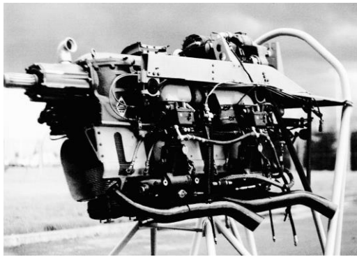
Moteur Renault 6Q de 220 ch restauré par le Musée SNECMA de Villaroche en 1987. (Musée SNECMA).
