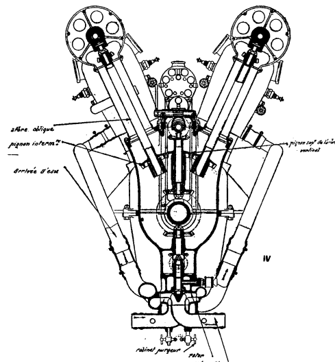
Renault type 12 E/F de 220 ch, coupe transversale par la distribution. (Manuel d'aviation de la 1 ère guerre mondiale).
