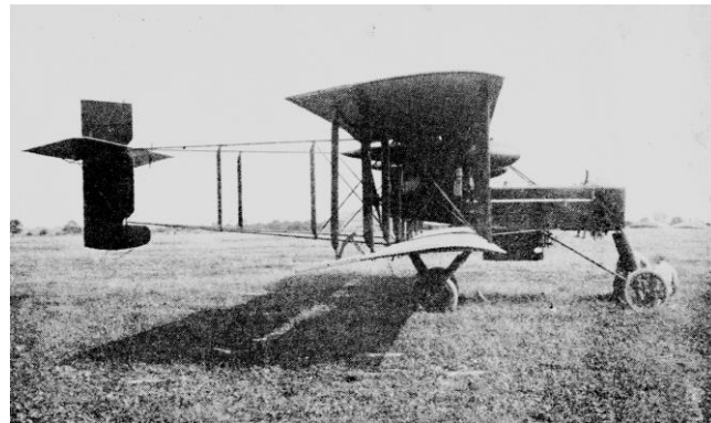
Bombardier Voisin type 10 à moteur Renault, succédant au type 8 dont le moteur V8 Peugeot n'est pas fiable.
