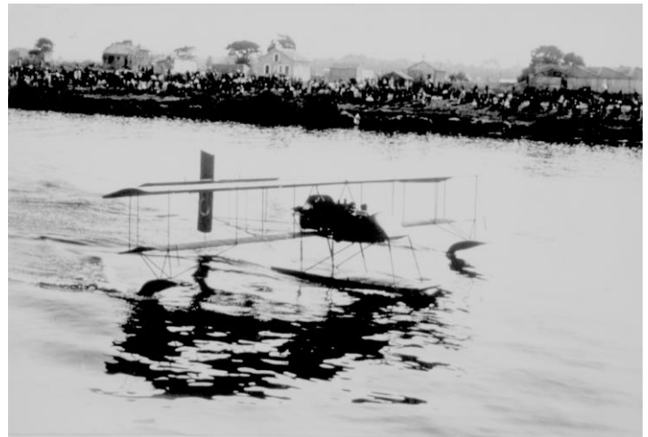
Le biplan Sanchez-Bathiat construit à Billancourt en 1912, vu ici aux essais au Pecq en 1913 avant la course de Deauville, propulsé par un V12 Renault. (Archives mun. de Boulogne-Billancourt).
