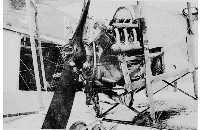
Le MF-11 « shorthorn » à moteur Renault 70 ch construit en Angleterre. (Musée de la R.A.F.).
