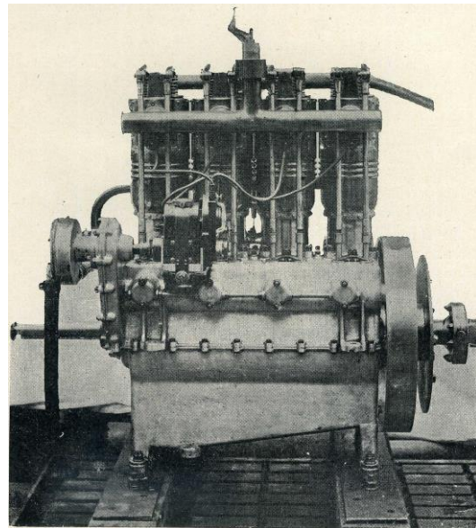
Renault 4A, refroidissement par eau, 9 litres de cylindrée, 35/40 ch selon le régime, masse 100 kg. (Moteurs d'aviation et de dirigeables).
