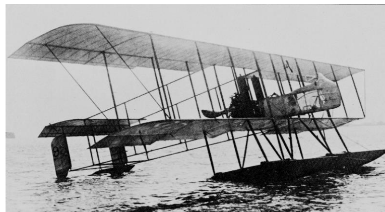
Dérivé marin du MF-11, cet hydravion participa de 1912 à 1914 au concours de Monaco, piloté par Eugène Renaux.
