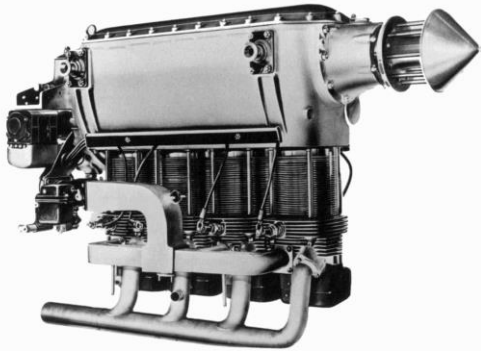
Moteur Renault 4-cyl inversés type 4 Pci de 100/110 ch (1932). (Musée Renault).
