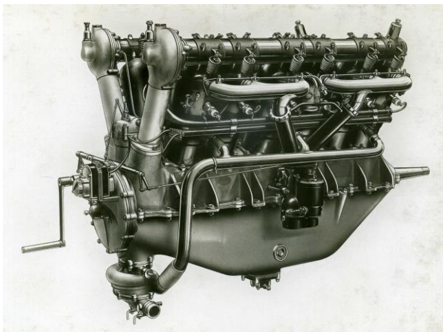
Moteur Renault 12 E/F de 220 ch (1915), une belle mécanique de 177 cm de long, robuste et puissante. (Musée Renault)
