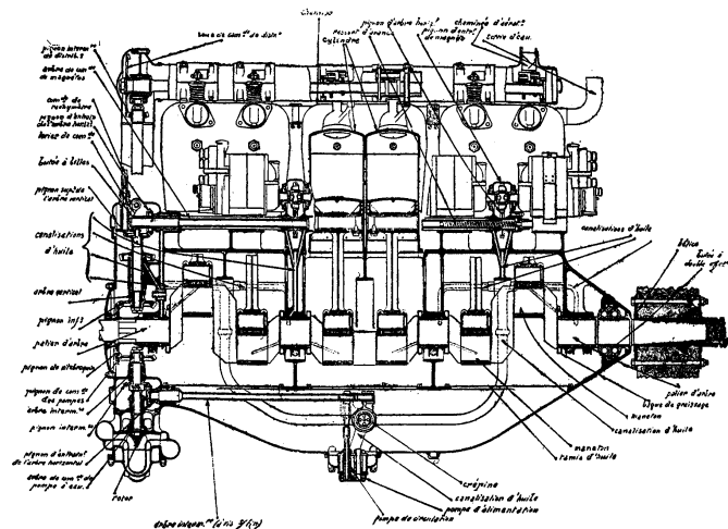
Moteur Renault 220 ch. (Manuel d'aviation de la 1 ère guerre mondiale, ministère de la guerre).
