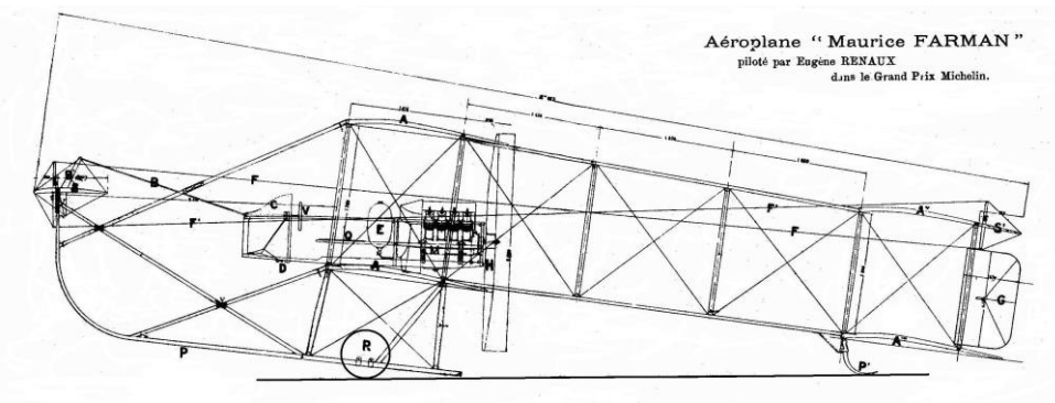
Le MF-2 « grandes ailes » de Renaux et Senouque, victorieux du Grand Prix Michelin. (L'Aérophile).
