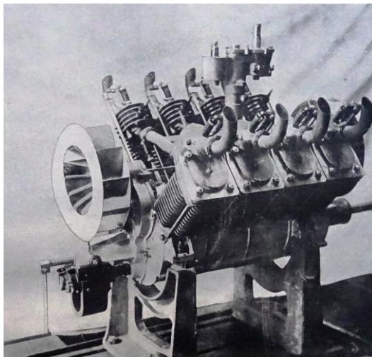
Le premier moteur Renault d'aviation, présenté en décembre 1907 au Salon de l'auto. (LFA).
