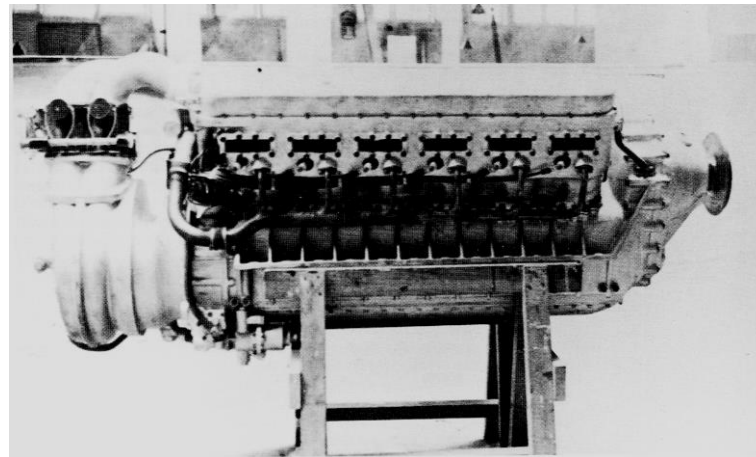
Moteur 12N de 2000 ch destiné aux hydravions de vitesse de la Coupe Schneider 1931. (Musée Renault).
