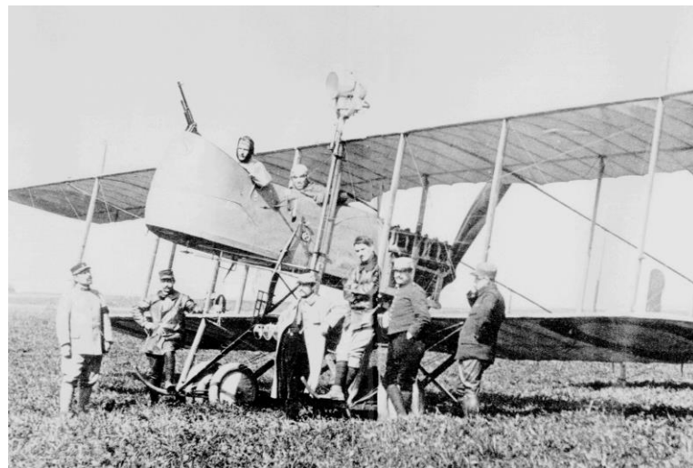
Biplan Maurice Farman MF-11 à moteur V12 Renault de 130 ch (1916). (Cliché Musée de l'Air).
