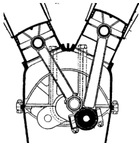
Embiellage type bielle maîtresse (à droite) et secondaire (à gauche) utilisé sur le V12 Renault.
