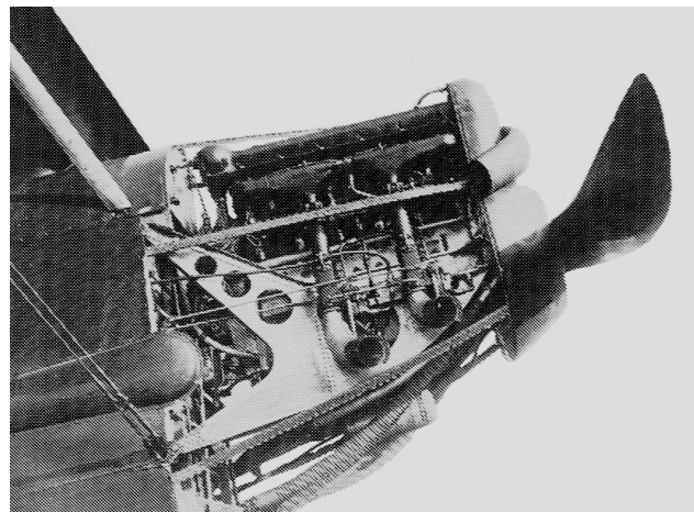
Prototype du Potez 28.2 à moteur Renault 12 Kg de 550 ch. (Cliché Musée SNECMA).
