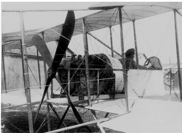
Le premier Renault V12 d'aviation, en 1912, monté sur un biplan Maurice Farman. (Musée Renault).
