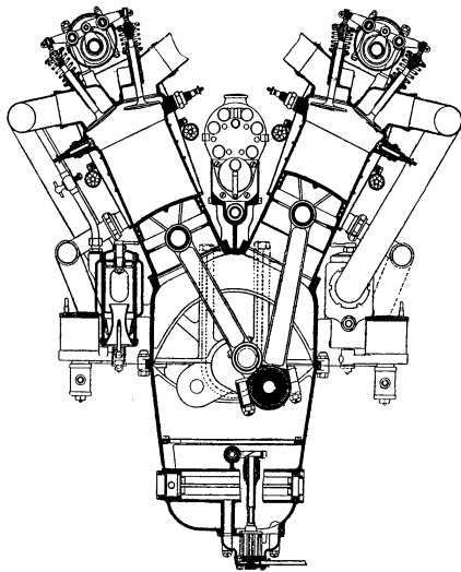
Moteur Renault 12 E 1915 développant 220 ch. (Manuel d'aviation de la 1 ère guerre mondiale).
