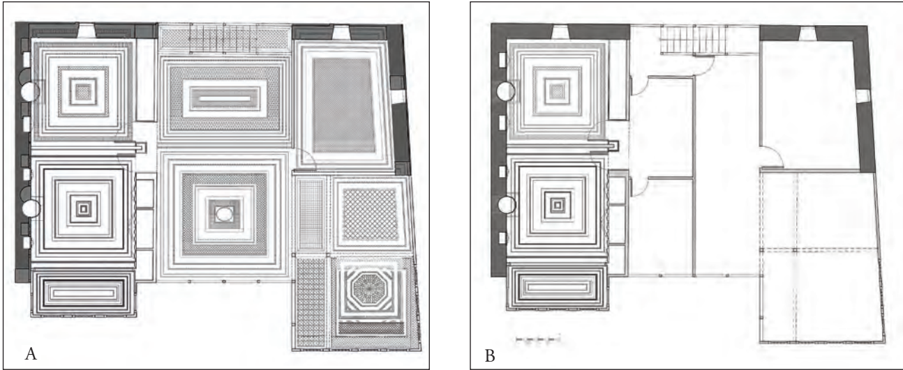
Εικ. 140α- β. Σχέδια αποκατάστασης της κάτοψης του καλού ορόφου του αρχοντικού Τοιμινάκη-Δημοξένους σε δύο φάσεις της λειτουργίας του (σχέδια της Έλ. Τουτουντζή).
