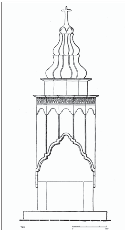
Εικ. 68. Το «μπουχαρί»: αποτύπωση τζακιού σε οντά της Κοζάνης.
