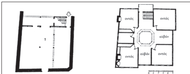
Εικ. 6. Το σπίτι Βογοτόφ στην Κοπήρφιστησα της Βουλγαρίας (κατόψεις).
