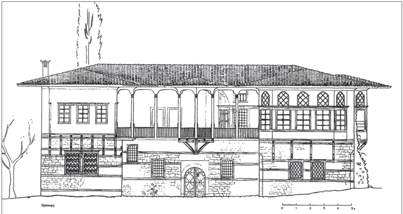
Εικ. 61. Αποτύπωση όψης του αρχοντικού Χατζηδημητρίου-Δημισκή (σχέδιο της Αλεξάνδρας Πασχαλίδου-Μωρέτη).
