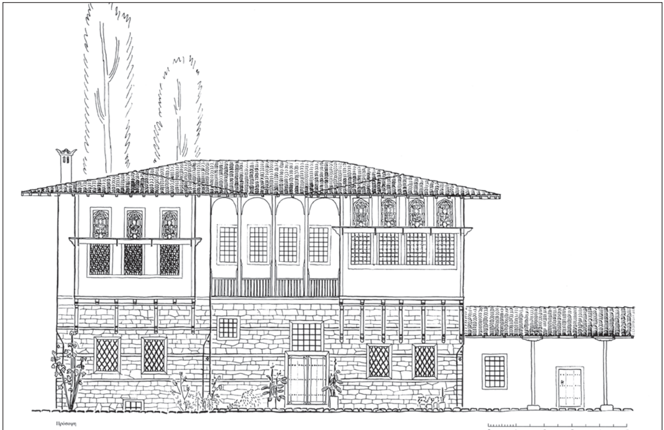
Εικ. 60. Αποτύπωση όψης του αρχοντικού Γρ. Βούρκα (σχέδιο της Αλεξάνδρας Πασχαλίδου-Μωρέτη).
