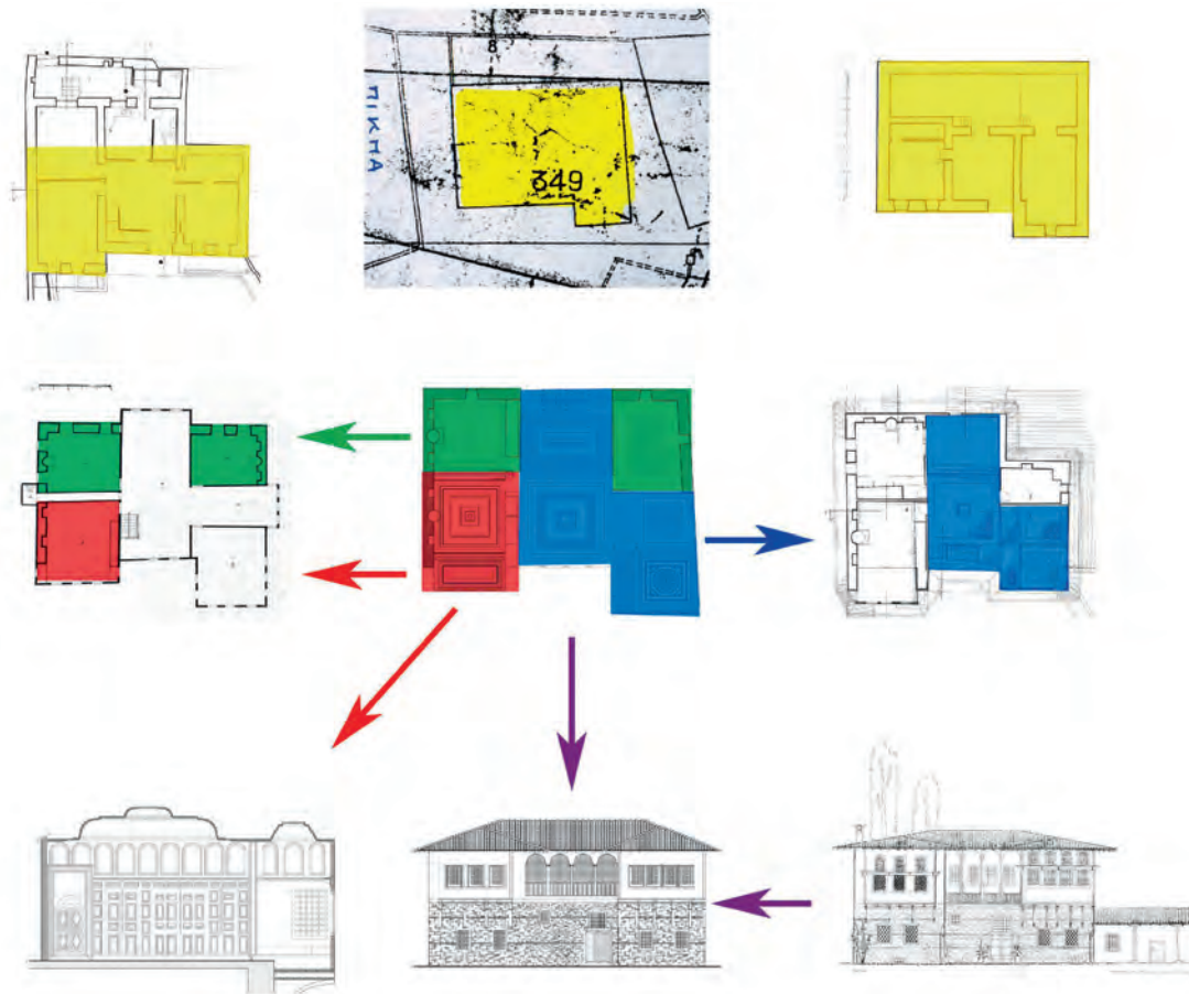
Εικ. 142. Πίνακας με σχέδια συγκριτικής τεκμηρίωσης της μορφής του αρχοντικού Τοιμινάκη-Δημοξένους.
