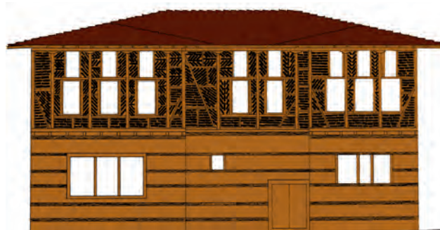
Εικ. 57. Εξωτερικοί τοίχοι - κατασκευαστικό ισόγειο και ορόφου.
