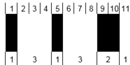
Abbildung 5.4.3.1-2. Symbolzeichenwert 35
