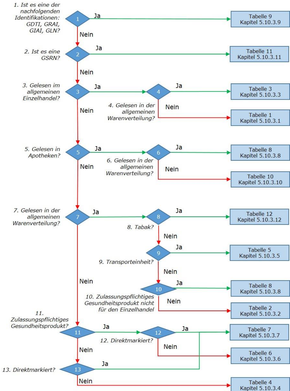
Abbildung 5.10.2.6-2. Entscheidungsbaum
