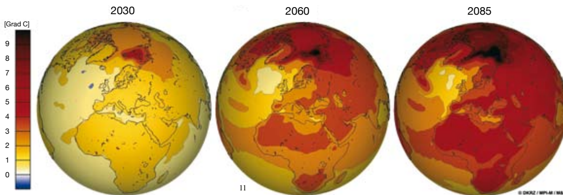
Abbildung 1: Globale Temperaturveränderung gemäß Klimaszenario A1B der UNO. Dieses globale Szenario bildet die klimatologische Basis der vorliegenden Studie.
