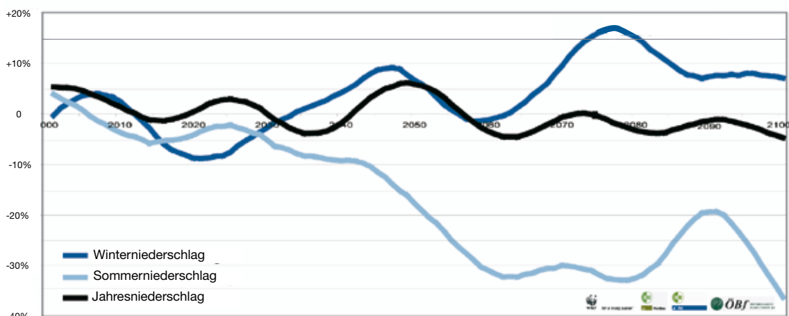
Abbildung 5: Entwicklung der Jahresniederschläge in Österreich gemäß dem UNO-Klimaszenario A1B. Dargestellt sind die Entwicklung von Sommer-, Winter- und Jahresniederschlägen. Die Winterniederschläge nehmen zu (dunkelblau), die Sommerniederschläge nehmen ab (hellblau), die Jahresniederschläge bleiben etwa gleich.
