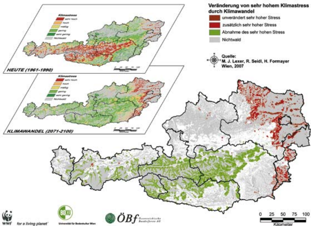
Abbildung 8: Veränderung der Stressbelastung für Buche durch Klimawandel. 34 Im Insert sind anhand von zwei Karten die Klimastress-Belastung der Buche heute und unter Klimawandel in fünf Stress-Kategorien dargestellt. Die Hauptkarte zeigt die Gebiete mit sehr hoher Stressbelastung und gibt deren flächenmäßige Veränderung (Ausdehnung, Verringerung) durch Klimawandel wieder.
