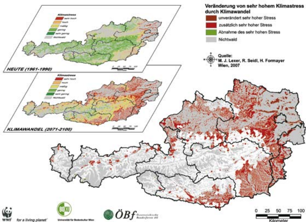
Abbildung 7: Veränderung der Stressbelastung für Fichte durch Klimawandel unter Berücksichtigung von Borkenkäferstörungen. 34 Im Insert sind anhand von zwei Karten die Klimastress-Belastung der Fichte heute und unter Klimawandel in fünf Stress-Kategorien dargestellt. Die Hauptkarte zeigt die Gebiete mit sehr hoher Stressbelastung und gibt deren flächenmäßige Veränderung (Ausdehnung, Verringerung) durch Klimawandel wieder.
