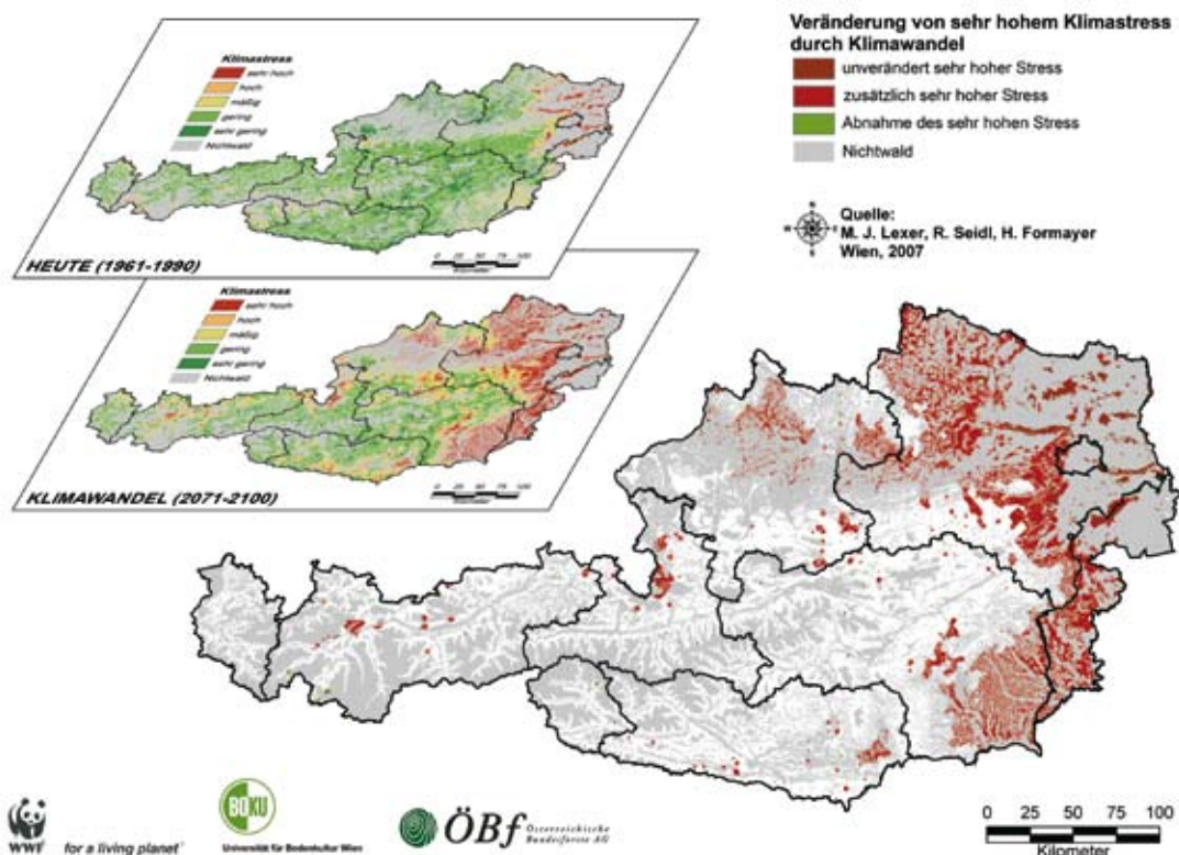
Abbildung 6: Veränderung der Stressbelastung für Fichte durch Klimawandel. 34 Im Insert sind anhand von zwei Karten die Klimastress-Belastung der Fichte heute und unter Klimawandel in fünf Stress-Kategorien dargestellt. Die Hauptkarte zeigt die Gebiete mit sehr hoher Stressbelastung und gibt deren flächenmäßige Veränderung (Ausdehnung, Verringerung) durch Klimawandel wieder.
