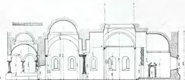
Fig. 199. — Coupe
