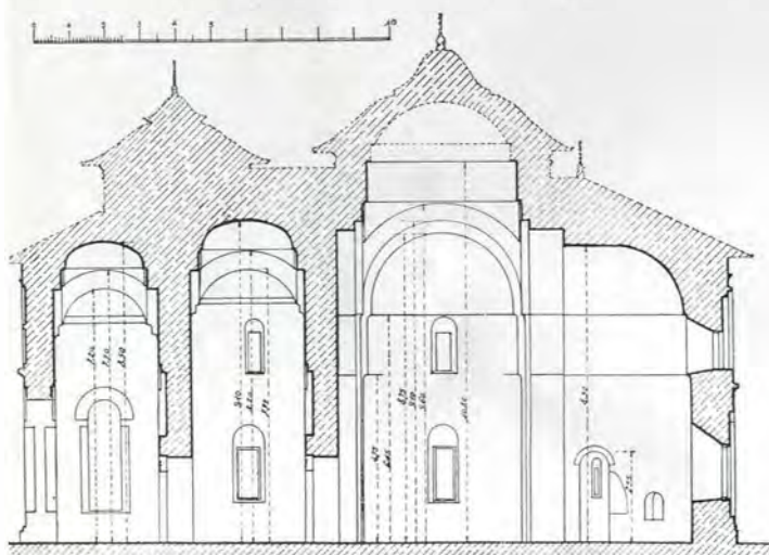
Fig. 198. — Coupe
