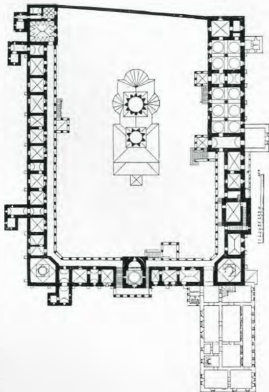
Fig. 236. — Plan
