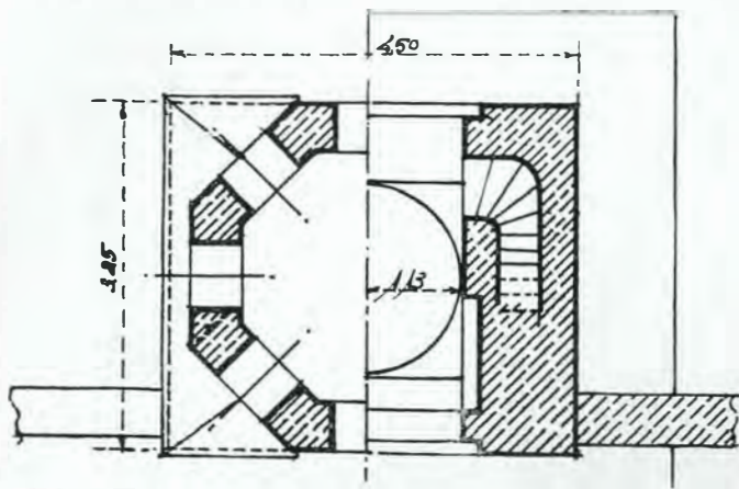
Fig. 242. — Plan
