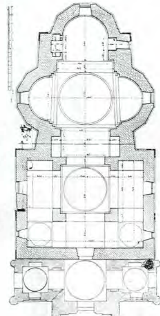
Fig. 169. — Plan de Radu Vodă
