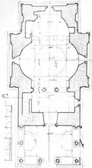
Fig. 222. — Plan
