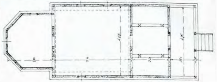
Fig. 322. — Plan
