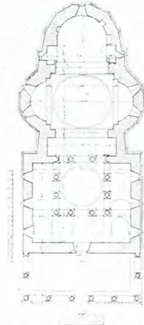
Fig. 211. — Plan
