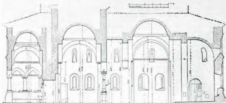
Fig. 230. — Coupe
