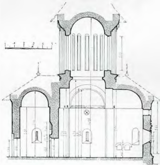
Fig. 118. — Coupe de Căluu
