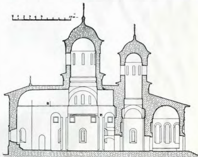
Fig. 109. — Coupe
