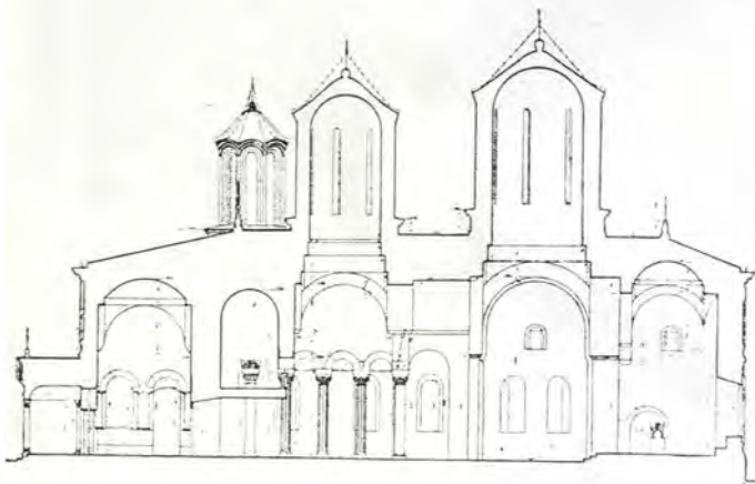
Fig. 212. — Coupe
