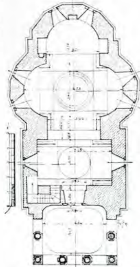
Fig. 223. — Plan
