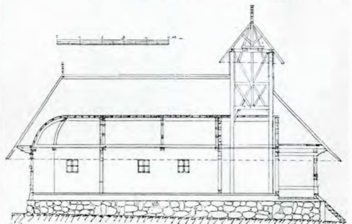
Fig. 323. — Coupe
