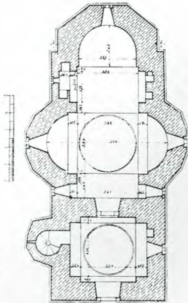
Fig. 216. — Plan
