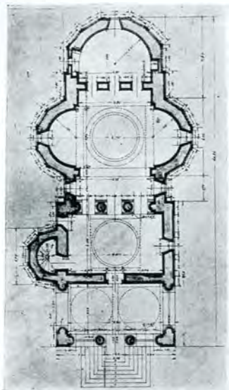
Fig. 347. — Plan
