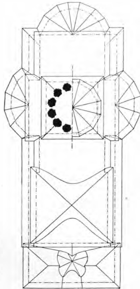
Fig. 33. — Plan de la toiture
