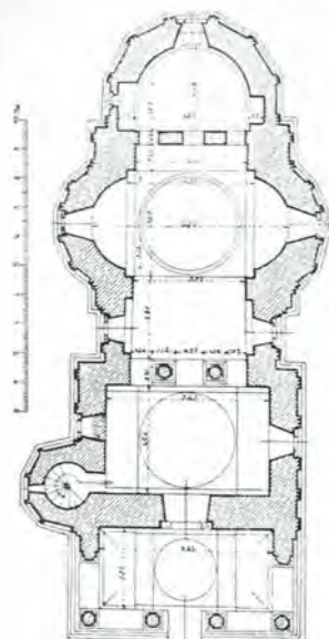
Fig. 303. — Plan
