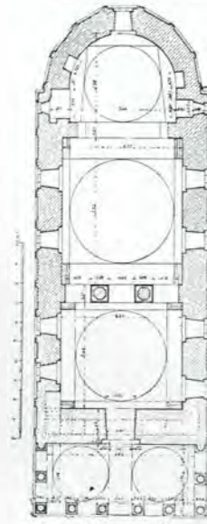
Fig. 190. — Plan
