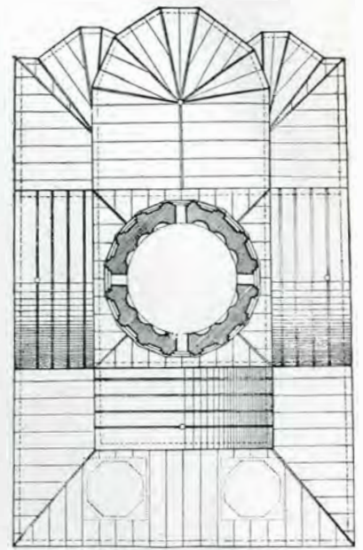
Fig. 44. — Plan des toitures
