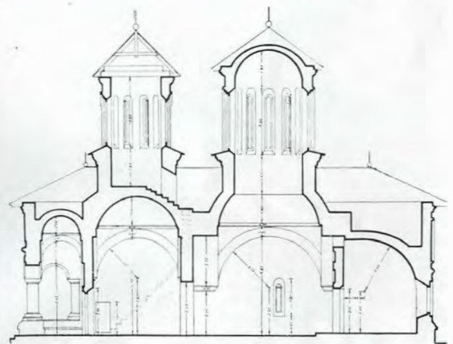
Fig. 338. — Coupe
