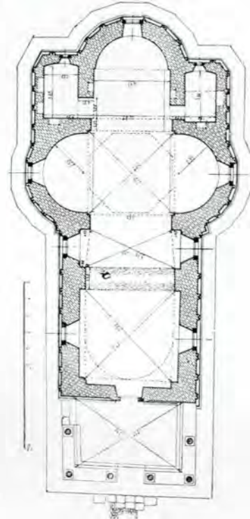
Fig. 126. — Plan
