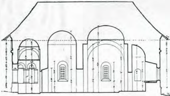
Fig. 268. — Coupe
