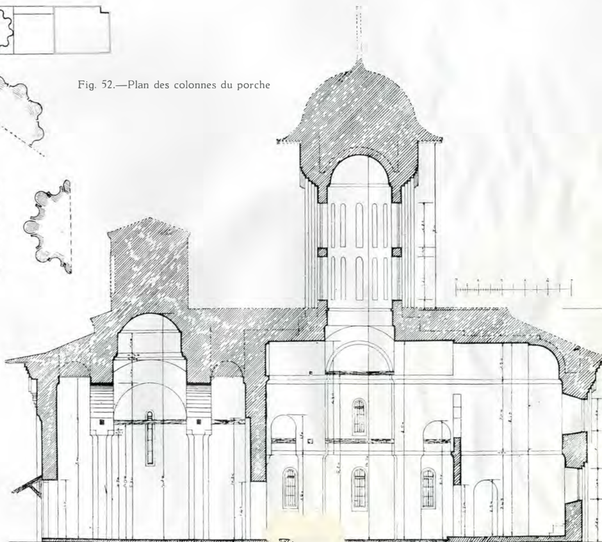
Fig. 52. Coup longitudinal
