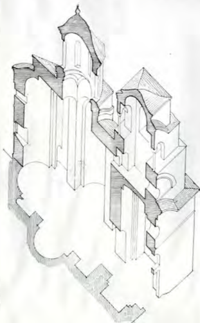
Fig. 21. — Coupe perspective
