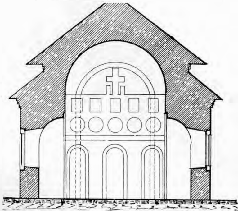
Fig. 13. — Coupe transversale
