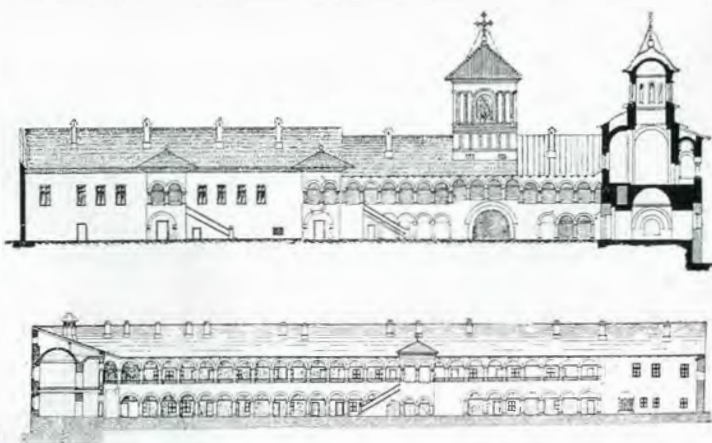
Fig. 238-239. — Coupes
