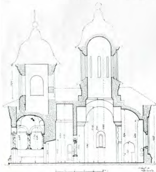
Fig. 224. — Coupe
