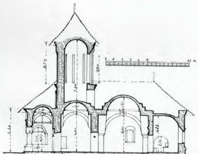
Fig. 282. — Coupe
