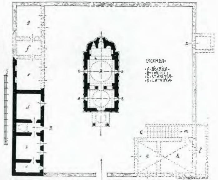
Fig. 184. — Plan
