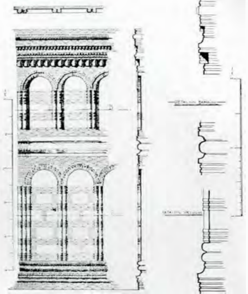
Fig. 120. — Détail de Marcuța
