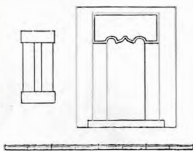
Fig. 3. — Biserica din Bohari. Cadrul ferestrei și al ușii. (rel. arh. Em. Costescu)
