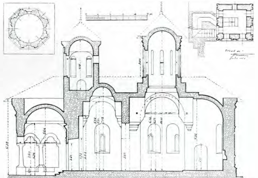
Fig. 225. — Coupe
