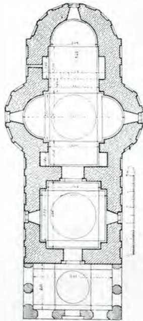
Fig. 165. Plan
