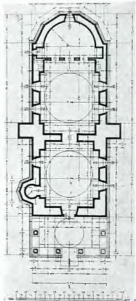
Fig. 279. — Plan
