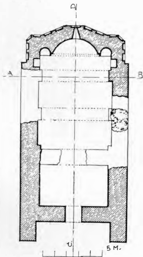
Fig. 3. — Plan de l'Église de San-Nicoara à Curtea de Argeş
