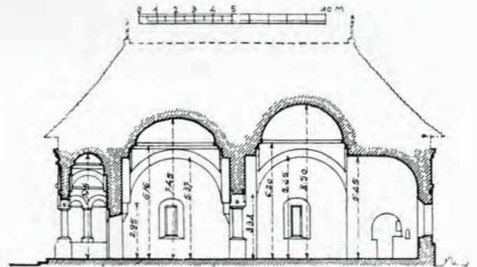
Fig. 269. — Coupe
