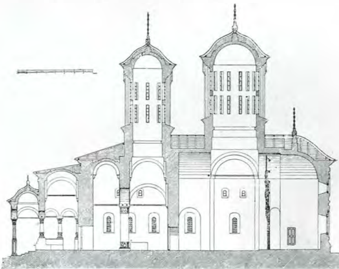
Fig. 205. — Coupe
