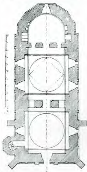
Fig. 177. — Plan
