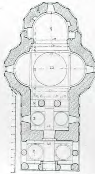
Fig. 204. — Plan
