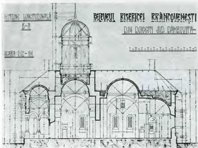
Fig. 281. — Coupe
