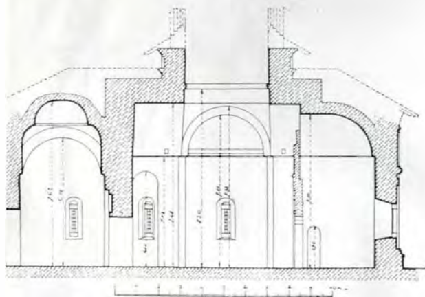
Fig. 124. — Coupe
