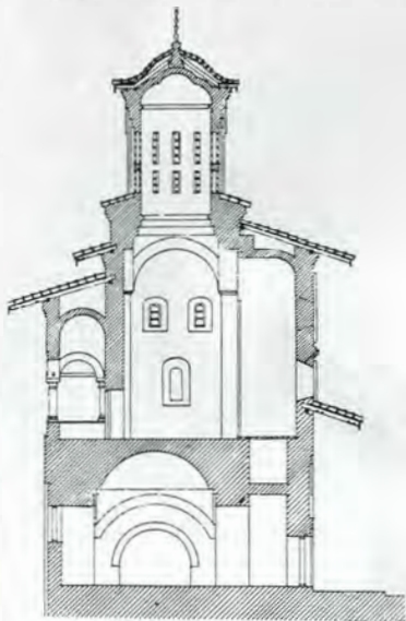
Fig. 185. — Coupe
