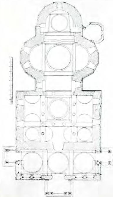
Fig. 210. — Plan
