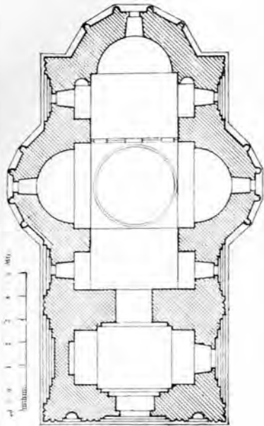
Fig. 19. — Plan
