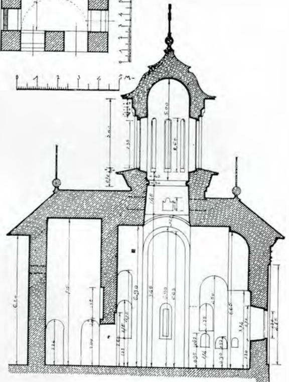
Fig. 115. — Coupe de Cozia
