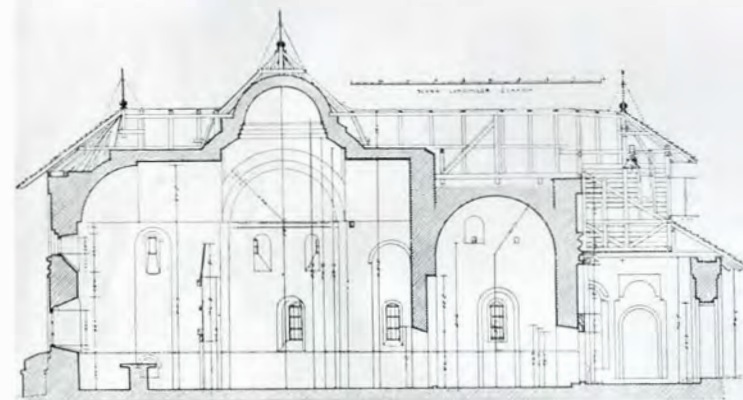
Fig. 160. — Coupe
