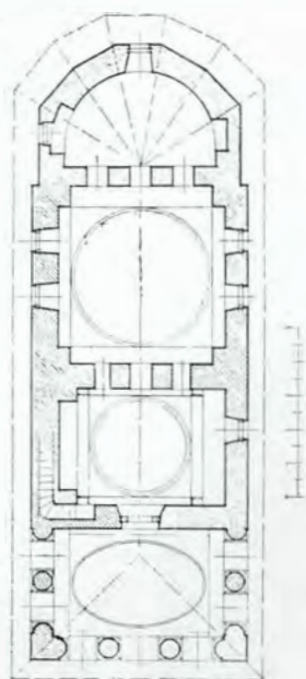
Fig. 285. — Plan
