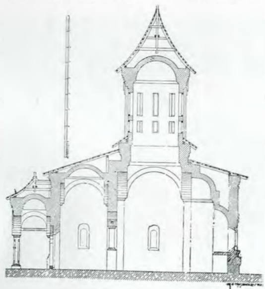
Fig. 186. — Coupe
