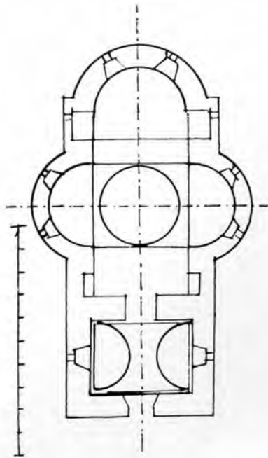
Fig. 25. — Plan
