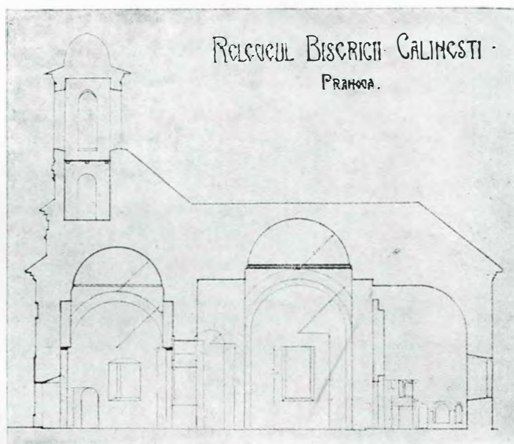
Fig. 150. — Coupe
