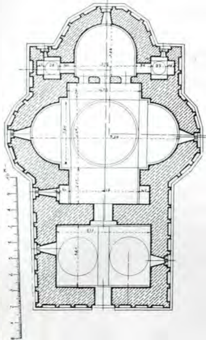
Fig. 123. — Plan
