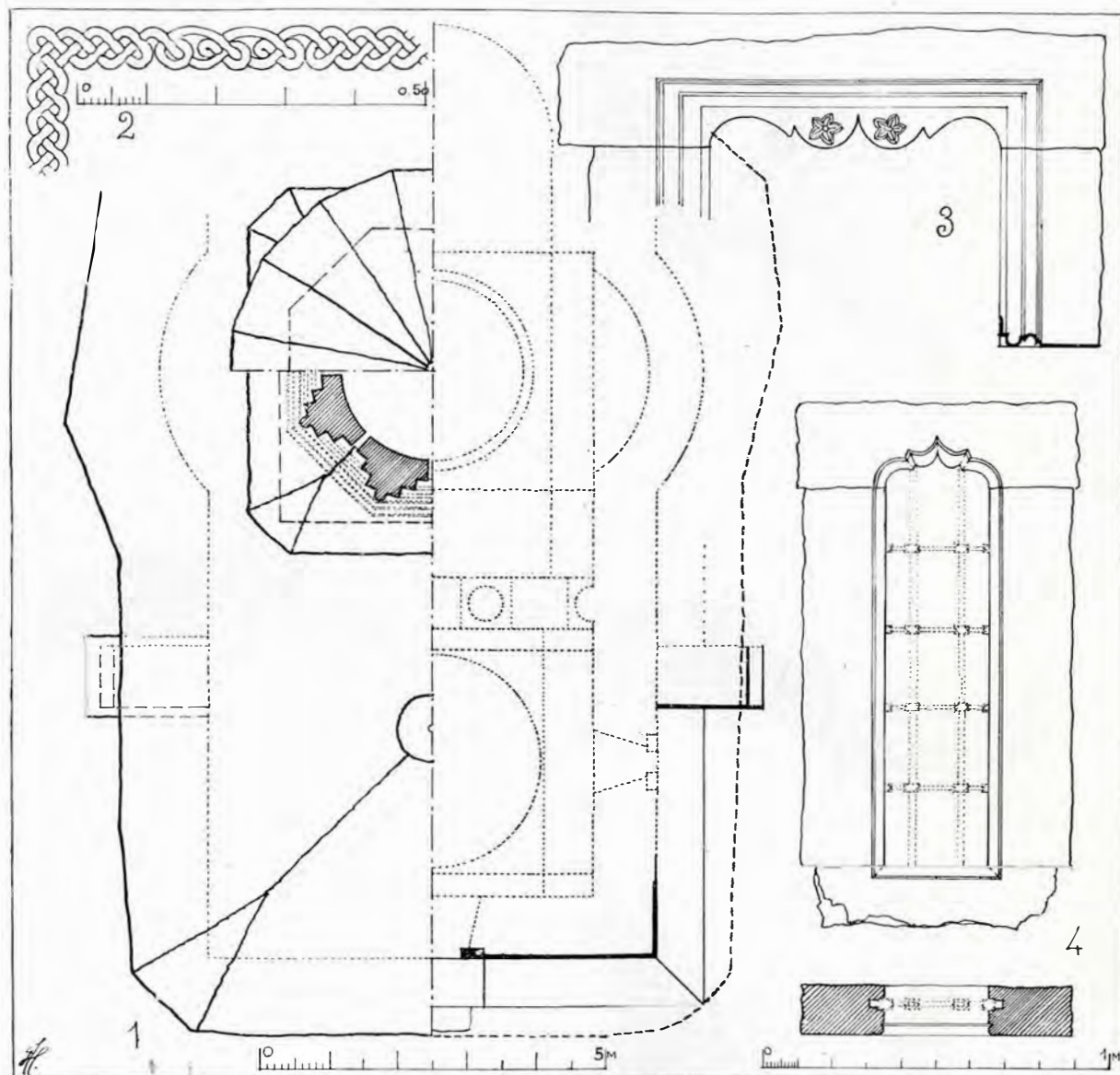
Fig. 10. — Biserica Schitului Mărculești-Flămânda. 1) Plan ipotetic dedus din conturul strășinei acoperișului, restituit după fotografii; 2) Chenarul sculptat al pisaniei și 3) Cadrul ușei restituite după fotografii; 4) Ferestrele reconstituite după blocurile de piatră ce s'au găsit.
