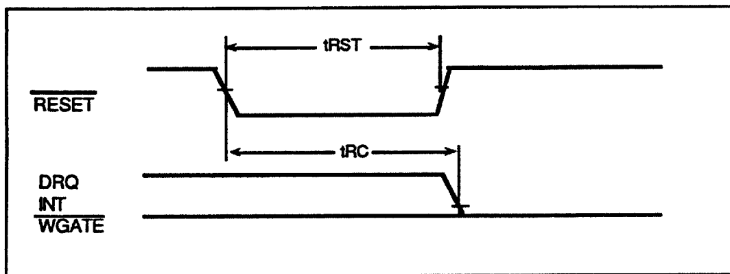
Fig. 9 Negative Reset
