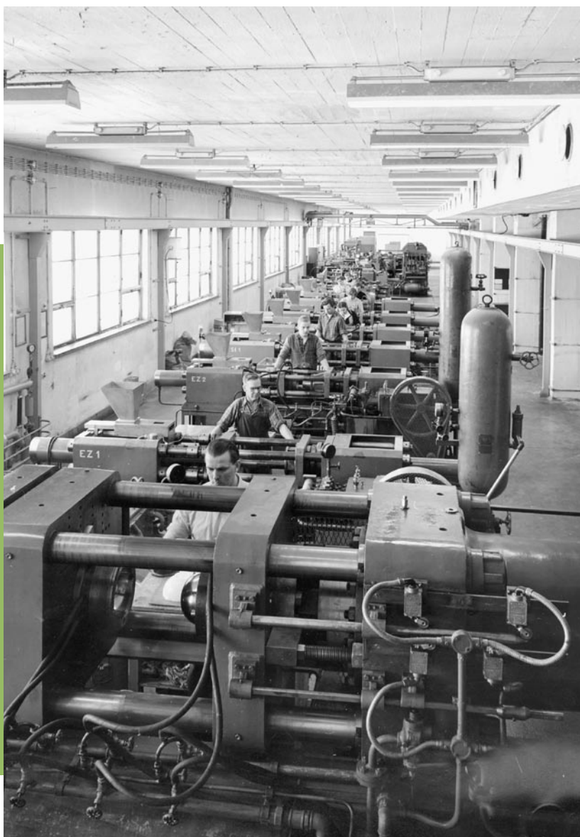
Tehtaan kestumuovipuristamo vuodelta 1959, jolloin suurimmalla ruiskupuristuskoneella voitiin valmistaa korkeintaan 1,5 kilon painoisia tuotteita. Kuva: Muoviyhdistys.
