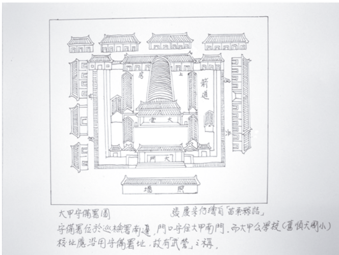
照 3-3-14 大甲中軍守備署平面圖
