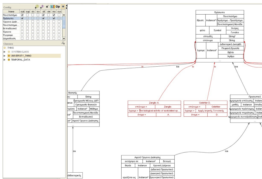
Fig. 2. Protégé OntoViz visualization.
