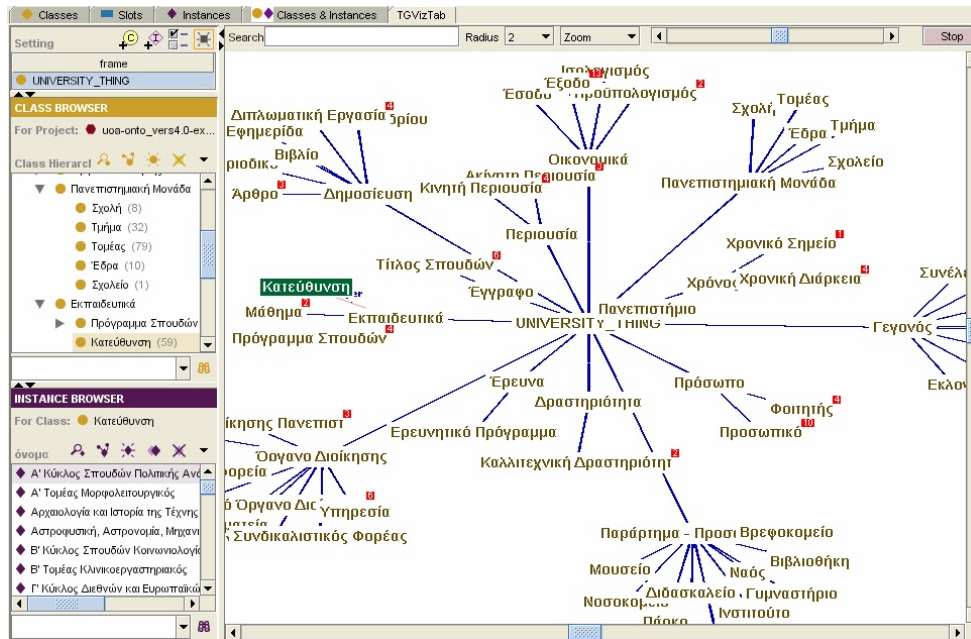
Fig. 10. Protégé TGvizTab
