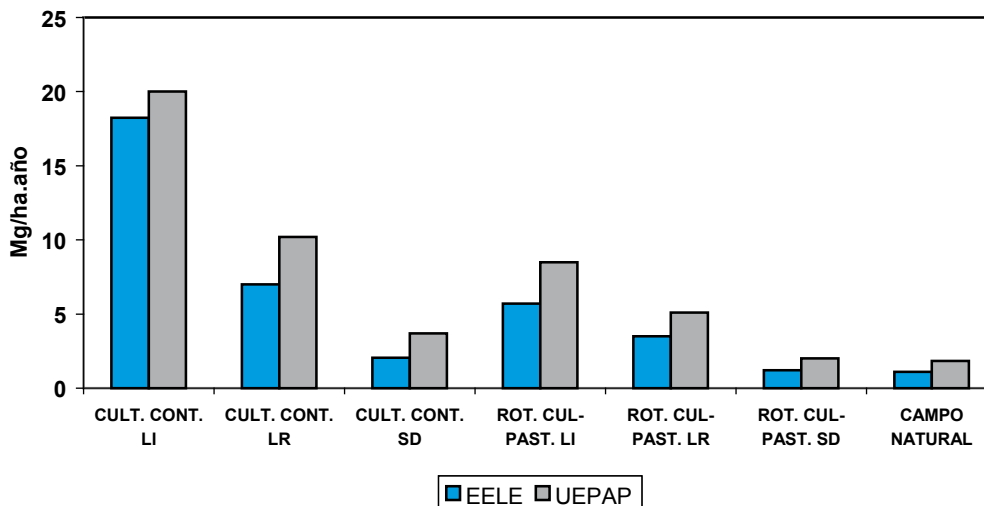
Figura 2.23 Erosión promedio en parcelas (de escurrimiento) en diferentes sistemas de producción con Laboreo Intensivo (LI), Laboreo Reducido (LR) y Siembra Directa (SD).
