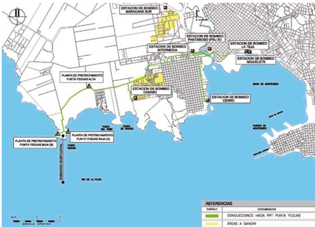
Figura 5.14 Obras comprendidas en el PSU IV Fuente: CSI et al. 2006
