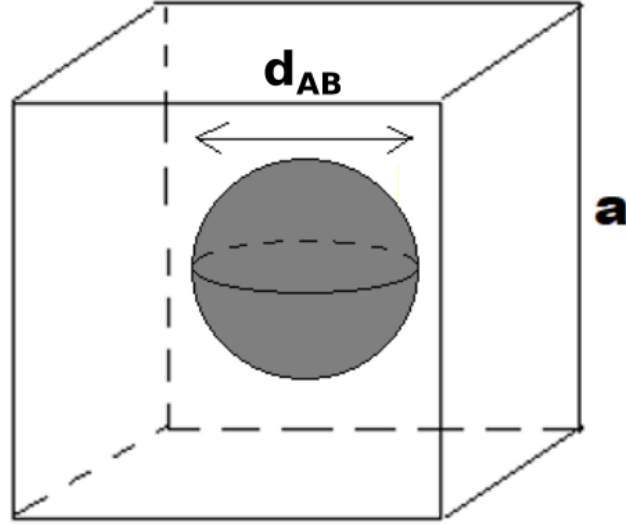
Figure 3.3 Représentation d'un cube élémentaire d'ergol solide : un cube de paraffine de côté a , avec un coeur d'AB de diamètre d_{AB}
