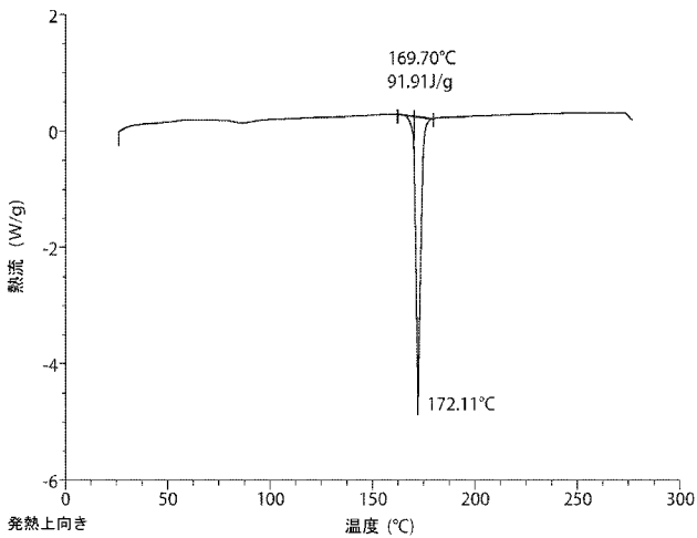
形態16のDSCプロファイル
