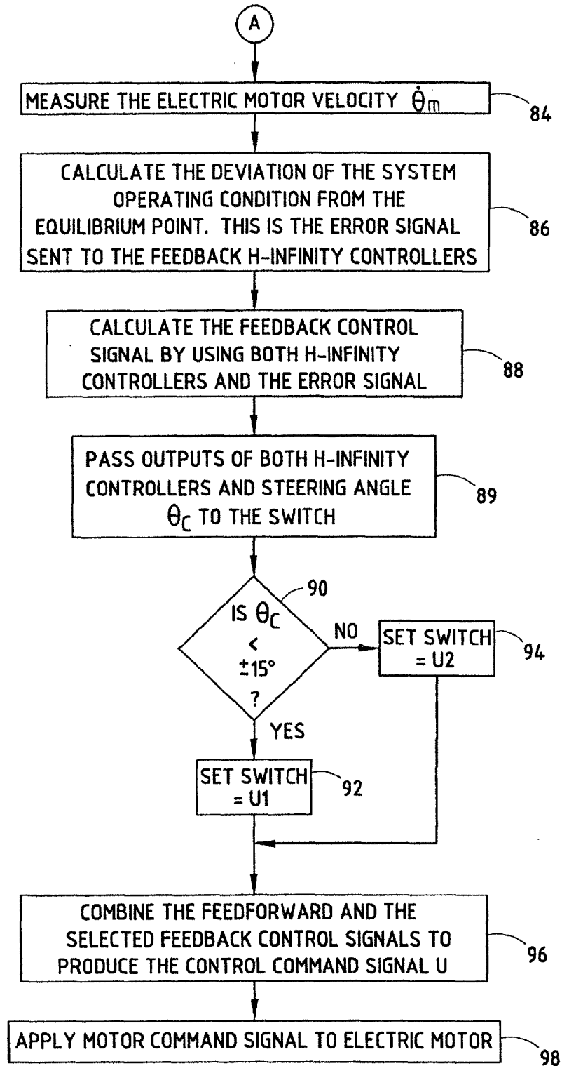
FIG. 5B
