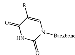
R = H: Uracil R = CH 3 : Thymine
