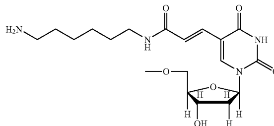
Amino modifier C6 dT
