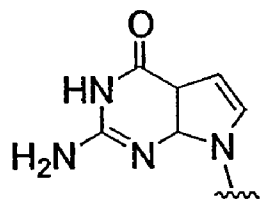
N9-(7-deaza-G)
