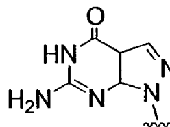
N9-(7-deaza-8-aza-G)
