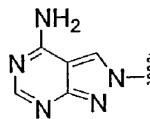
N8-(7-deaza-8-aza-A)
