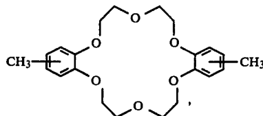
(20) 1,2-tert-Butylbenzo-18-crown-6
