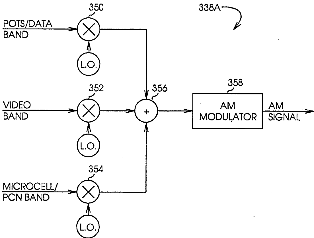
AM Modulator Fig. 25
