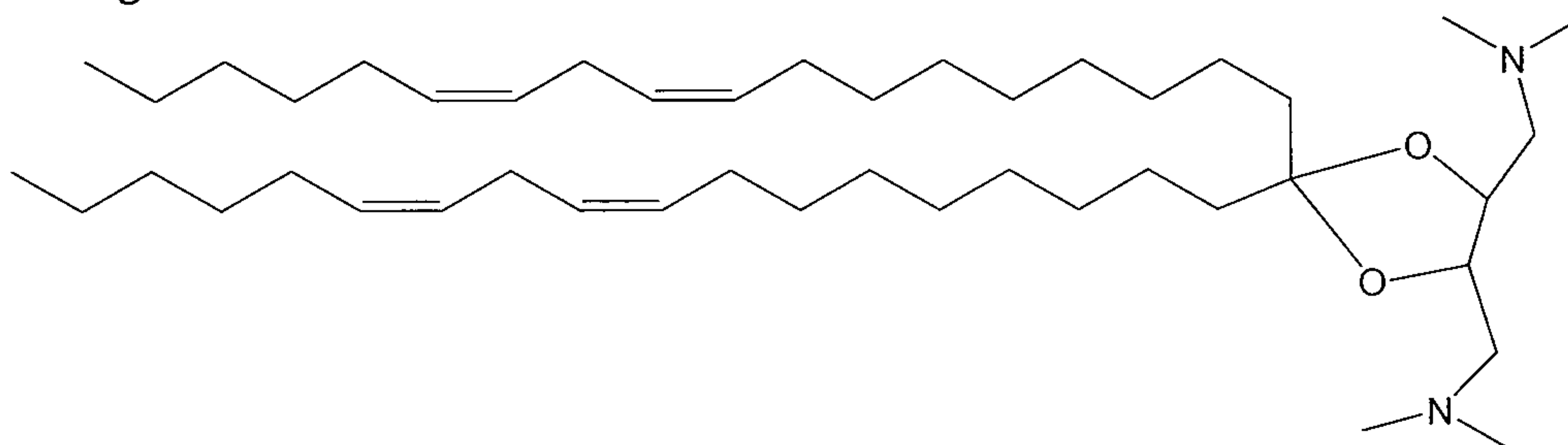
DLin-K 2 -DMA.
