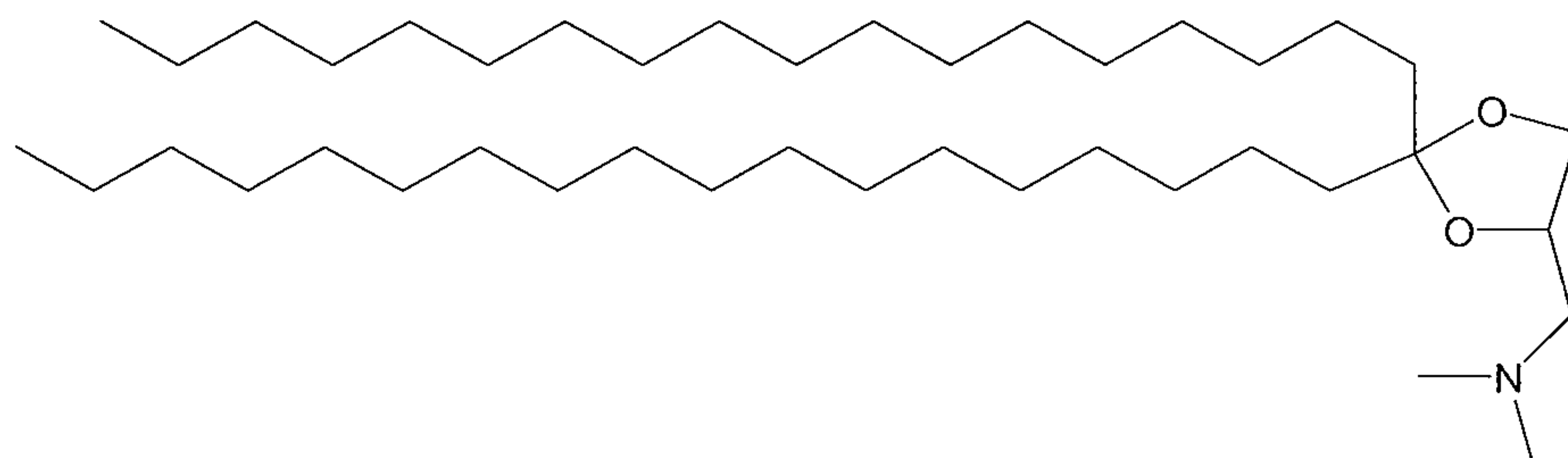
DS-K-DMA;
