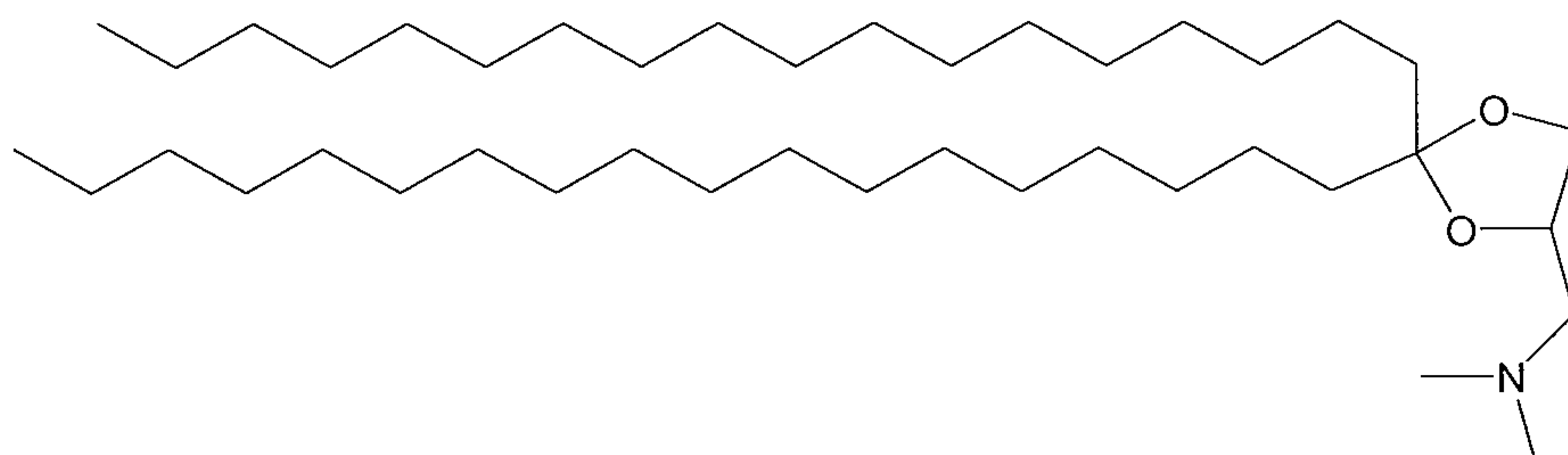
DS-K-DMA
