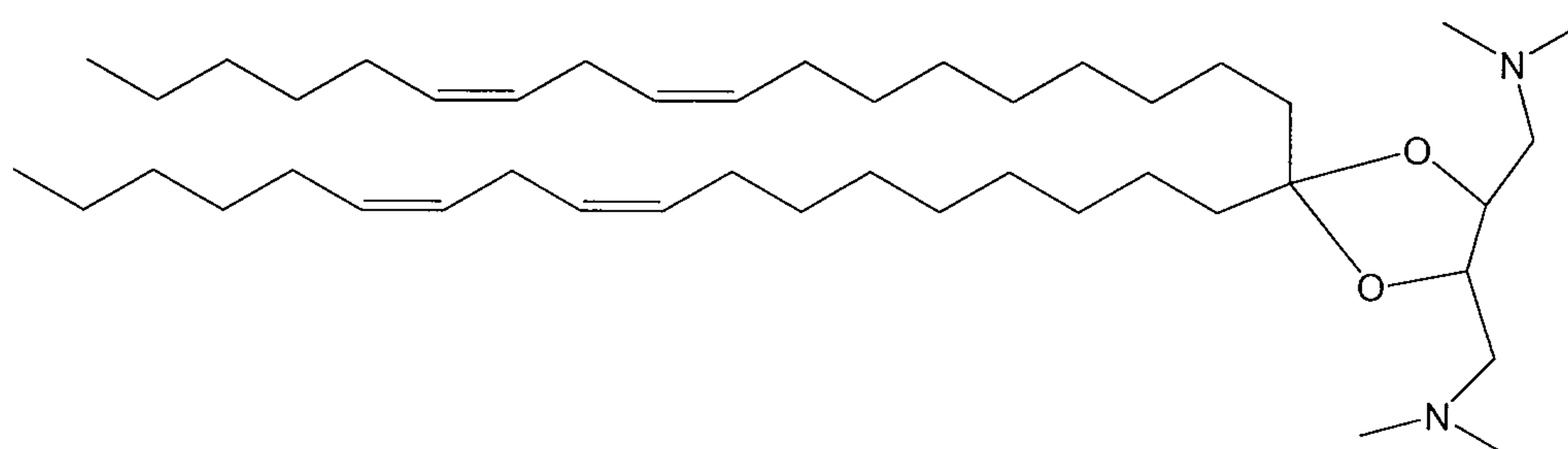
DLin-K 2 -DMA;
