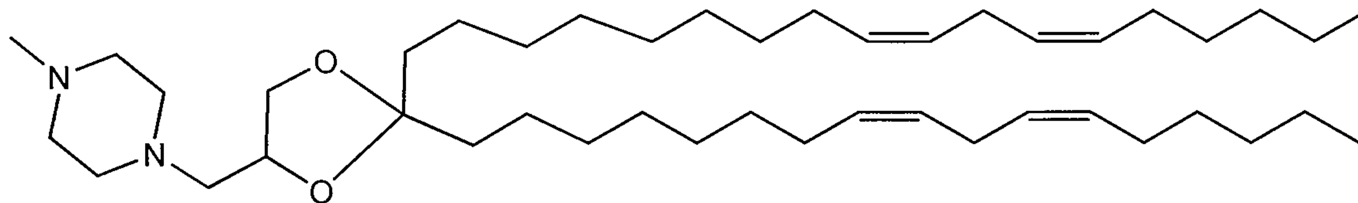
DLin-K-MPZ.
