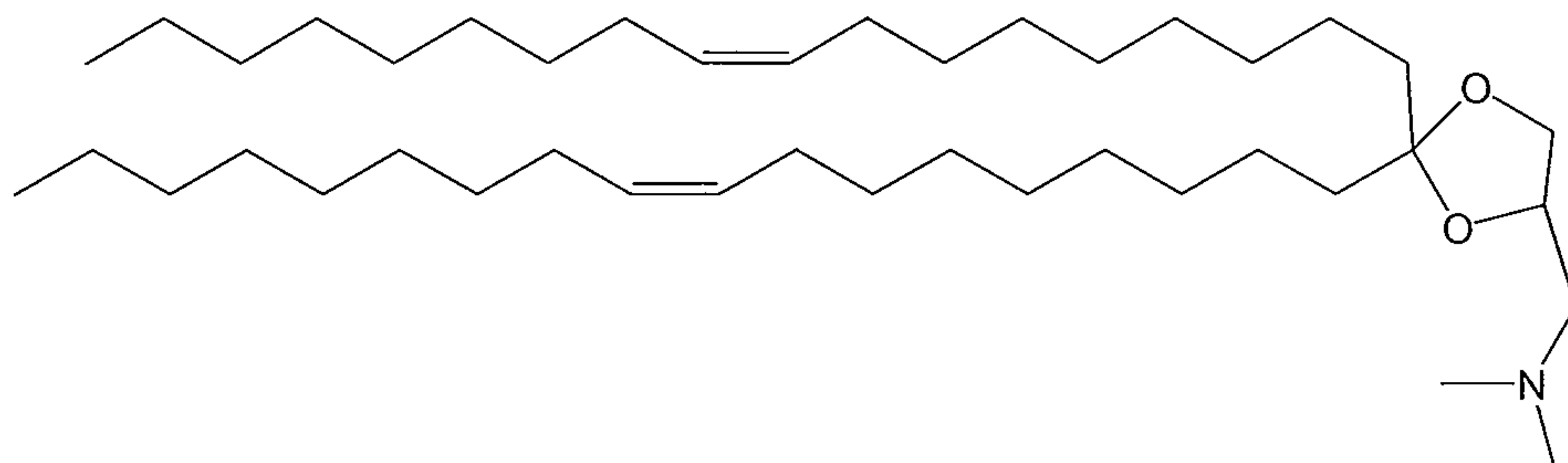
DO-K-DMA;
