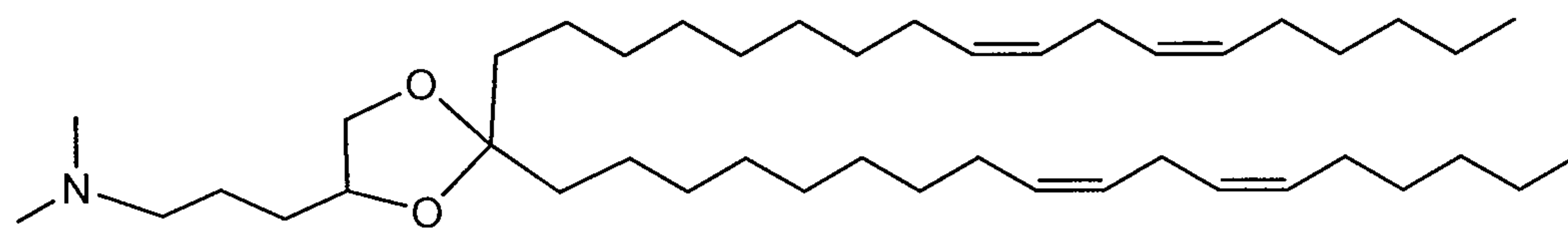
DLin-K-C3-DMA.
