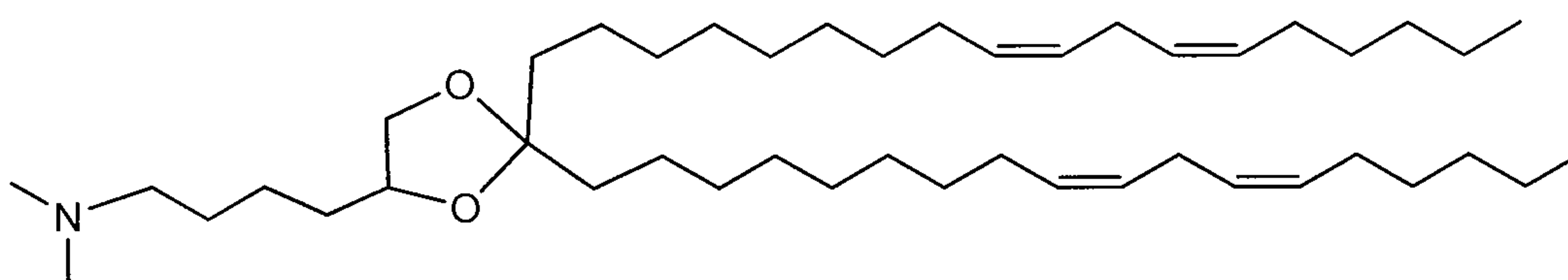
DLin-K-C4-DMA.
