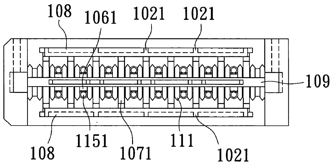
A-A' Fig. 16
