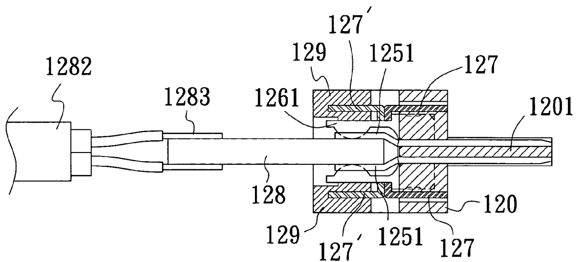
E-E' Fig. 20
