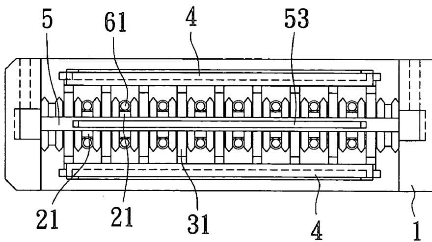
D-D' Fig. 10
