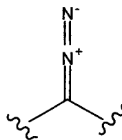
diazo
