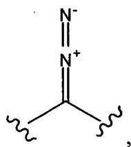
diazo
