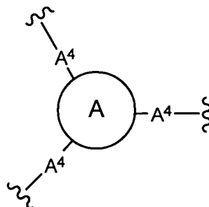
(XIV); or
