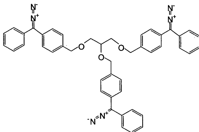
(XXVIIa)
