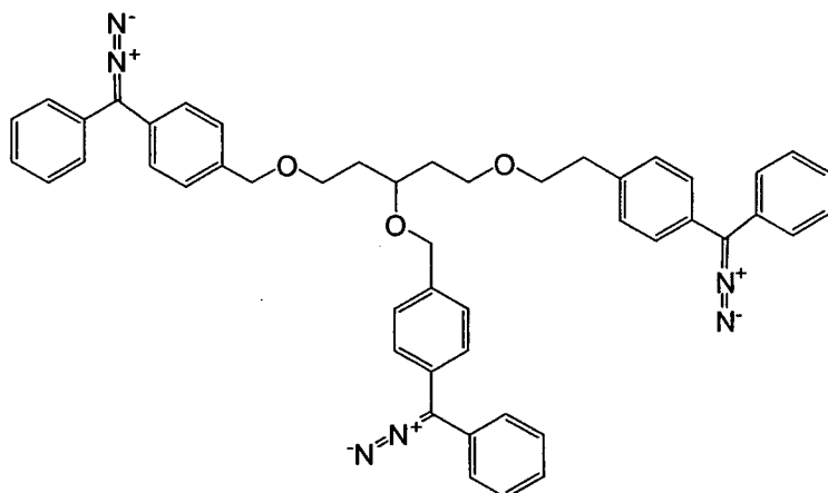
(XXVII)
