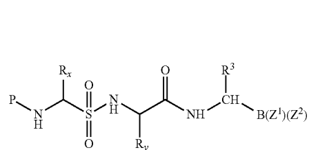
sulfonamide isostere
