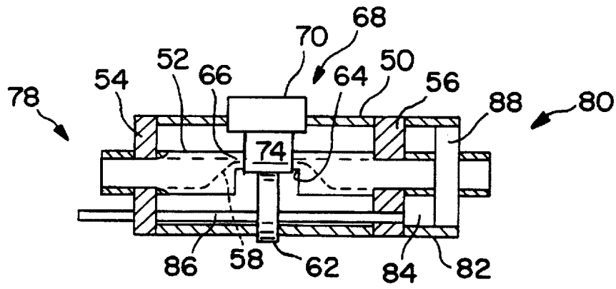
22 FIG. 3
