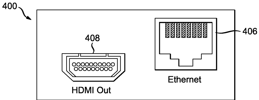
Simple AV Client Only Device Back Panel
