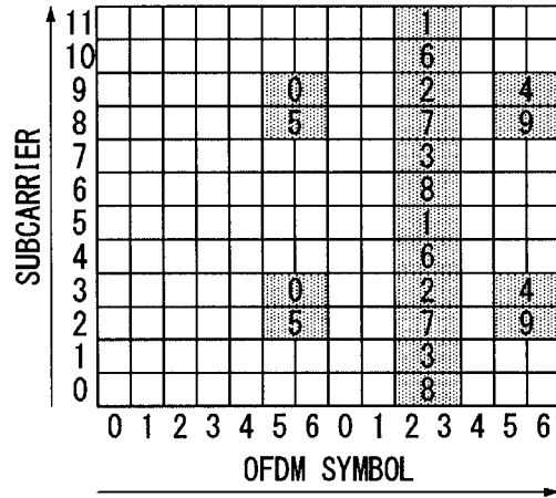
(b) 4 CSI-RS PORTS
