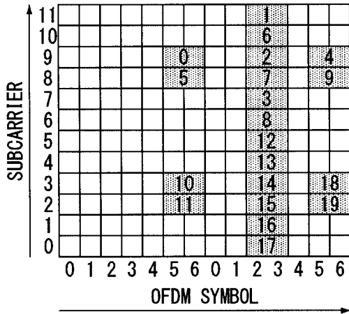
(a) 1 OR 2 CSI-RS PORT
