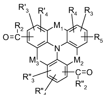
(Ib)
