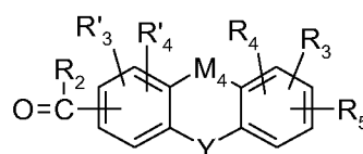
(IIb), wherein
