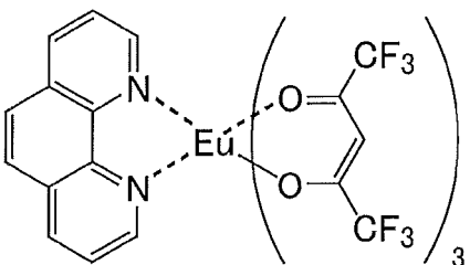
Eu(HFA) 3 phen
