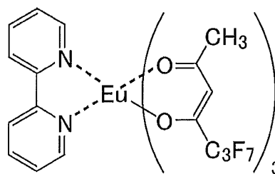
[Eu(FPD) 3 ]bpy
