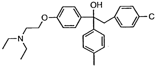
TRIPARANOL
