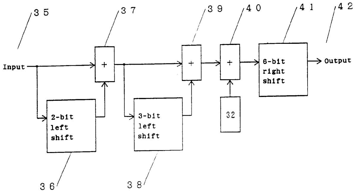
Fig. 10 Divider 33
