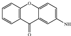
2-amino-xanthone (2AX)
