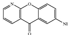
7AAX
