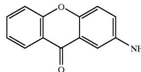
2AX
