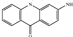
3-amino-acridone (3AAC)
