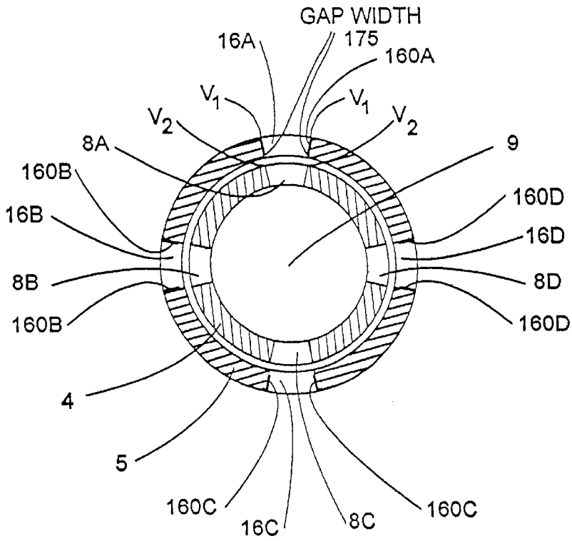
FIG. 2E
