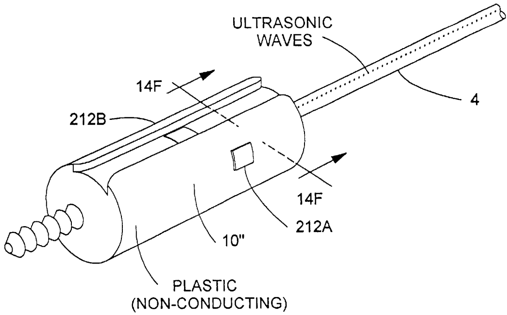
FIG. 14E
