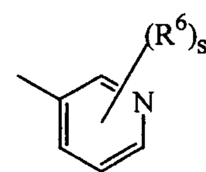
(a-4)
