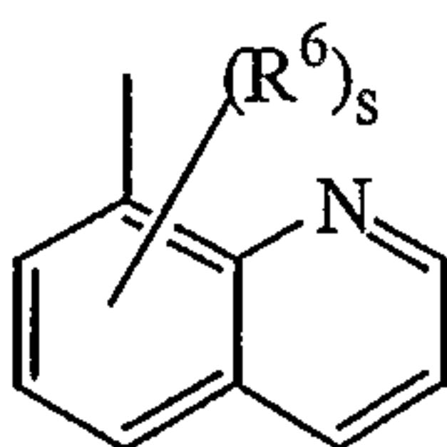
(a-22)
