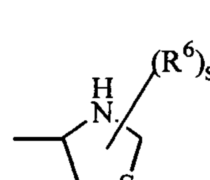
(a-16)
