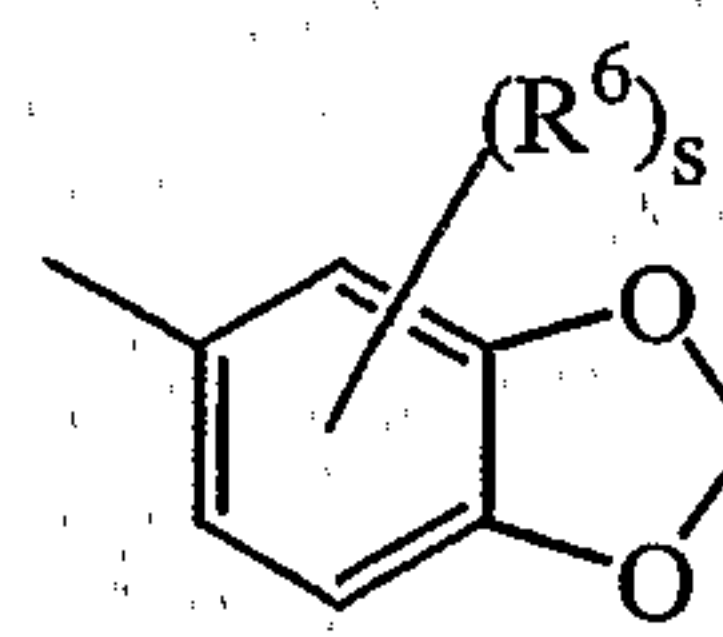
(a-32)
