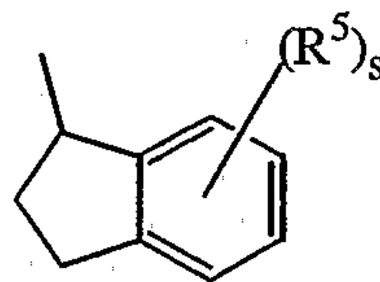
(a-27)
