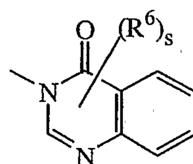
(a-47)
