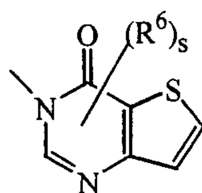
(a-46)
