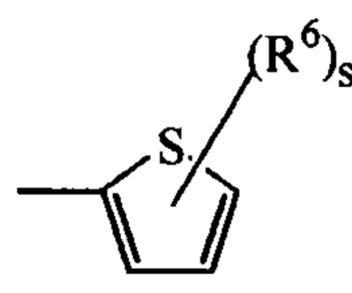
(a-9)
