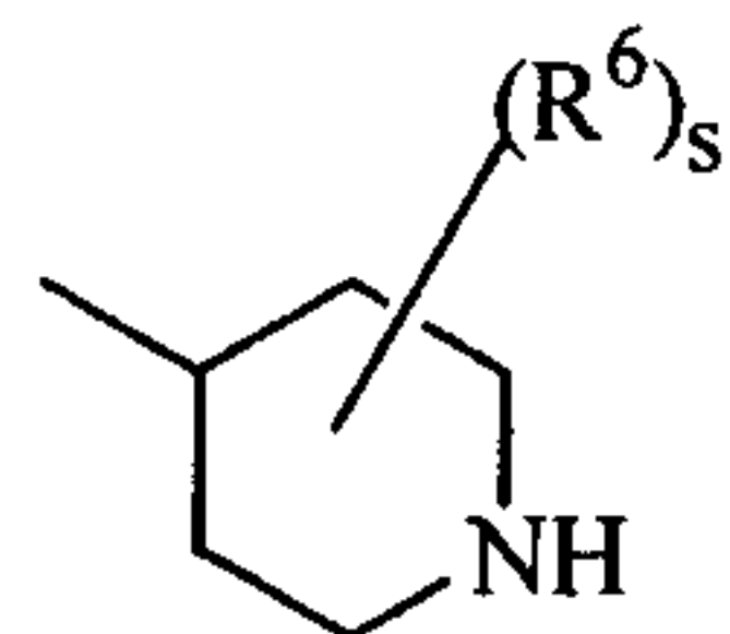
(a-6)
