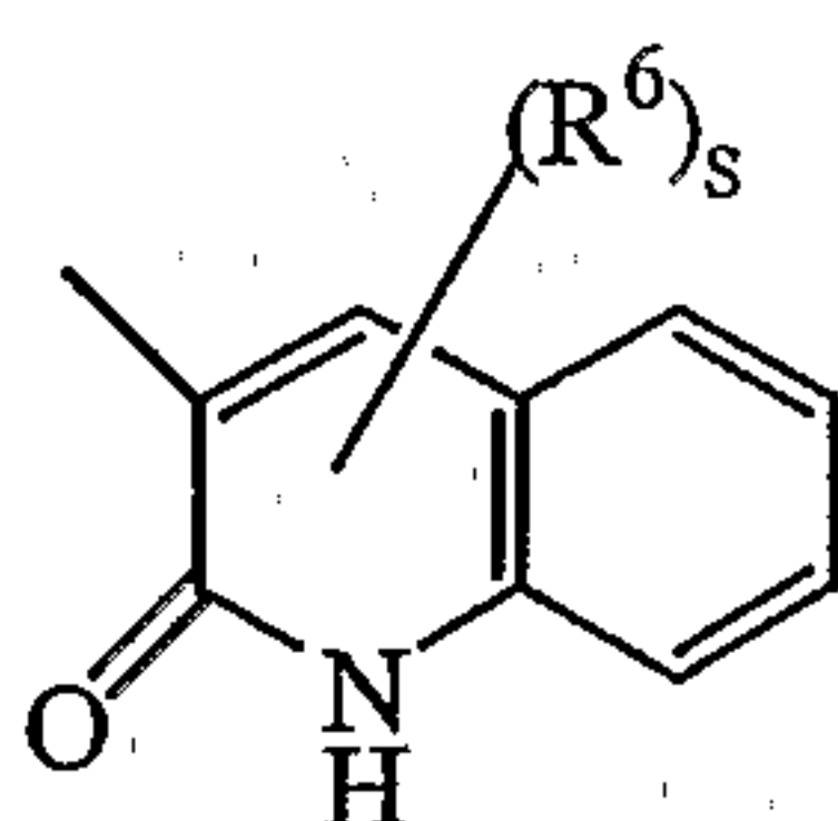
(a-26)
