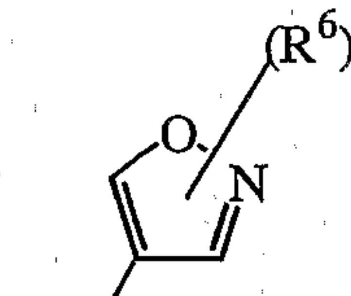
(a-12)
