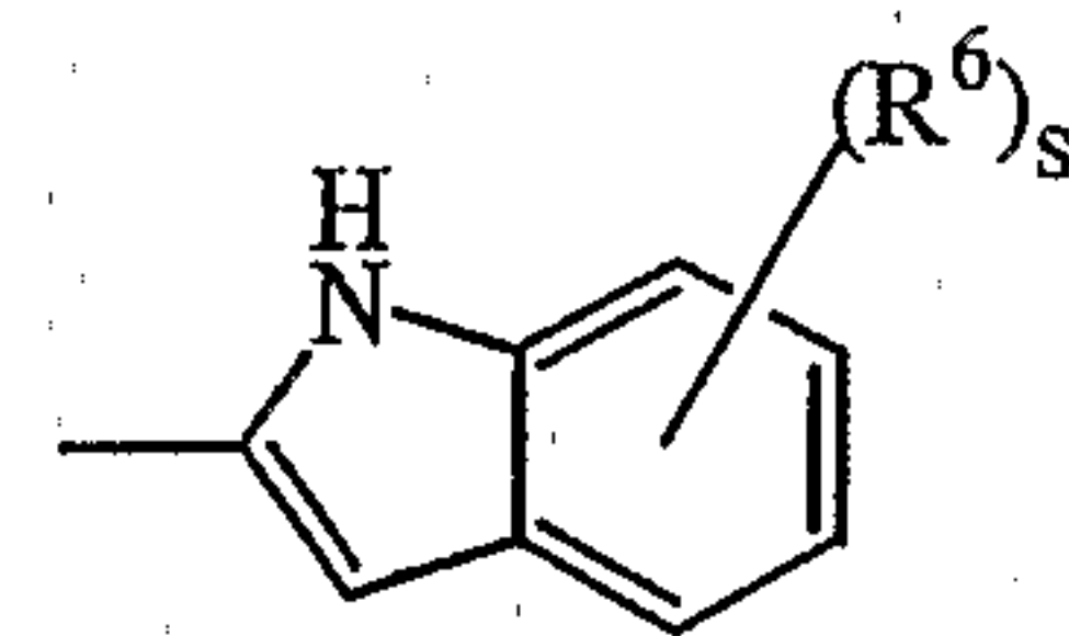
(a-28)
