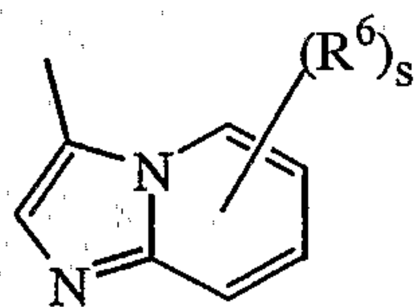
(a-33)
