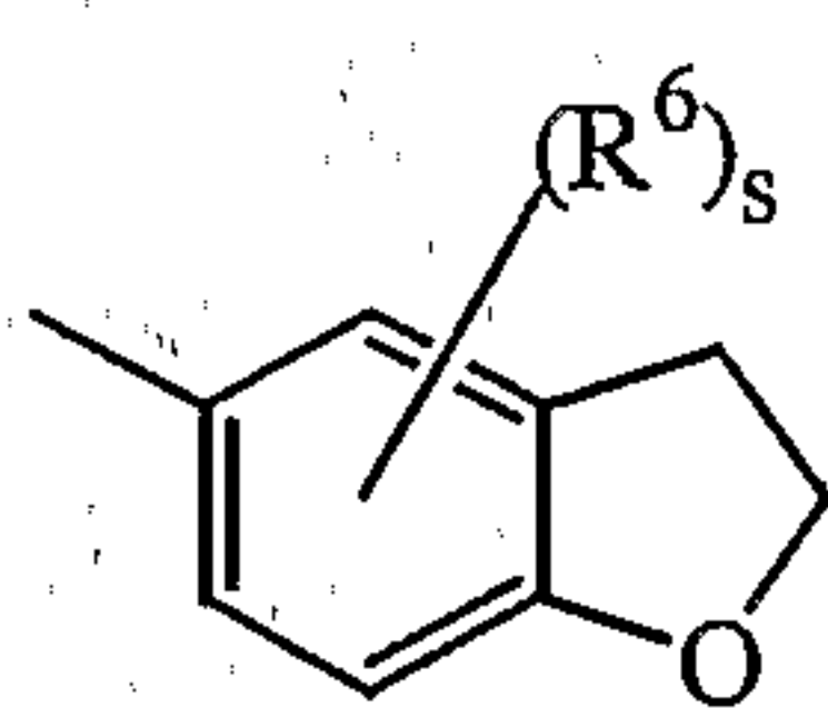
(a-30)
