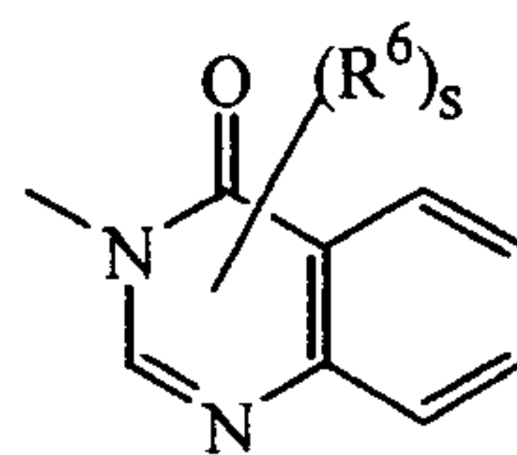
(a-47)
