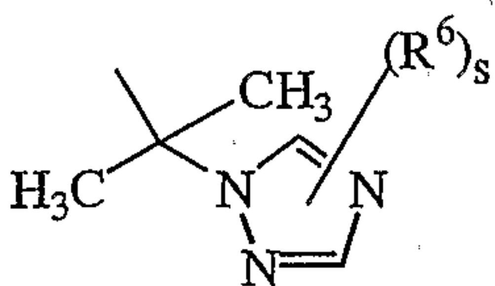
(a-17)
