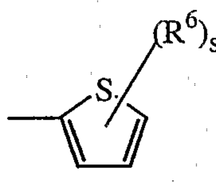
(a-9)
