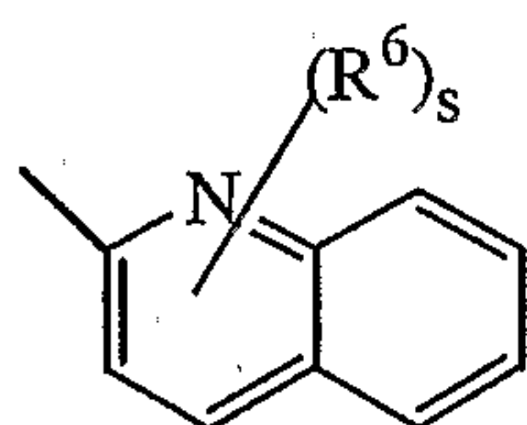
(a-41)
