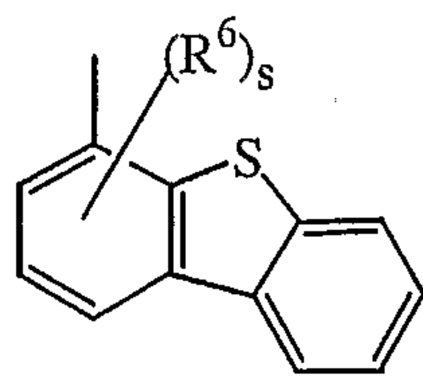
(a-49)
