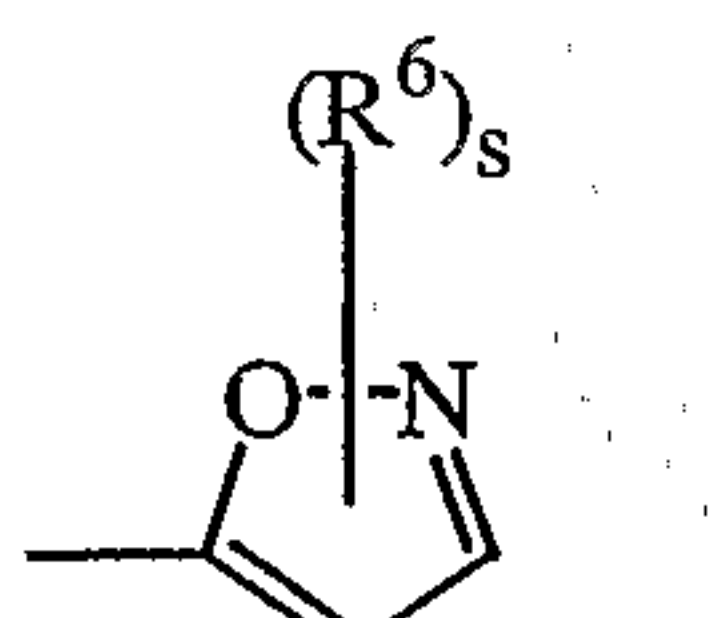
(a-13)
