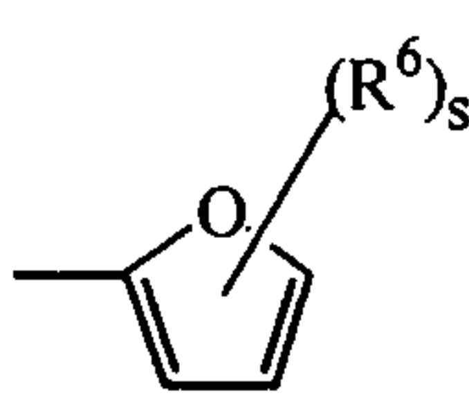
(a-11)
