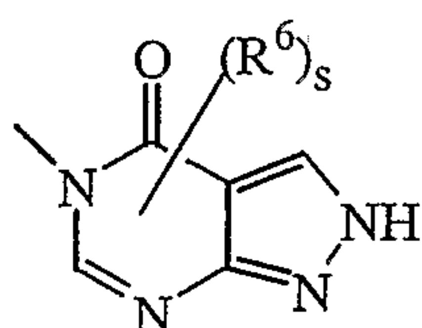
(a-45)
