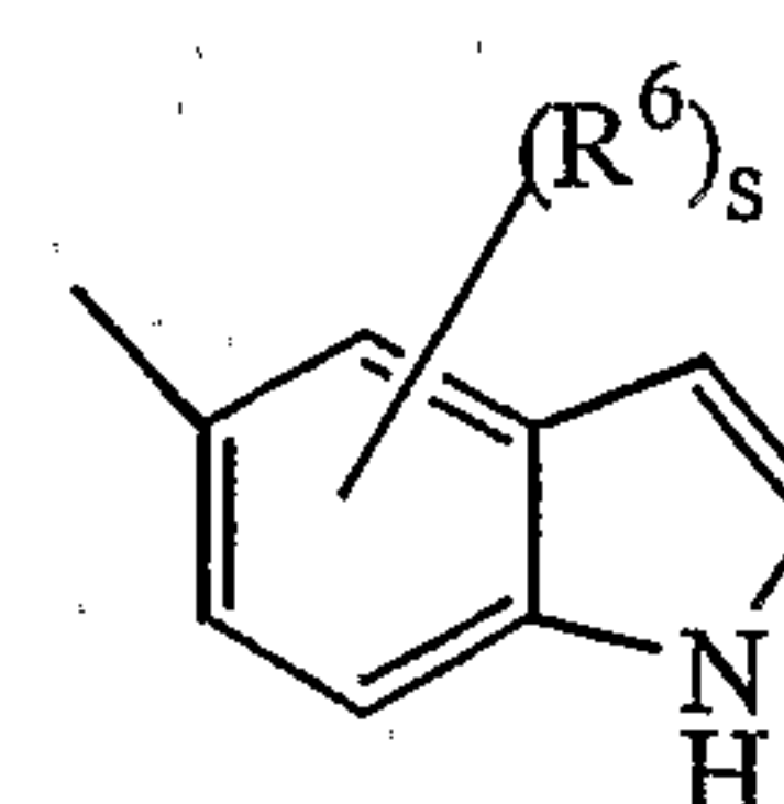
(a-48)
