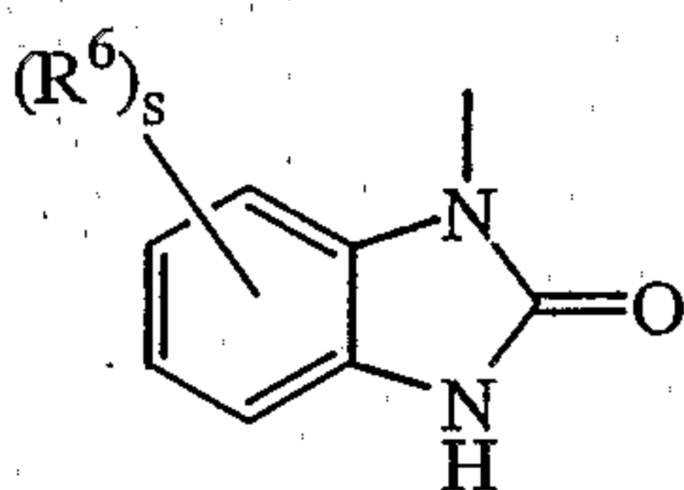
(a-33)
