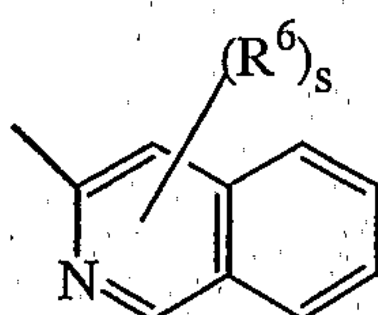
(a-42)
