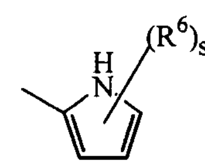
(a-8)
