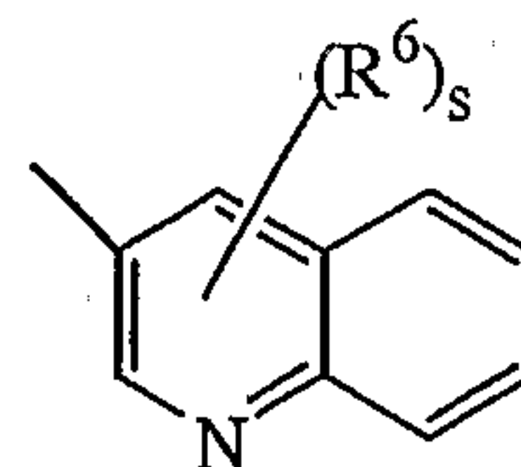
(a-24)
