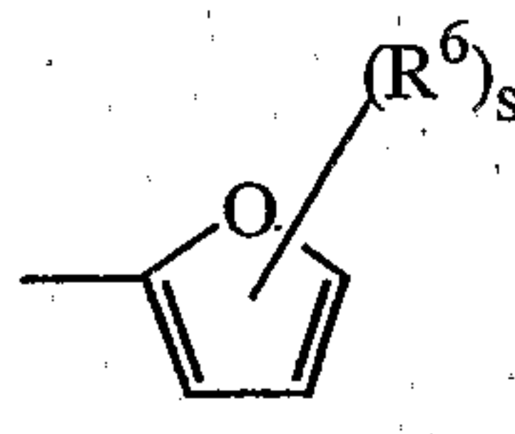
(a-11)
