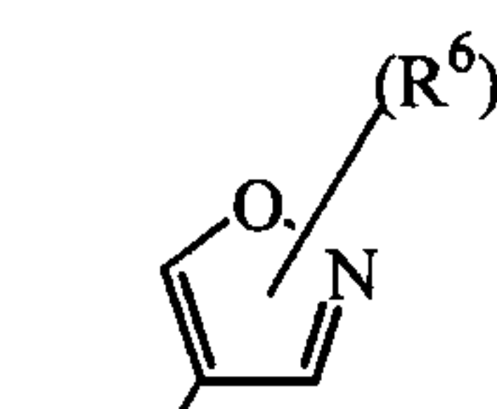
(a-12)
