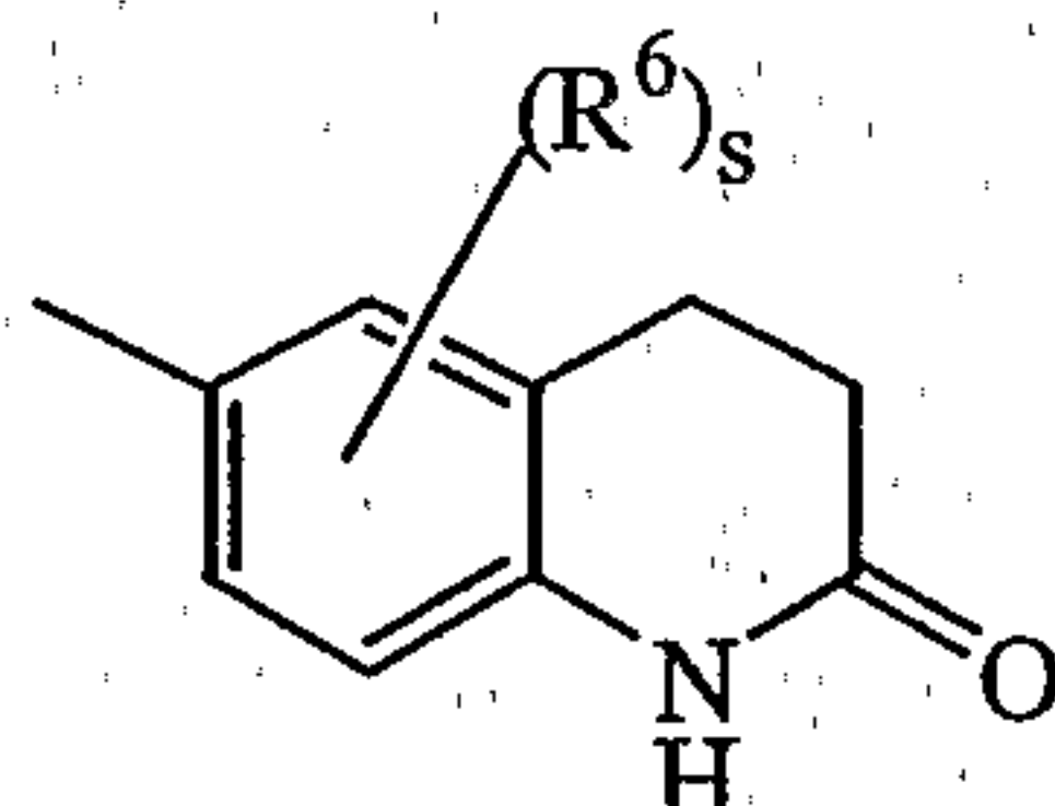
(a-38)
