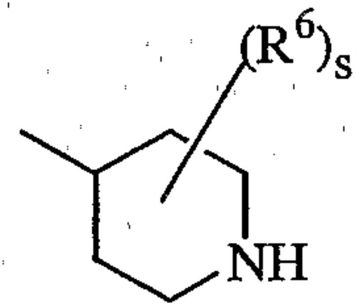
(a-6)
