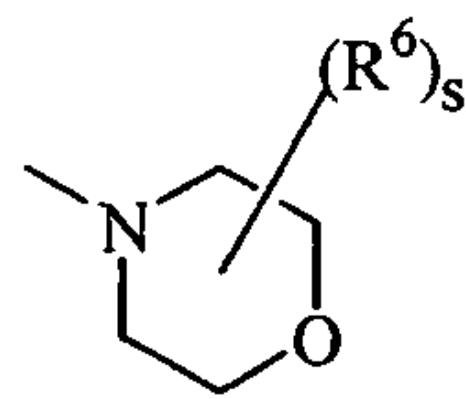
(a-7)
