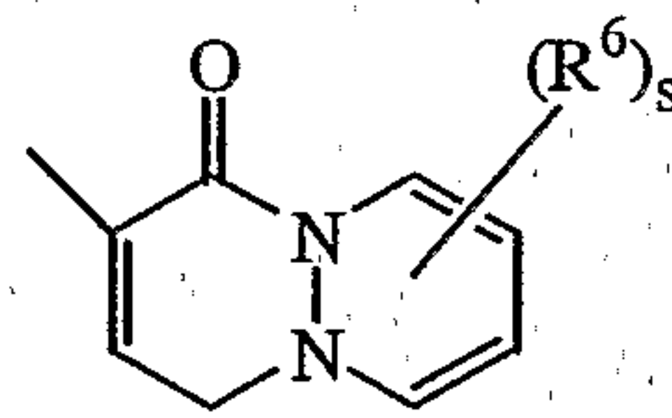
(a-35)
