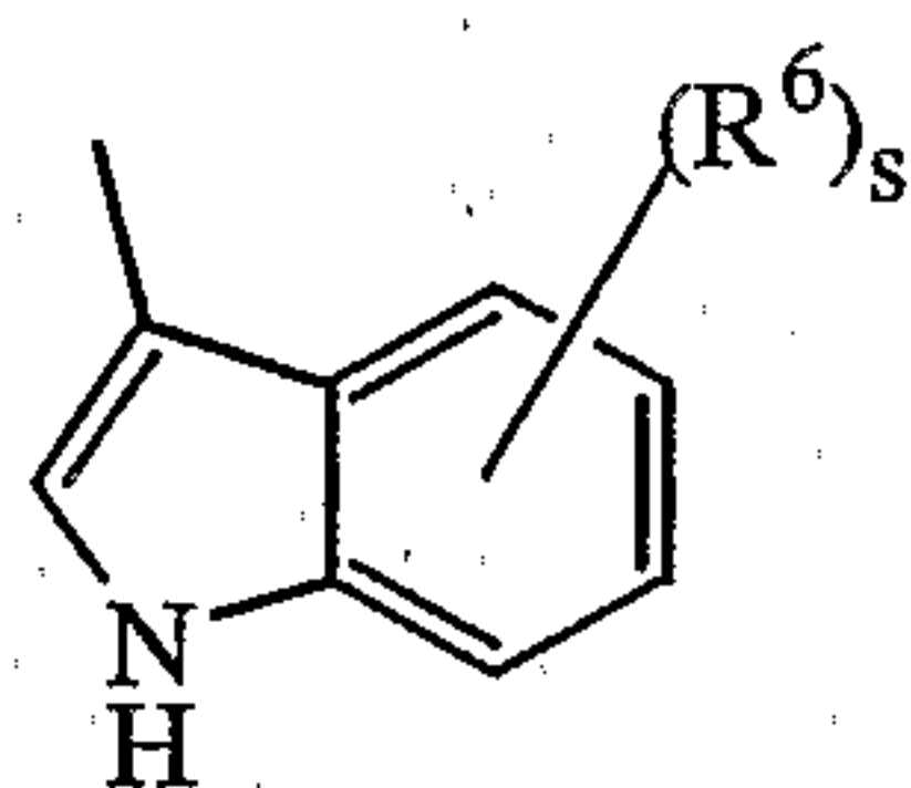
(a-29)
