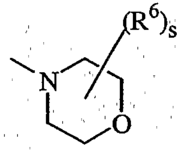
(a-7)
