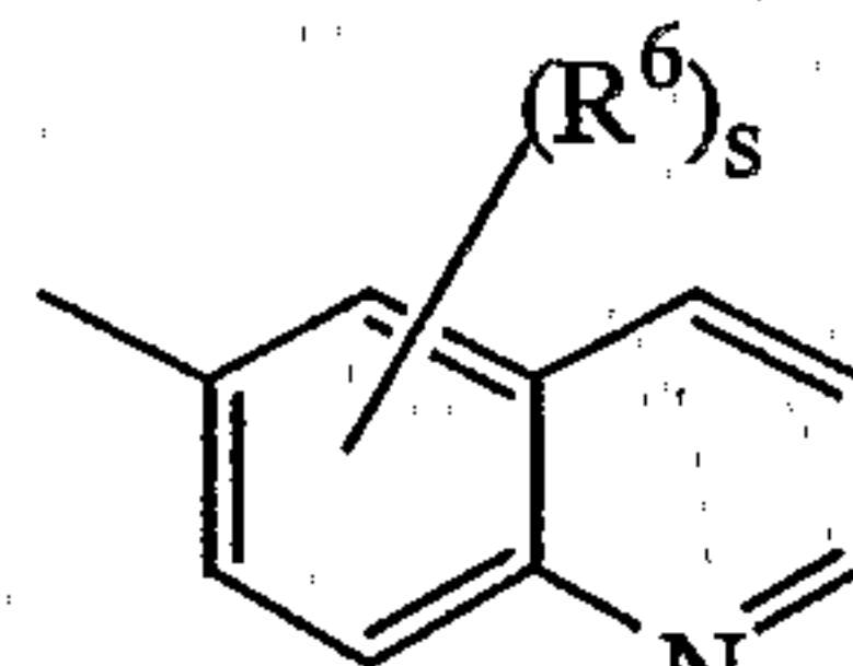
(a-39)
