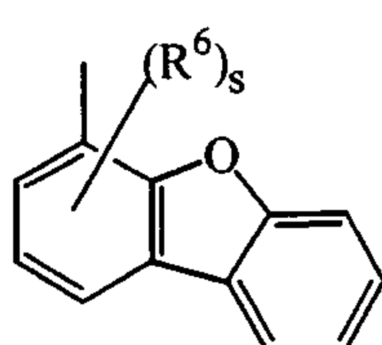
(a-50)
