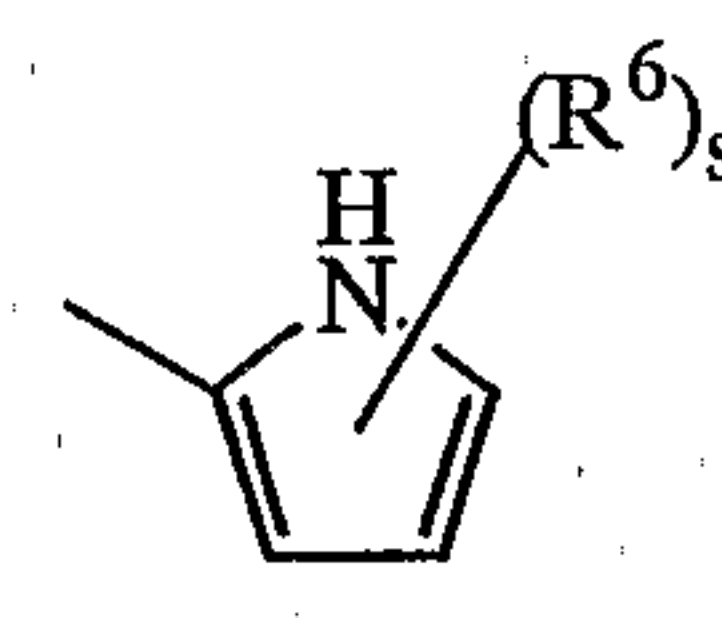
(a-8)
