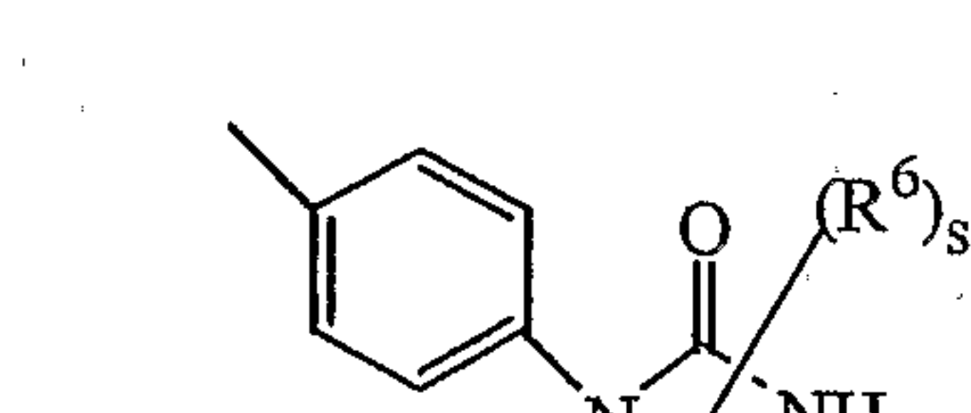
(a-18)
