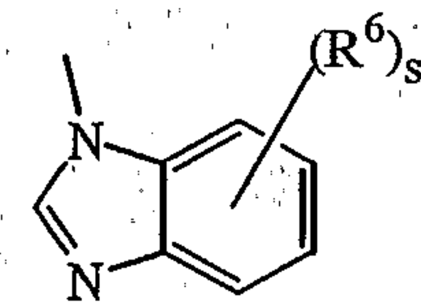
(a-36)
