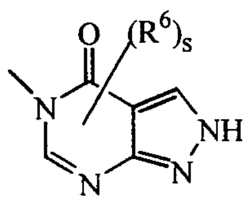
(a-45)
