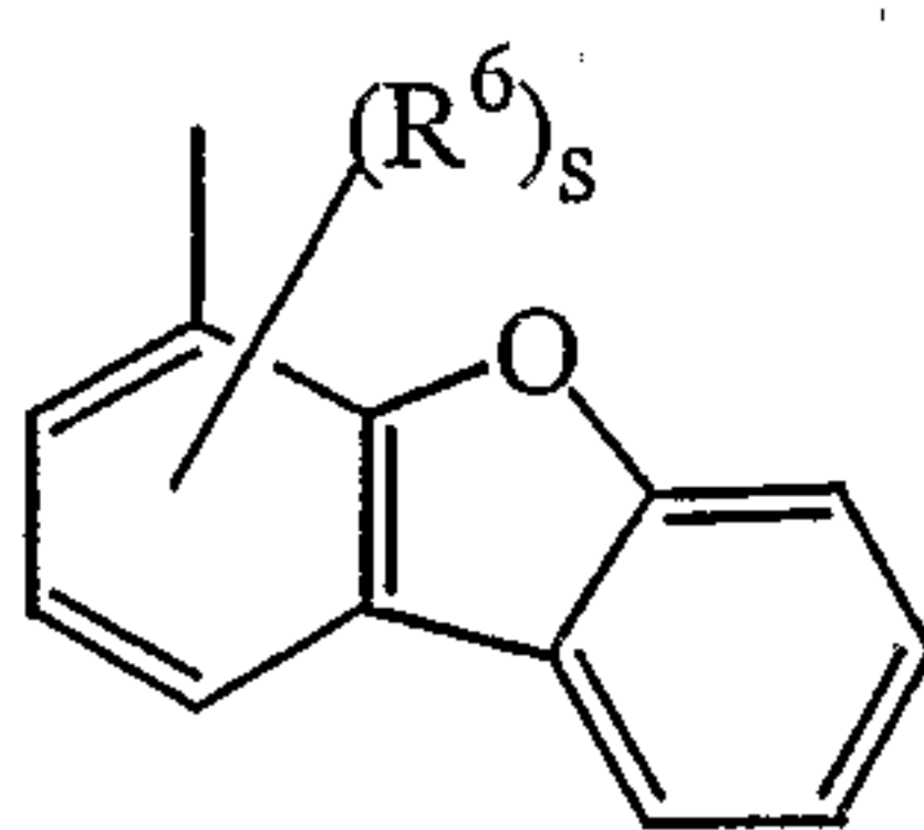
(a-50)
