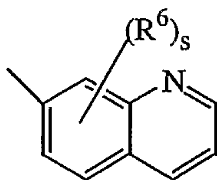
(a-23)
