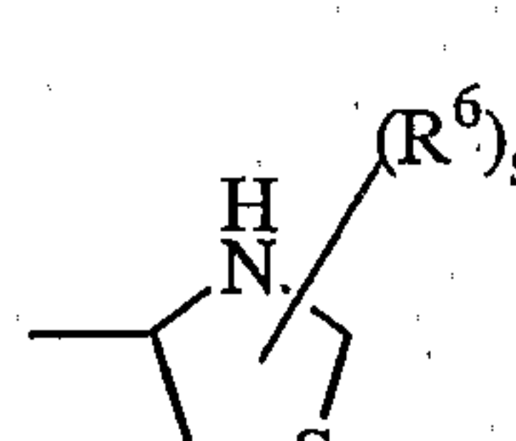
(a-16)
