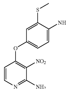
4-(4-amino-3-(methylthio)phenoxy)-3-nitropyridin-2-amine
