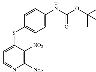
tert-butyl 4-(2-amino-3-nitropyridin-4-ylthio)phenylcarbamate
