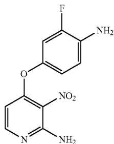
4-(4-Amino-3-fluorophenoxy)-3-nitropyridin-2-amine
