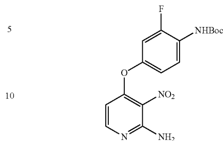
4-(4-N-tert-Butoxycarbonyl)amino-3-fluorophenoxy)-3-nitro-2-amino-pyridine
