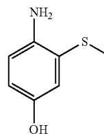
4-amino-3-(methylthio)phenol
