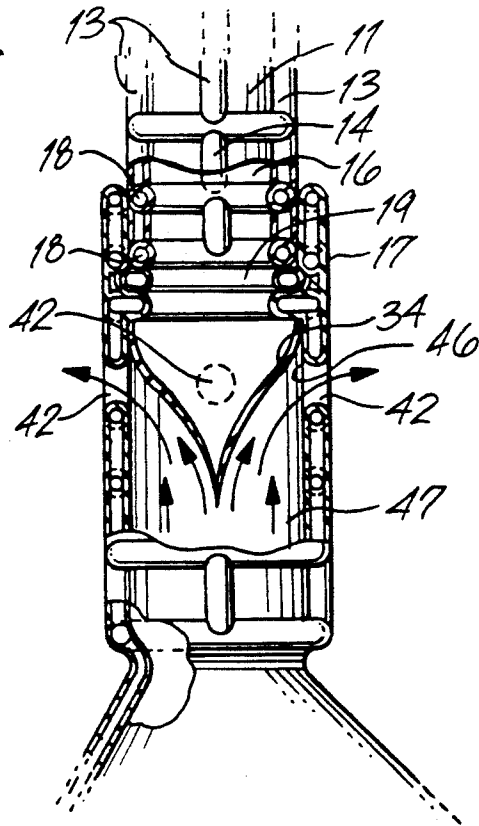
Fig. 8B
