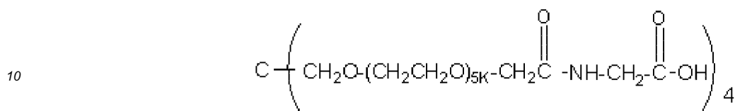
4-ARM-PEG 20K -CM-Glycine
