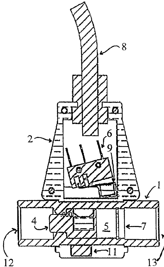
SECTION D-D
