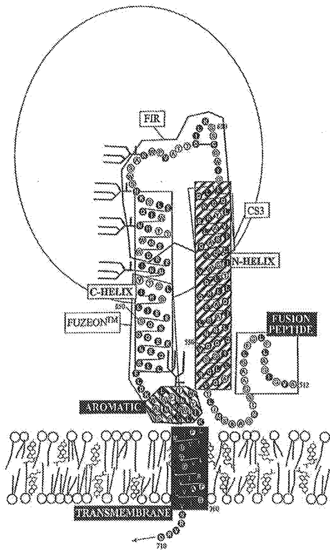
HIV-1 TM Figure 7
