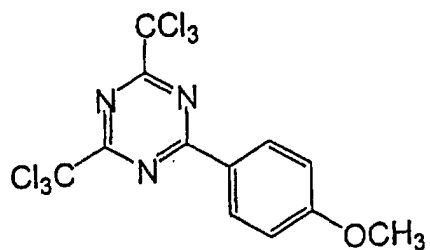
Initiator A
