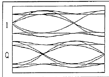
FQPSK-B MEAS.
