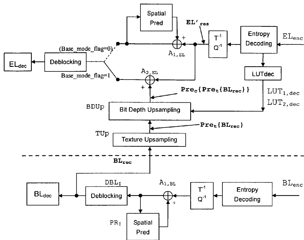
Fig. 3 (Intra-Decoder)
