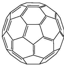
C60
