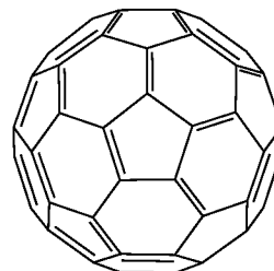
C70
