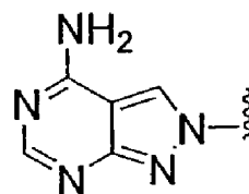
N8-(7-deaza-8-aza-A)
