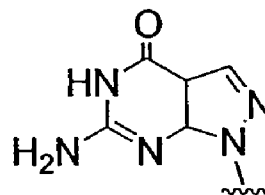
N9-(7-deaza-8-aza-G)
