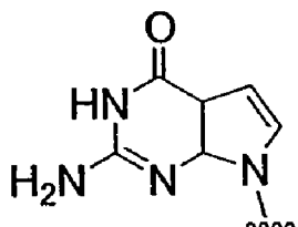
N9-(7-deaza-G)
