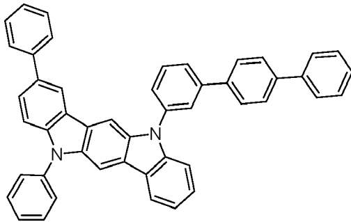
Cmpd 94
