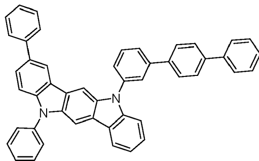
Cmpd 94
