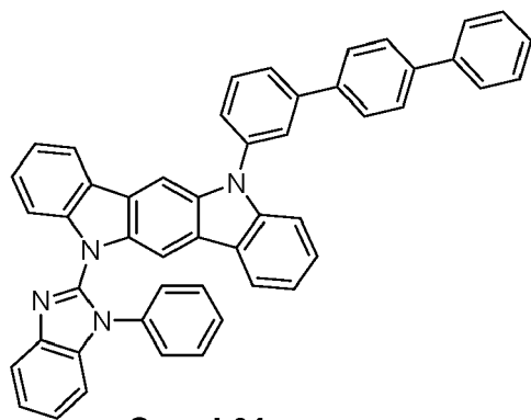
Compd 61
