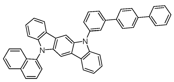
Cmpd 12
