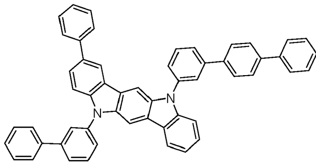
Cmpd 98
