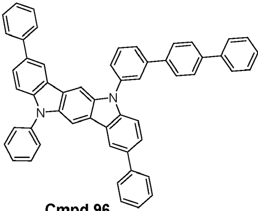
Cmpd 96
