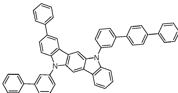
Cmpd 98
