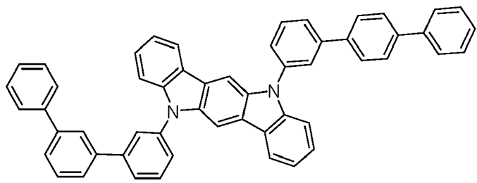
Cmpd 8
