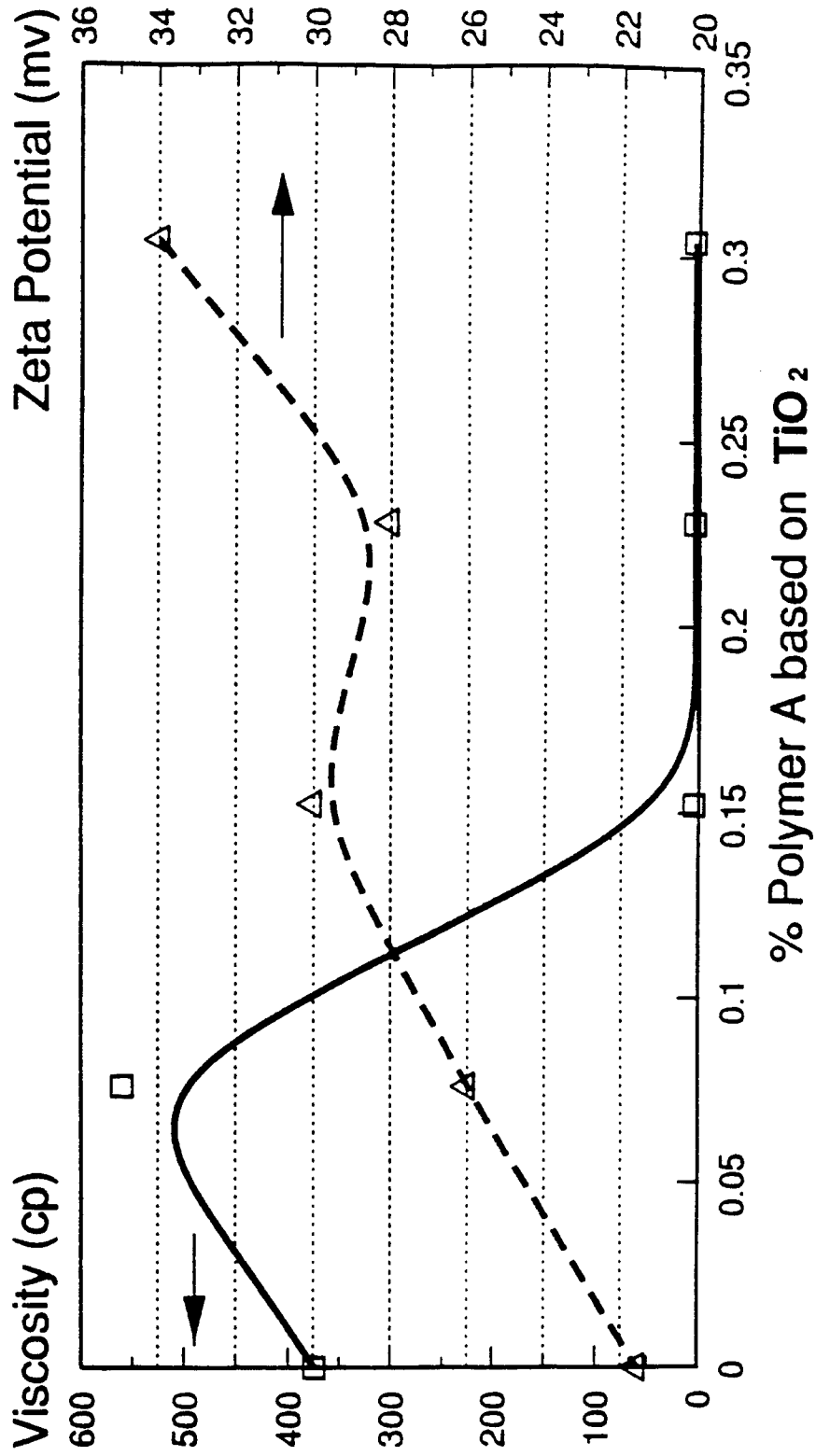
FIGURE 2 Rutile TiO 2 Breakover
